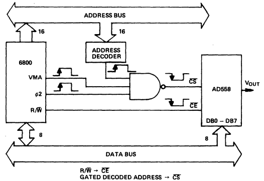
a. 6800/AD558 Interface
