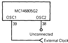
(d) External Clock Source Connections
