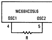
(d) RC OSCILLATOR CONNECTIONS
