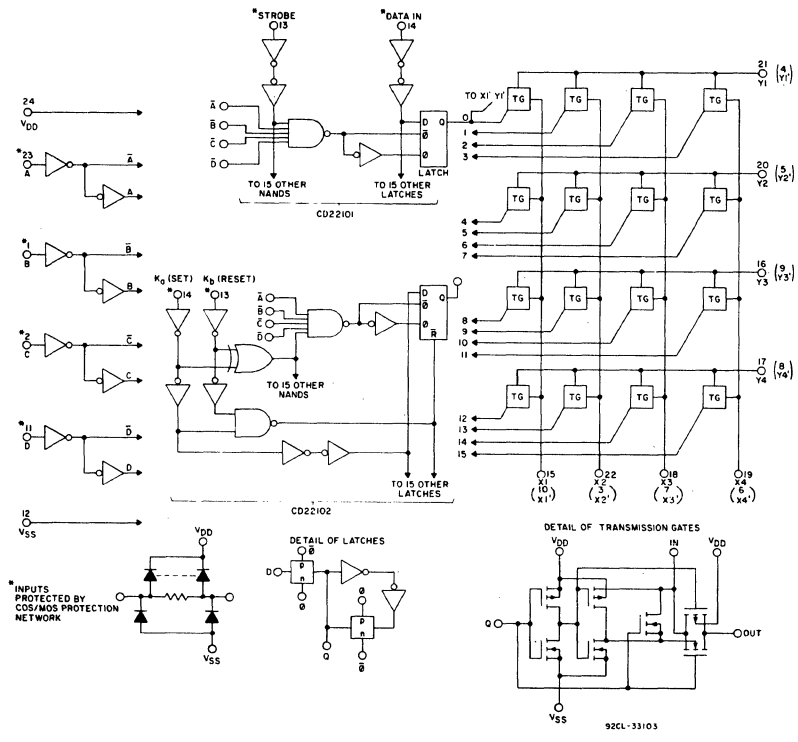
Fig. 2 - Logic diagram.
