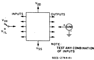
Fig. 16 - Input-voltage test circuit.
