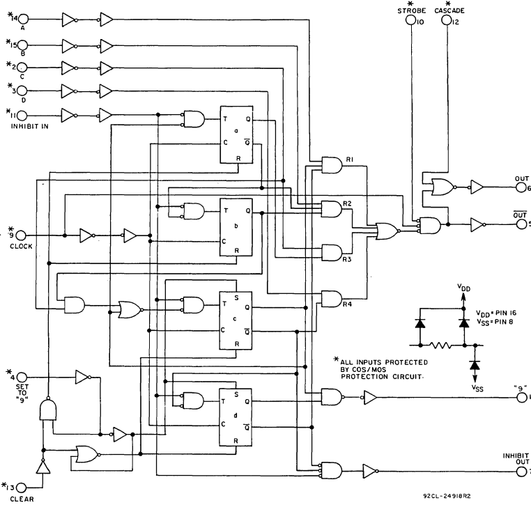
Fig. 13 - Logic diagram.
