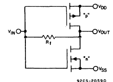
Fig. 5— COS/MOS amplifier.
