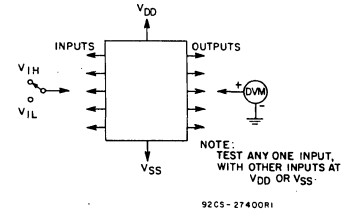
Fig. 15 - Input voltage.
