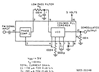
Fig. 10— FM demodulator.
