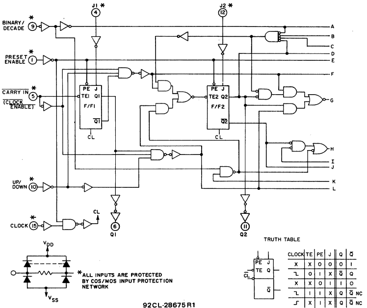
Fig. 9 - Logic diagram.
