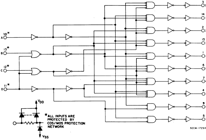
Fig. 4 - Logic diagram.
