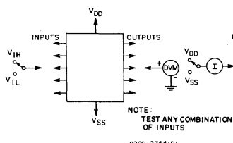
Fig. 15 - Input voltage test circuit.
