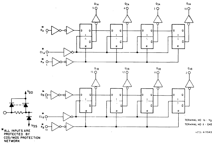
Fig. 6 - Logic diagram.
