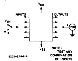
Fig. 17 - Input-voltage test circuit.
