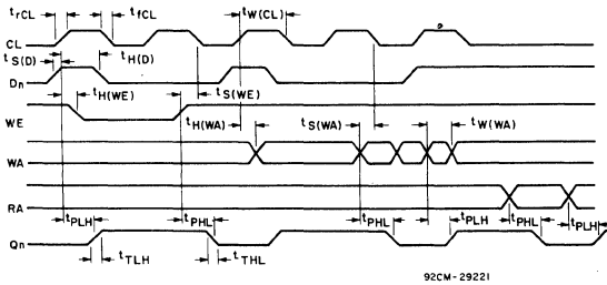
Fig. 4— Timing diagram.
