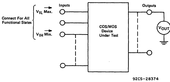
Fig. 19 - Input-voltage-level test arrangement.
