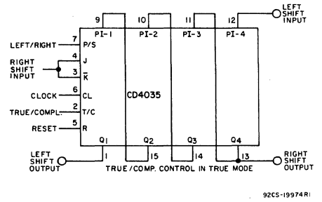
Fig. 14 - Shift left/shift right register.
