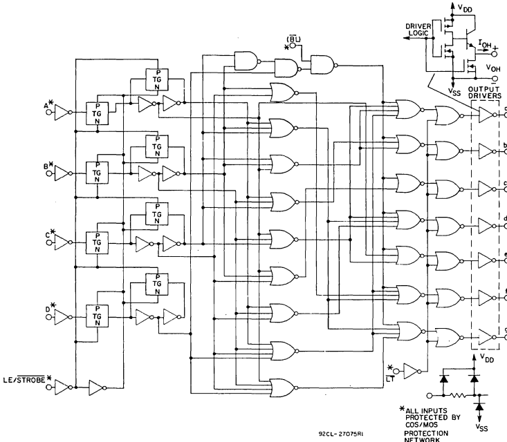
Fig. 8 - Logic diagram.
