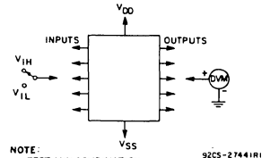
Fig. 13 - Input-voltage test circuit.
