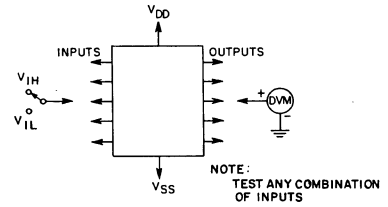
Fig. 16 - Input voltage.
