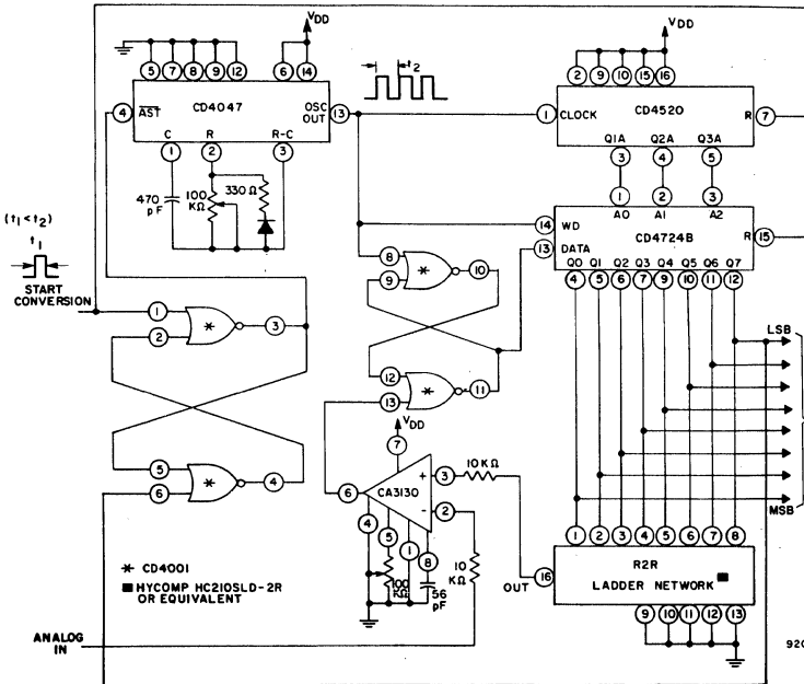
Fig. 5— A/D converter
