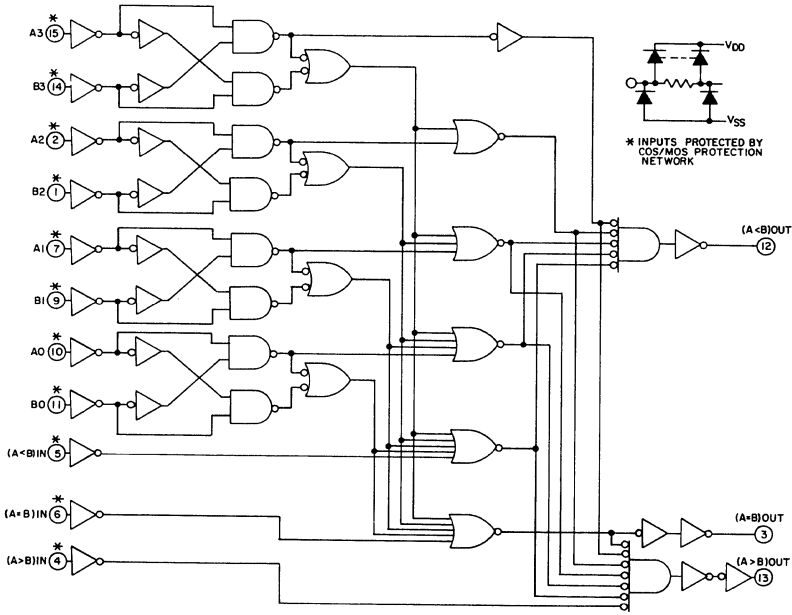
Fig. 4 - Logic diagram.
