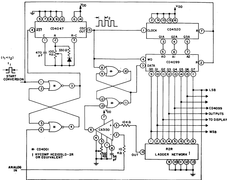
Fig. 5 - A/D converter
