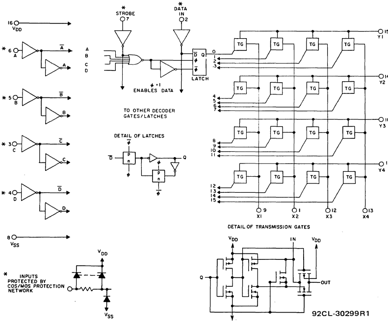
Fig. 6— Schematic diagram.
