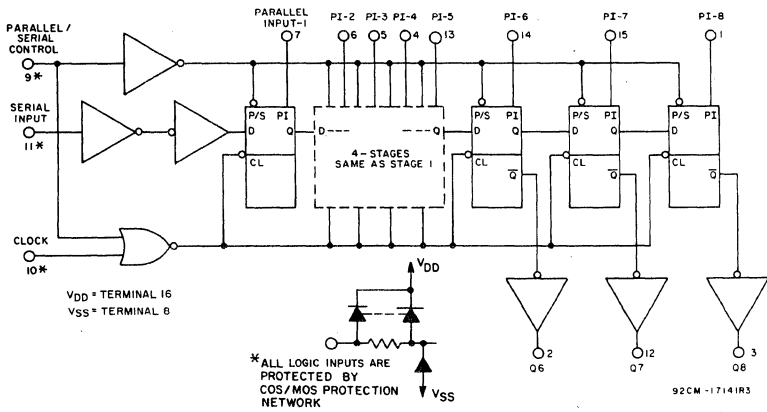
Fig. 5 - Logic diagram.
