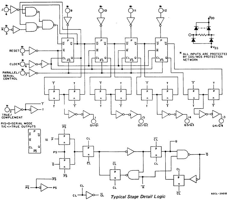
Fig. 4 - Logic diagram.
