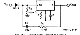
Fig. 22 - Input-pulse stretcher circuit.
