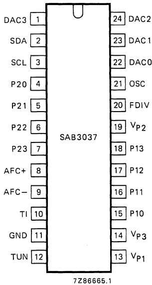
Fig. 2 Pinning diagram.
