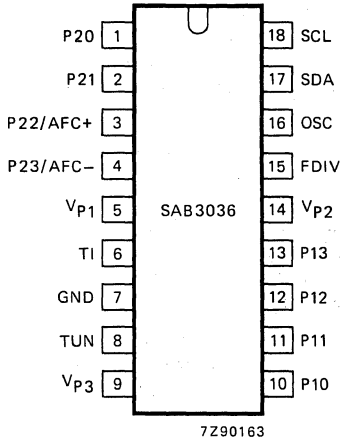
Fig. 2 Pinning diagram.
