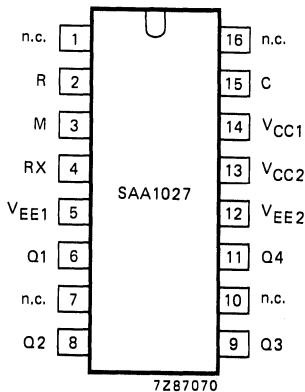
Fig. 2 Pinning diagram.
