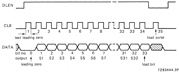
Fig. 3 Data format.
