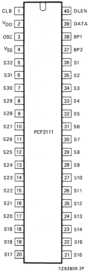
Fig. 11 Pinning diagram.
