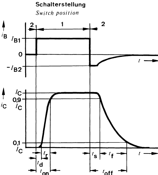
Fig. 1.23. den zeitlichen Verlauf der Steuergröße (des Basisstromes i_B ) und Fig. 1.24. den zeitlichen Verlauf des Kollektorstromes i_C beim Verändern der Schalterstellung.
