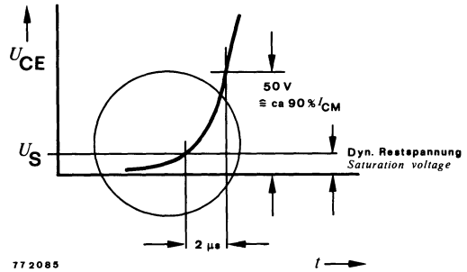
Fig. 1 Definition von U_{Rest\ dyn} Definition from U_{Rest\ dyn}
