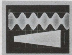
150 MHz AM
