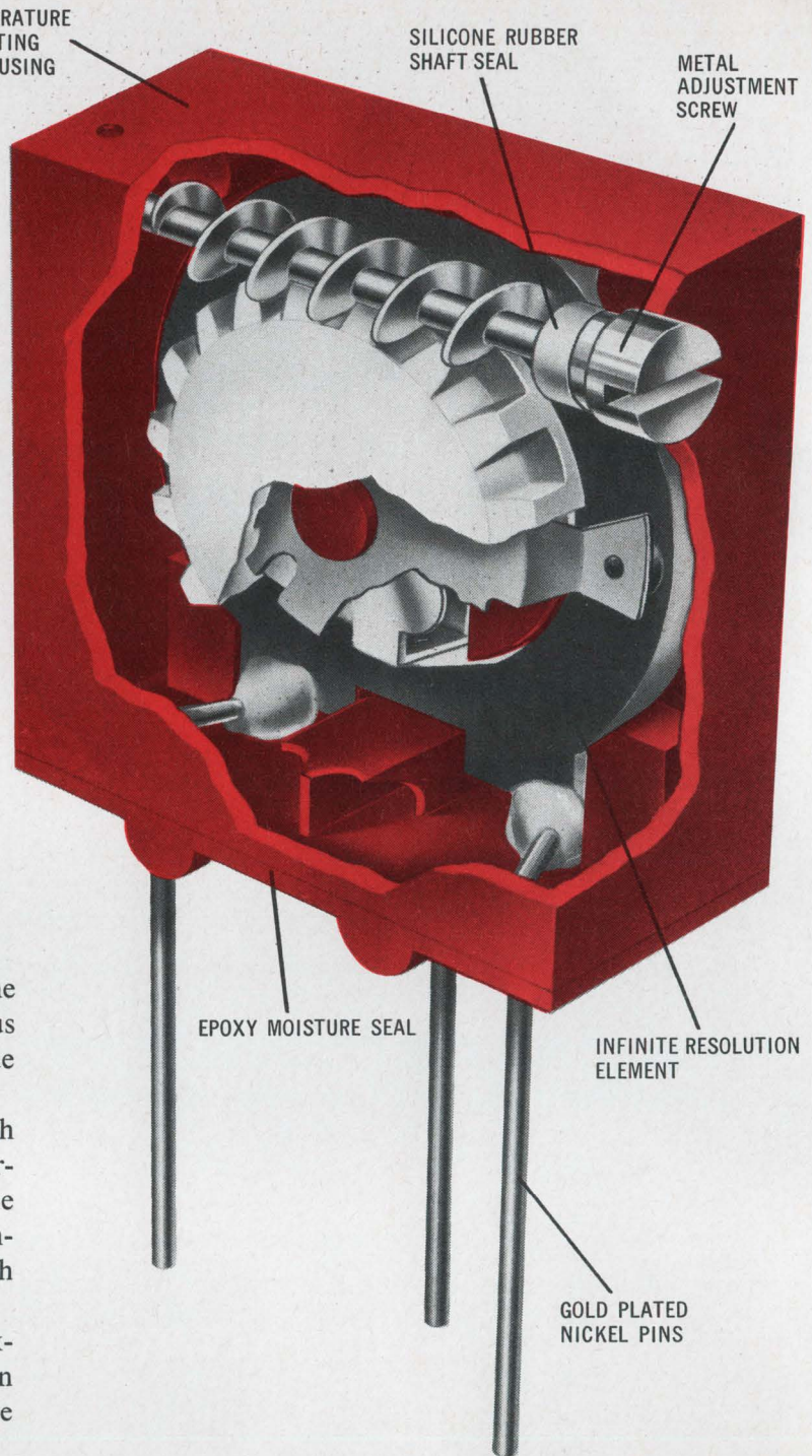
Actual size Infinite Resolution Circuitrim 850
