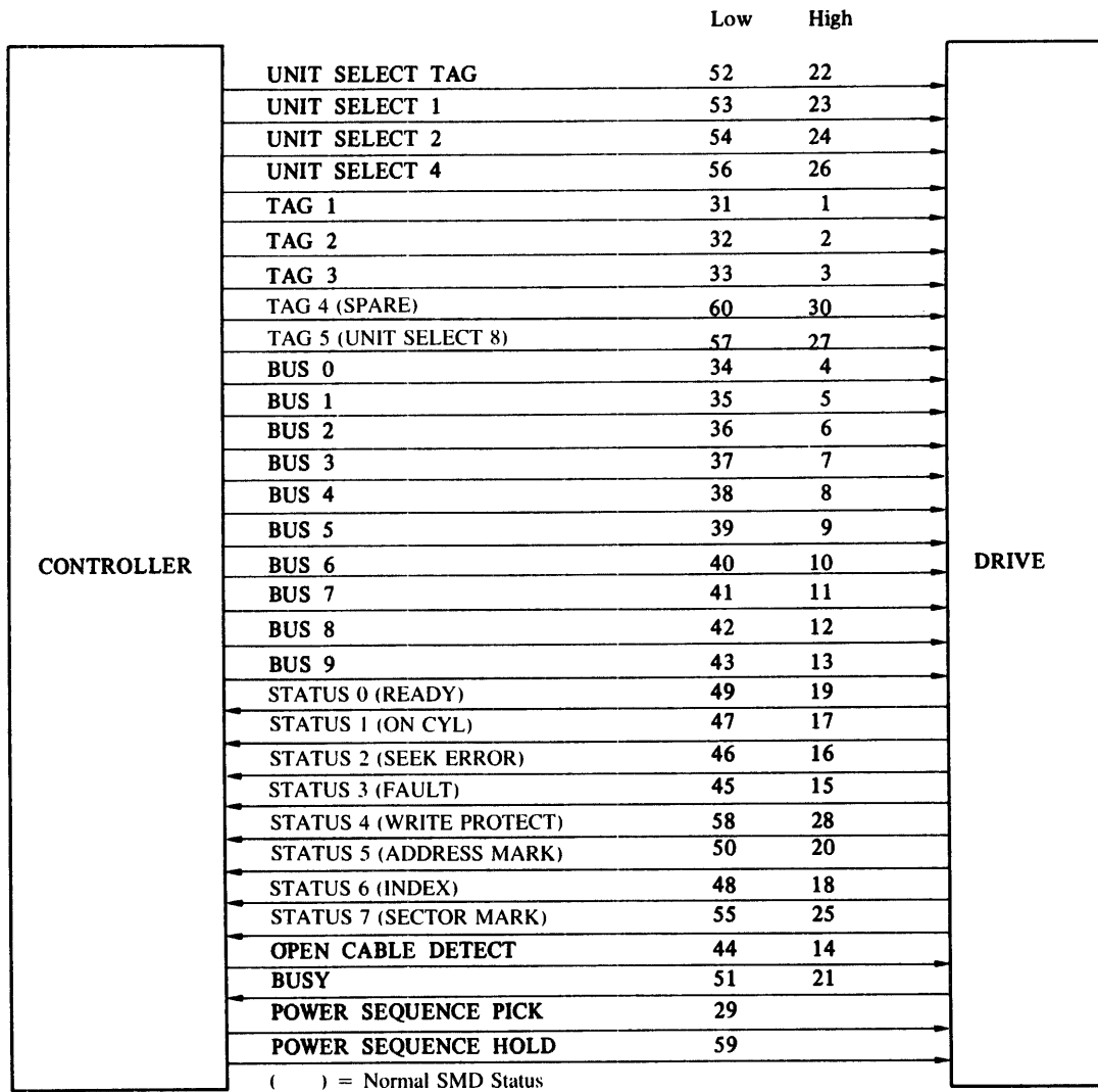
Fig. 7.2-1 A-Cable
