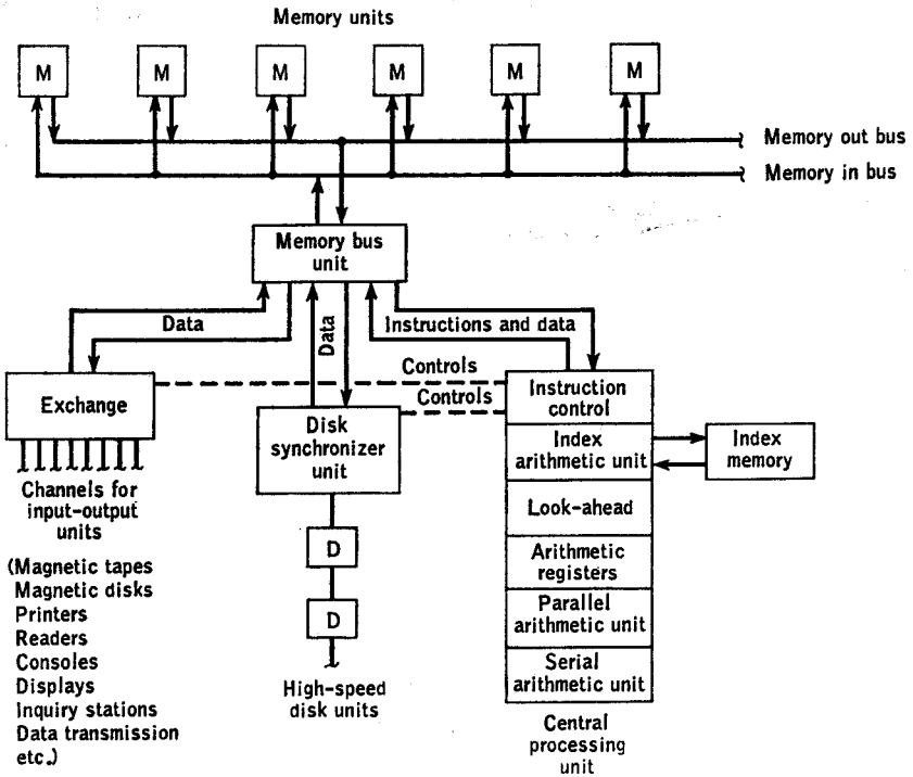
FIG. 3.1. 7030 system.
