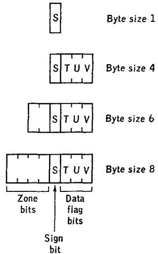
FIG. 7.3. Sign byte.
