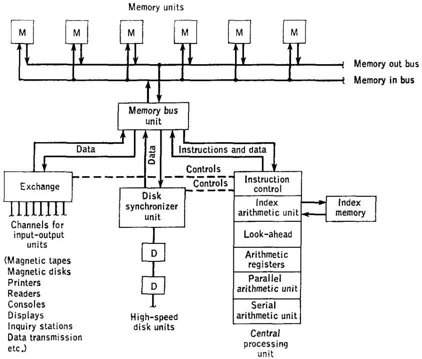
FIG. 14.1. 7030 system.
