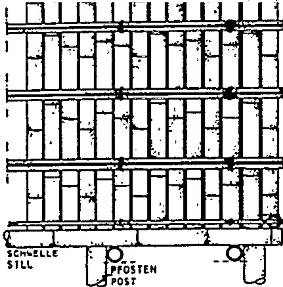
HORIZONTALSCHNITT HORIZONTAL SECTION DRUCKLEISTE HOLDING BATTEN
