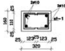
SEC.A-A Set:10
