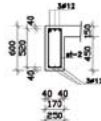
SEC.A-A Set:28
