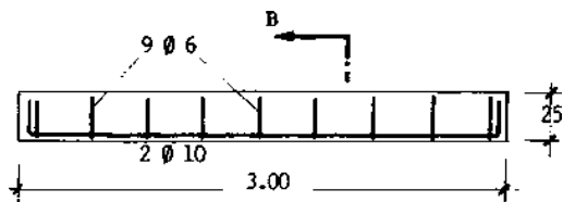
SIDE-VIEW A-A (1:40)
