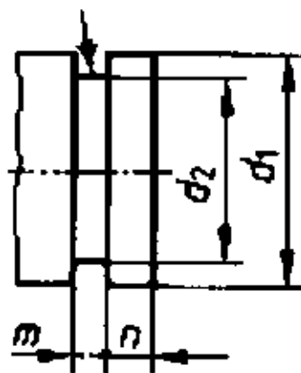
Groove
