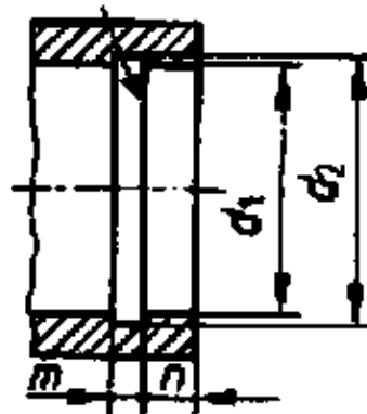
Groove
