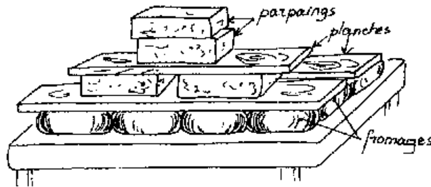
Figure 18 - Le pressage par poids (parpaings)
