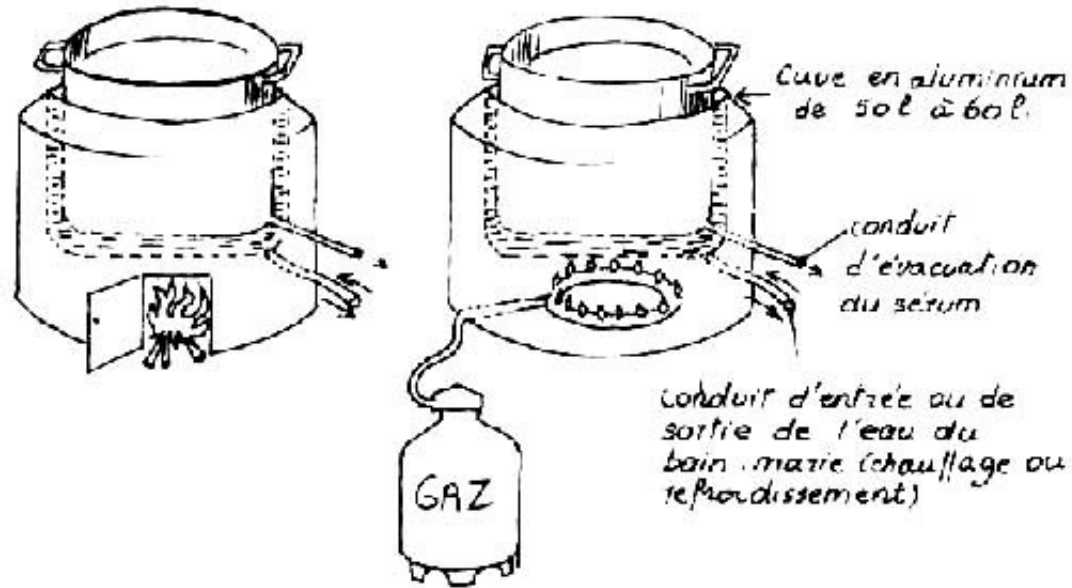
Figure 8 - Chaudière bain-marie améliorées
