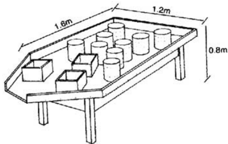
Figure 17 - Table de moulage(en bois ou en acier inoxydable)
