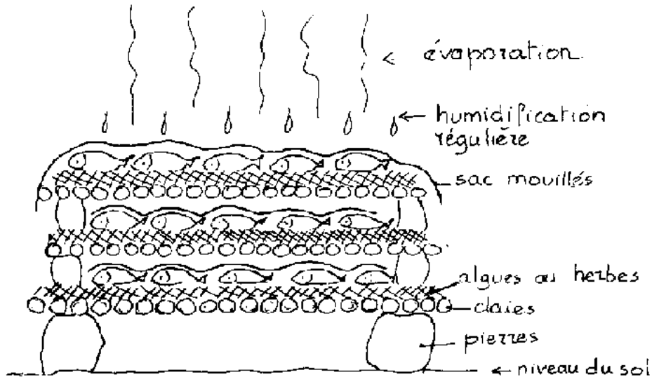
Figure 19: Refroidissement par évaporation
