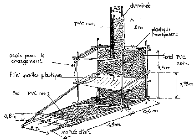
Figure 58: Séchoir solaire de bambou
