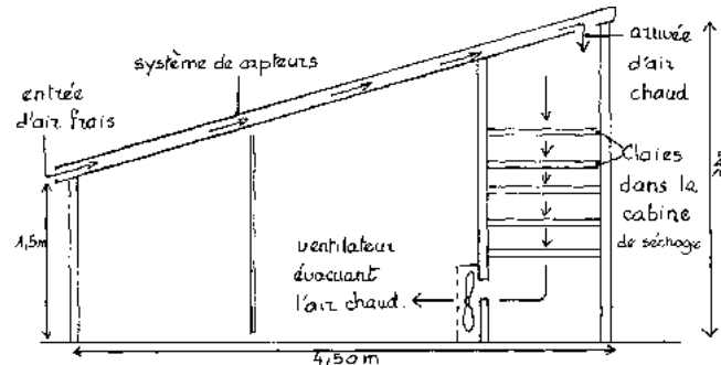
Figure 62: Coupe simplifiée d'un séchoir à convection forcée
