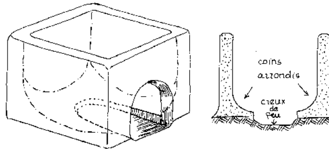
Figure 79: Intérieur d'un four Chokor amélioré
