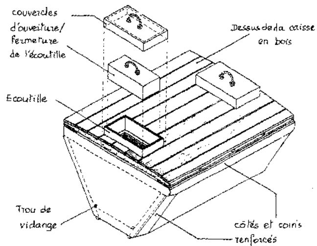
Figure 20: Caisse isotherme dont la forme est adaptée à la pirogue
