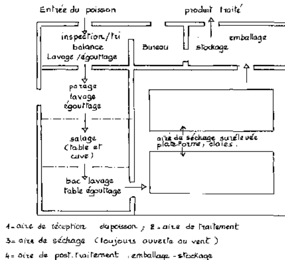
Figure 48: Plan-type d'un atelier pour le salage et le séchage naturel du poisson
