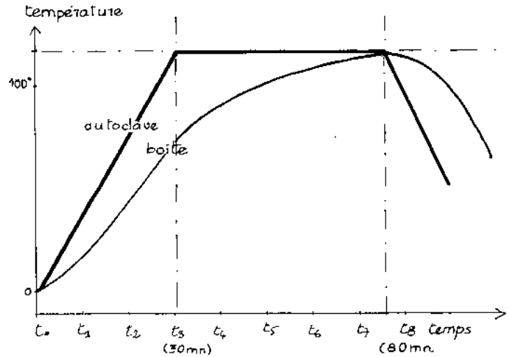
Figure 41: Au cours de la stérilisation, les transferts techniques s'effectuent par convection et/ou conduction
