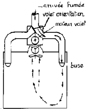
Cellule à inversion de flux
