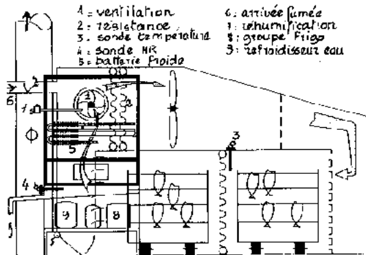
Climatiseur installé sur cellule "Apos"
