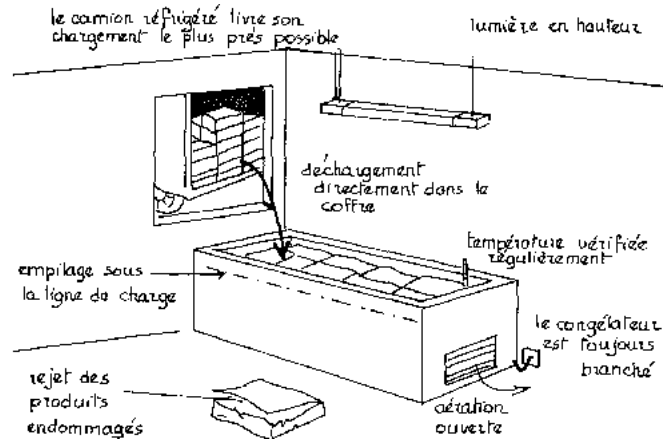
Figure 46: Utilisation correcte d'un coffre de congélation
