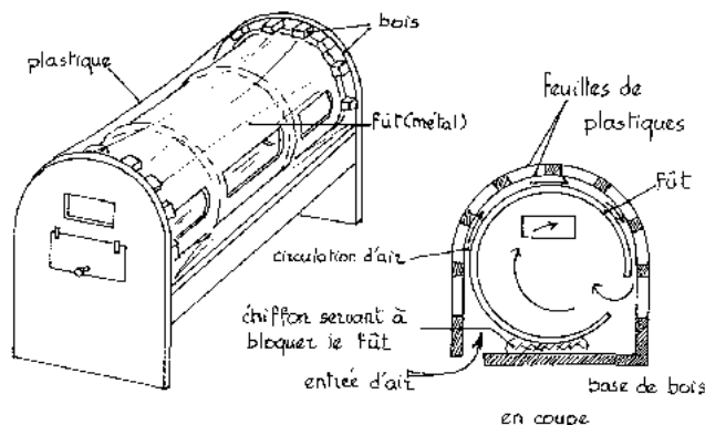
Figure 52: Séchoir solaire réalisé à partir d'un fût
