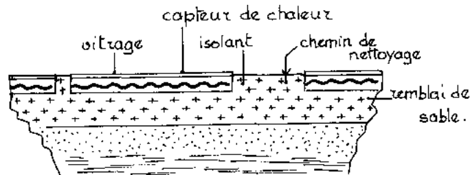
Figure 60: Coupe transversale du capteur solaire Sesol 1.20
