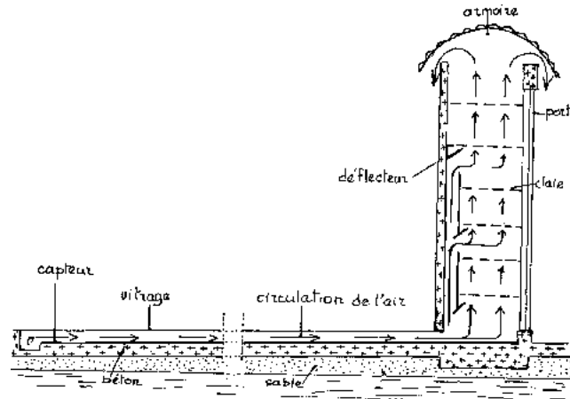
Figure 57: Schéma d'une armoire connectée à un collecteur solaire
