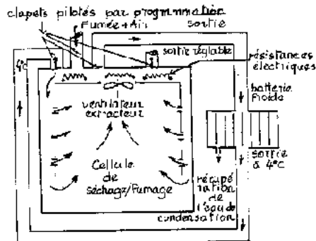
Schéma de principe d'une enceinte de séchage climatique
