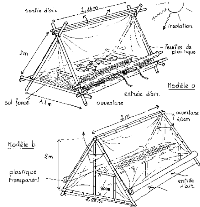
Figures 53 a et 53 b: Tente solaire
