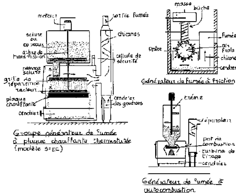
Figure 84: Modes de production de fumée
