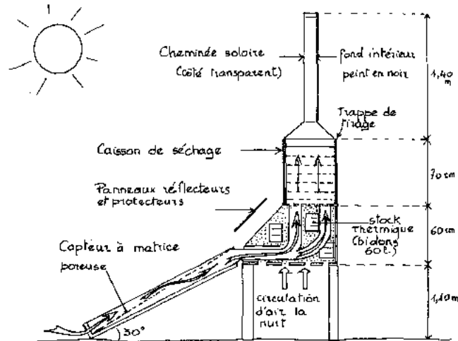
Figure 63: Séchoir solaire à séchage thermique M5 003
