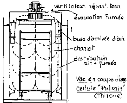
Cellule à inversion de flux
