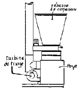
Générateur de fumées conventionnel
