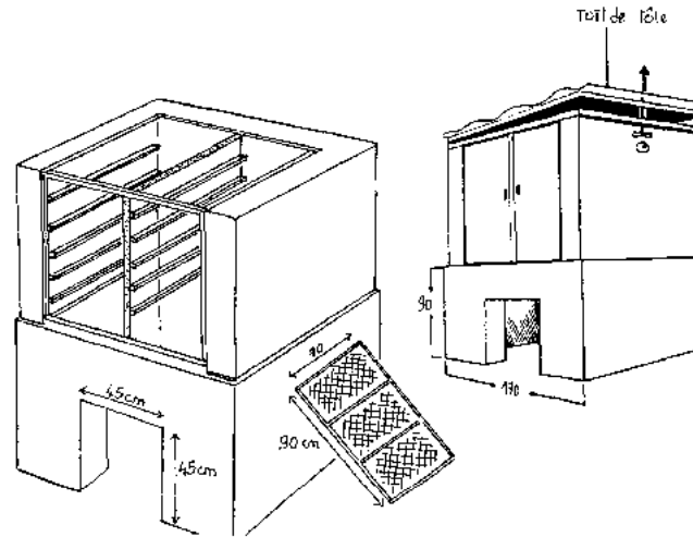
Figure 81: Four Altona plus perfectionné
