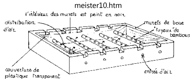
Figure 51: Boîte de séchage aux Philippines
