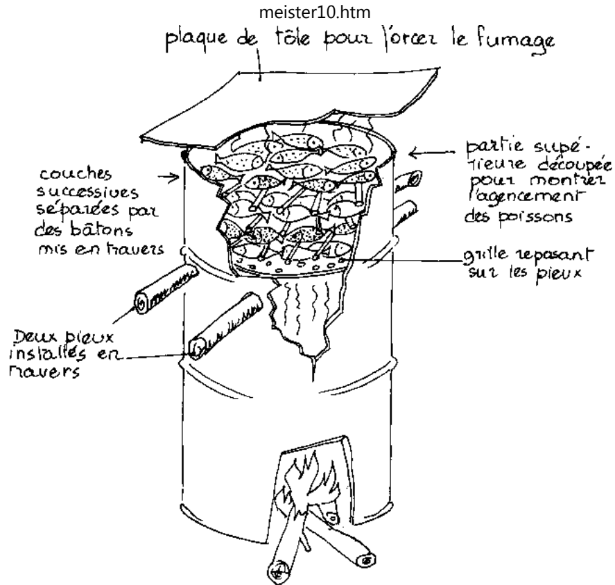
Figure 28: Fumage traditionnel sur fût métallique
