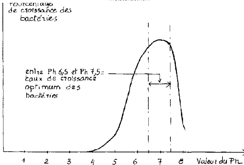
Figure 40: Développement des bactéries en fonction du pH
