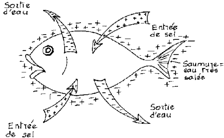
Figure 35: Mouvements de l'eau et du sel lors du salage
