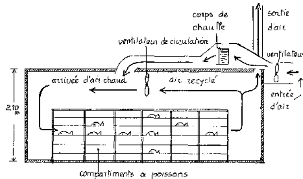
Figure 67: Tunnel de séchage (brésilien)
