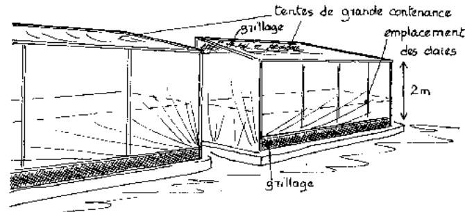
Figure 54: Grandes tentes solaires en polyéthylène (Joal)
