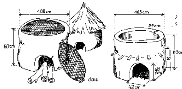
Figure 68: Four traditionnel en boue maniée
