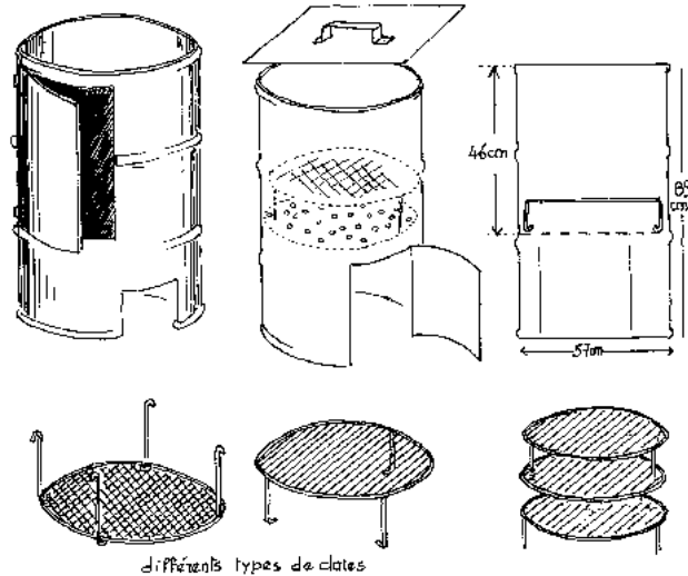
Figure 70: Four réalisés avec un fût métallique entier
