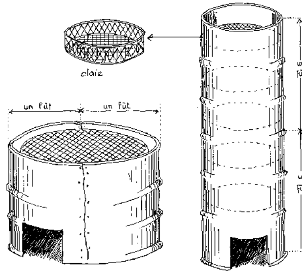
Figure 71: Four réalisé avec deux fût métallique soudés
