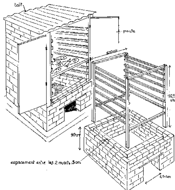
Figure 80: Four en maçonnerie (l'armature est en bois)
