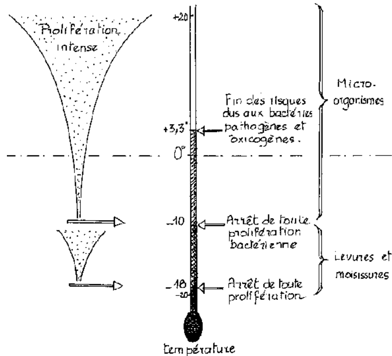
Figure 11: Action de la température sur la multiplication et la toxicogénèse des micro-organismes responsables des contaminations des denrées alimentaires
