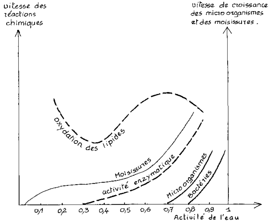
Figure 12: Relation entre la valeur de l'activité de l'eau, la croissance des microorganismes et la vitesse des réactions chimiques
