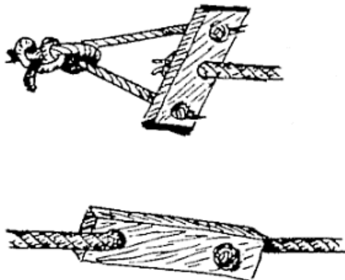
FIG. 145.—Swivels.
