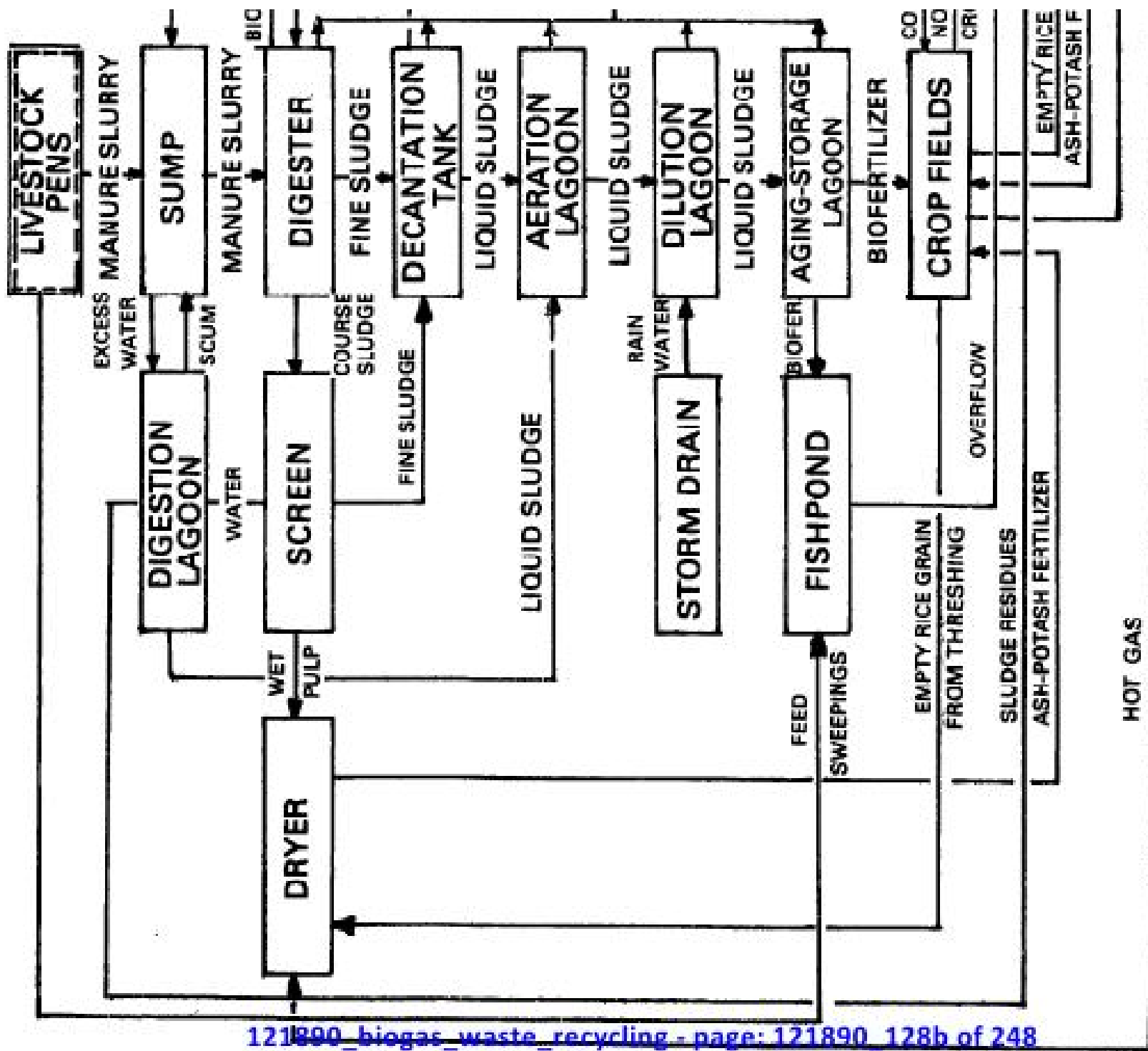
FIG. 9-3 AGRO-PULP BIOG
