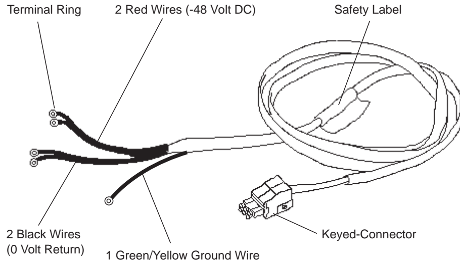
Figure 11. -48 Volt DC Input Power Cord
