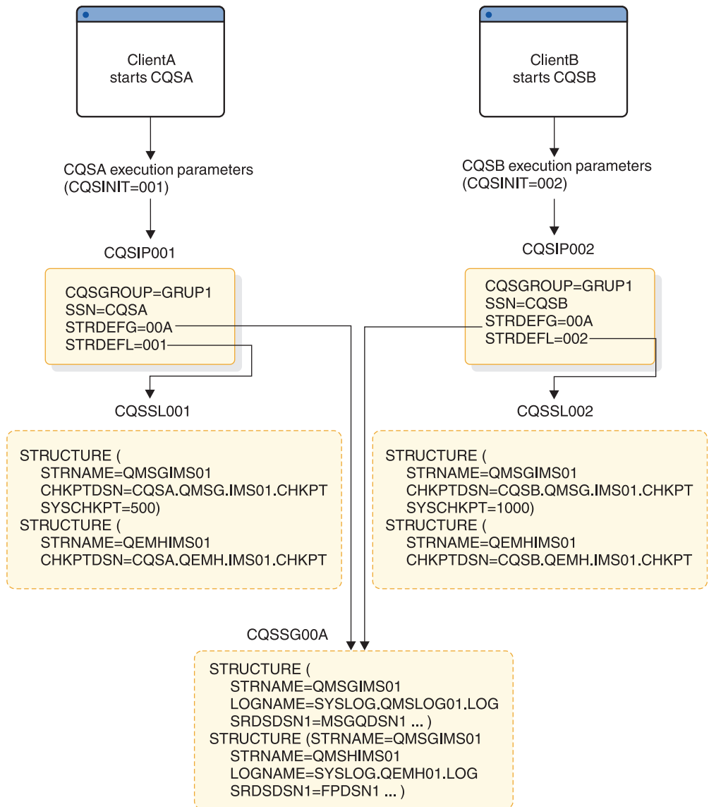
Figure 53. Specifying IMS and CQS parameters
