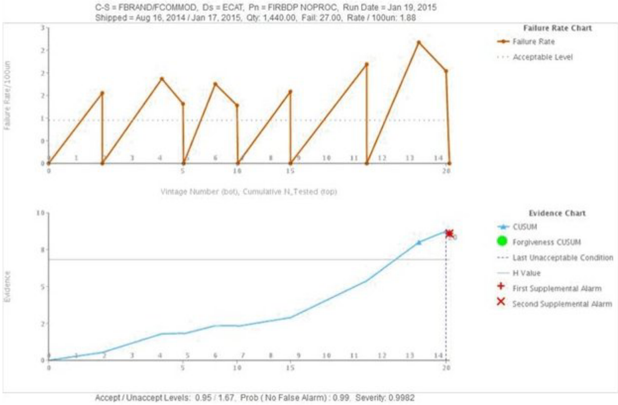
图 17. 检查图表 3
