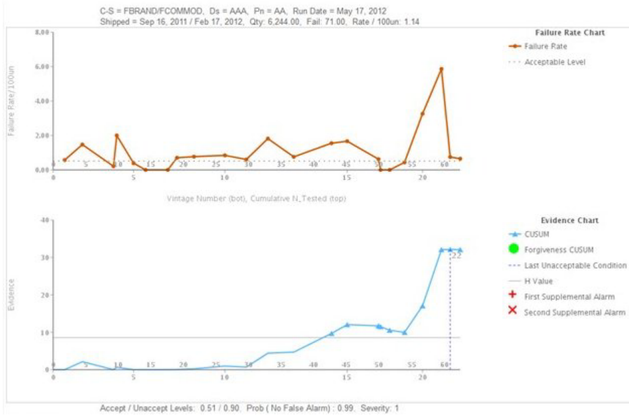
图 15. 检查图表 1
