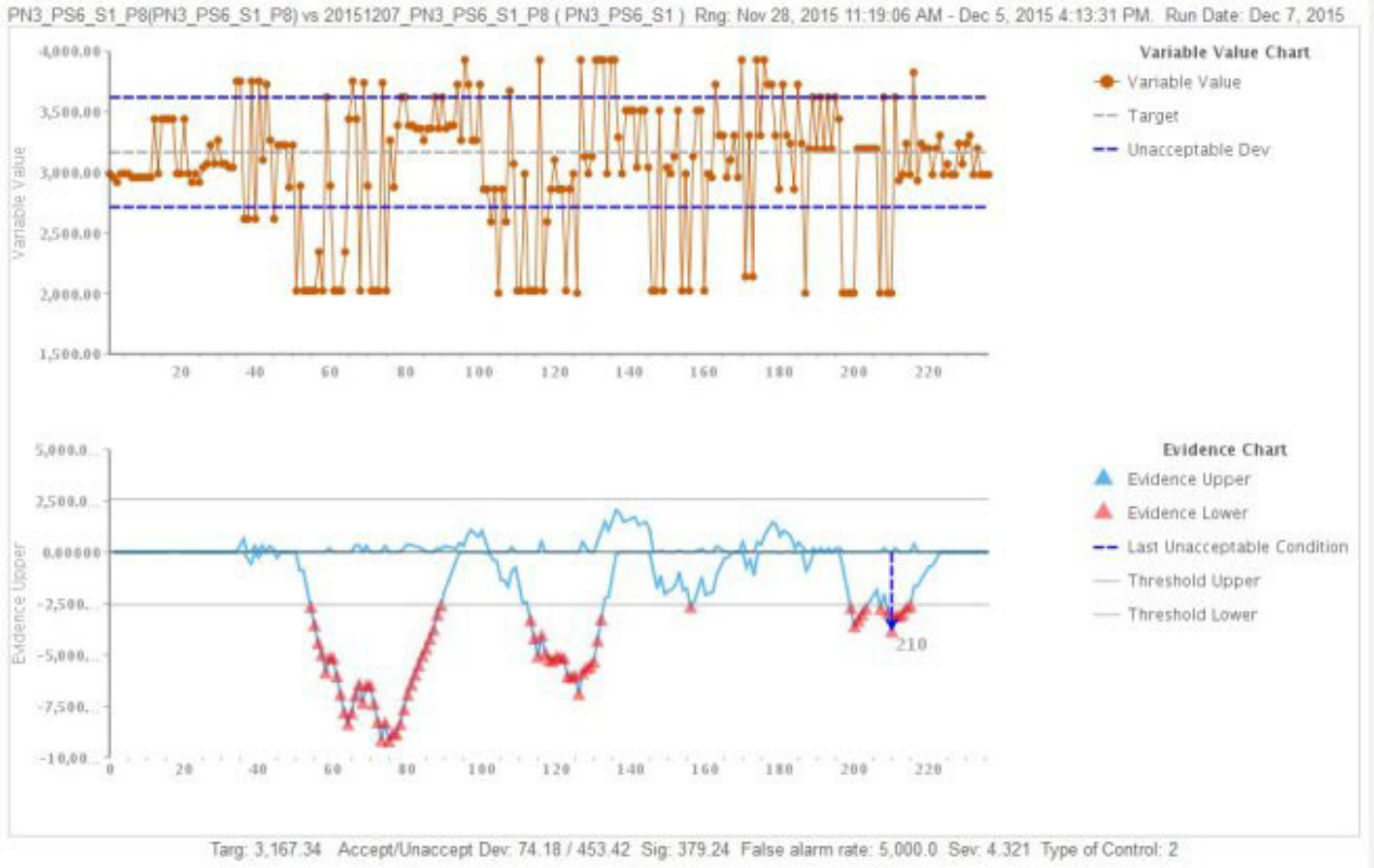
图 19. 参数化图表 1
