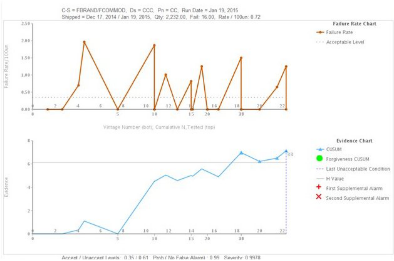
图 16. 检查图表 2
