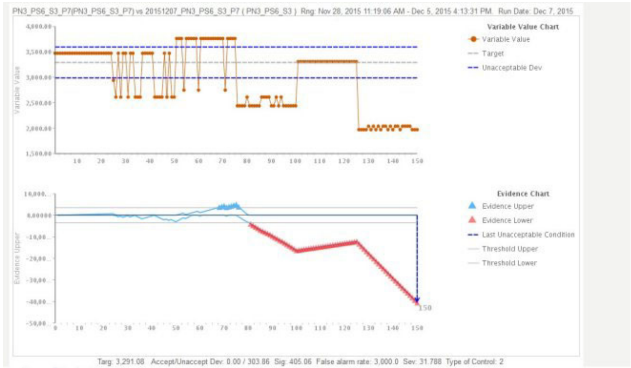
图 21. 参数化图表 3
