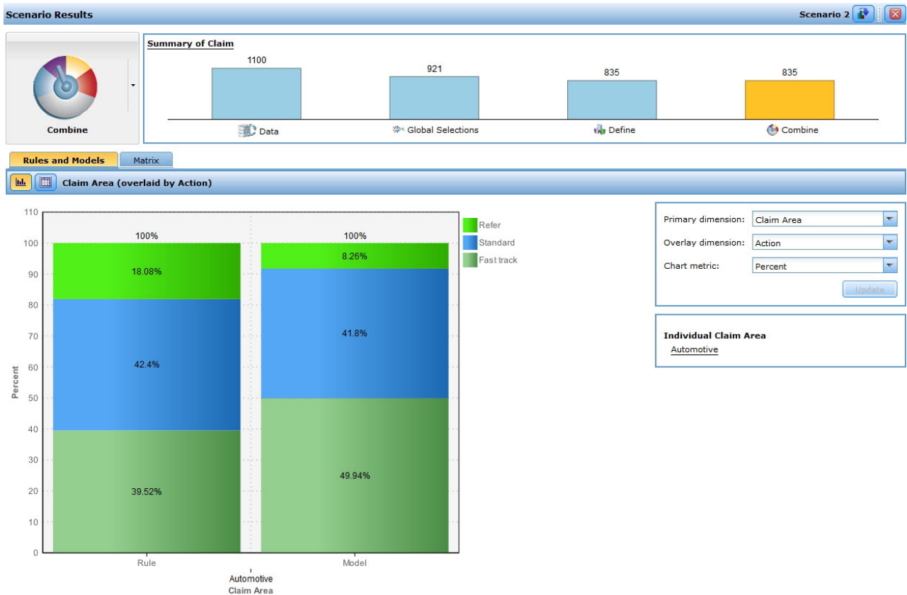
図 11. シナリオの実行
