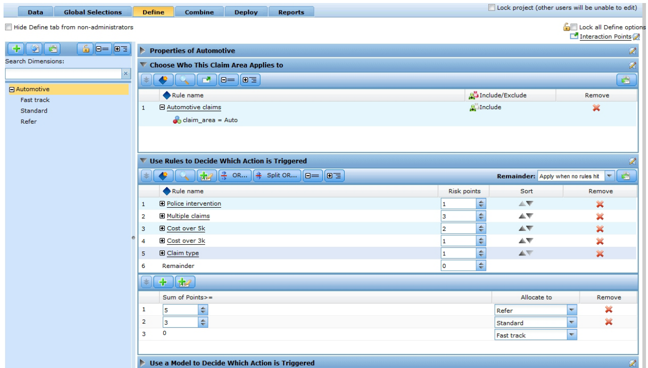
図5. 「自動車関連」のプロパティを表示する「定義」タブ
