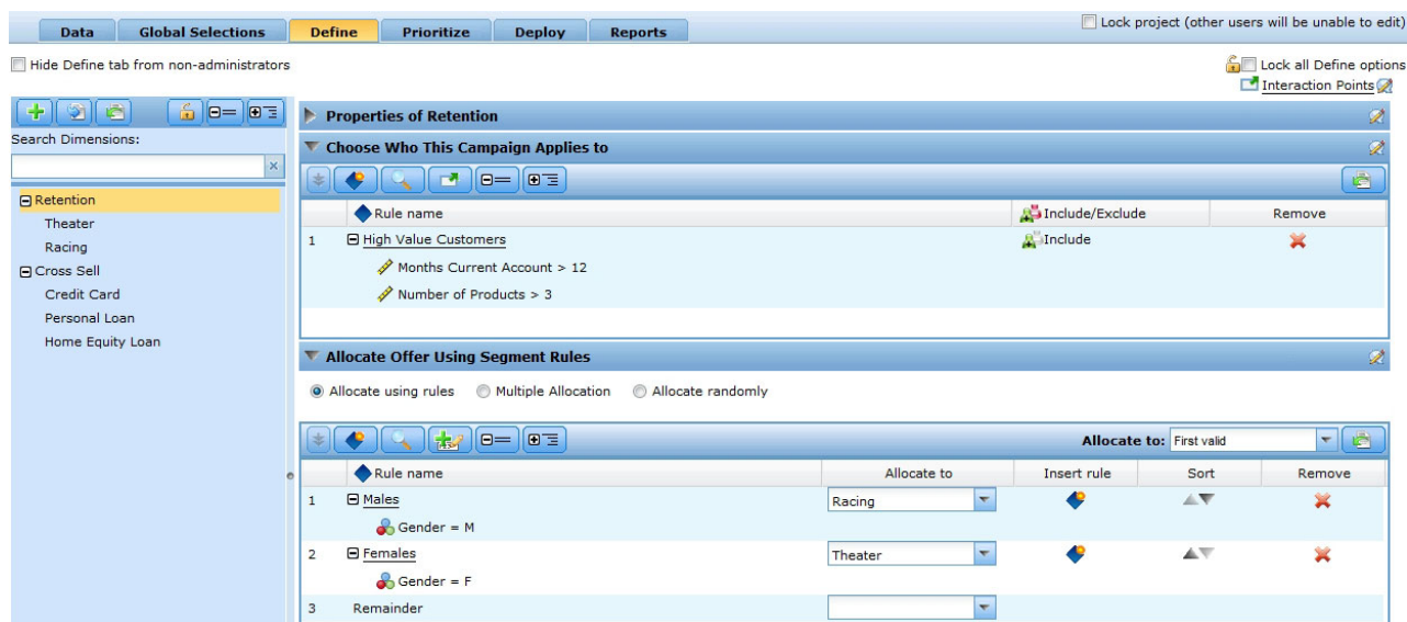
図5. 「顧客維持」キャンペーンのプロパティを表示する「定義」タブ
