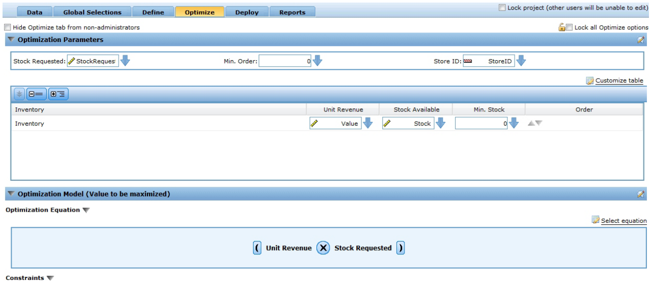
図 5. 「最適化」タブ
