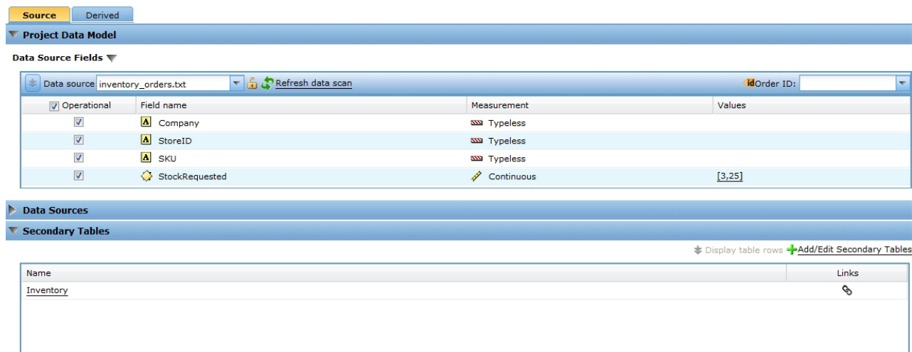
図3. 「データ」タブ
