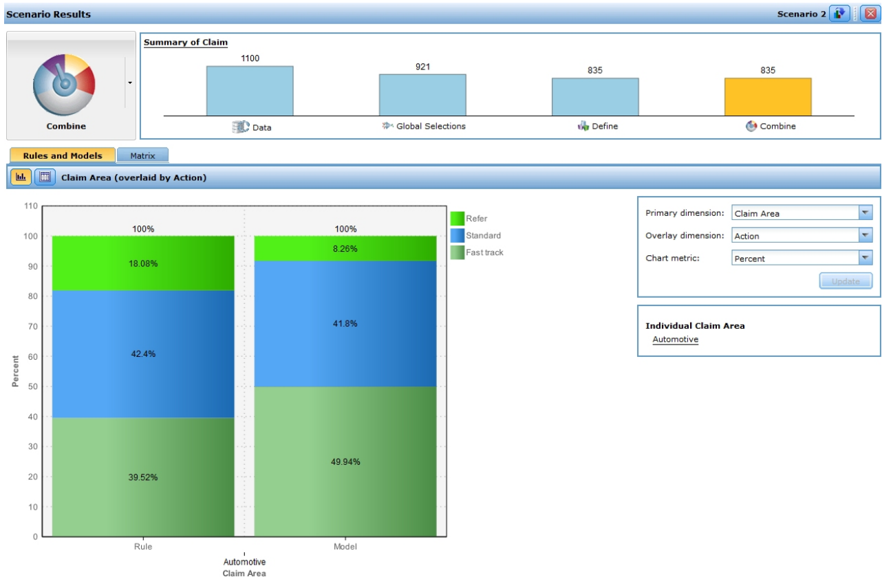
Figura 11. Running a scenario
