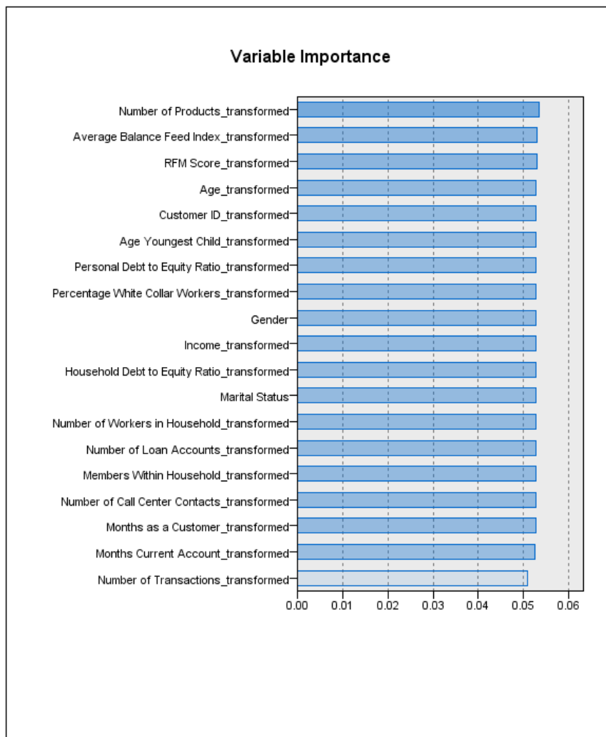
変数の重要度
