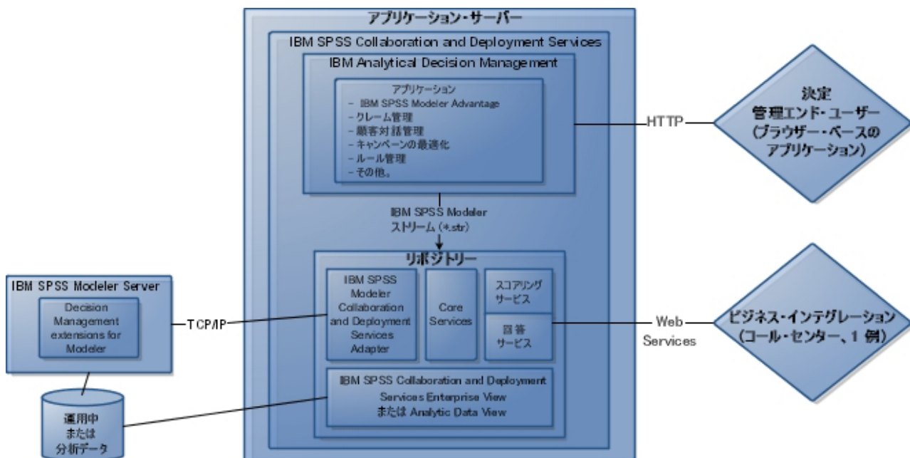
図 1. IBM Analytical Decision Management のインフラストラクチャ
