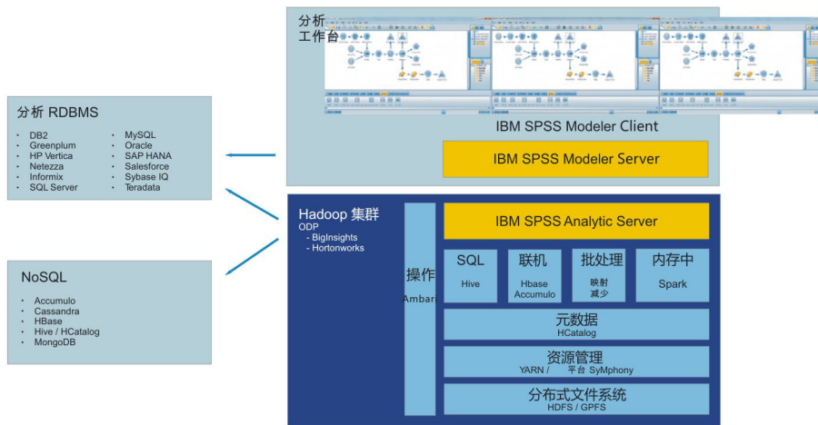
图 1. 体系结构
