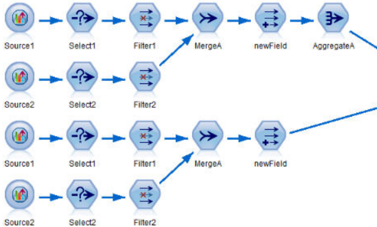
Abbildung 8. Beispieldatenstrom
