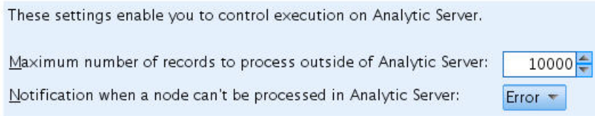
Abbildung 7. Analytic Server-Einstellungen
