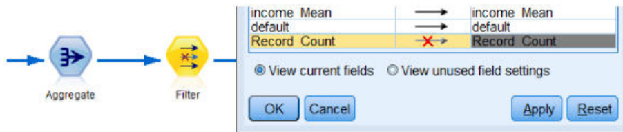
Abbildung 6. Modeler-Feldoptionen
