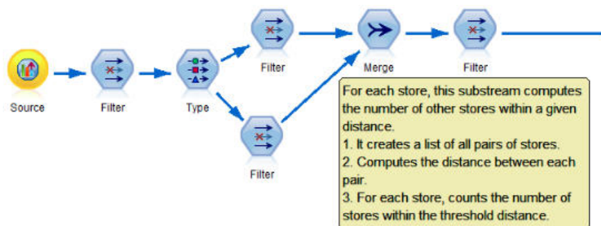
图 12. 包含注释的流示例
