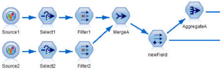
图 9. 示例流
