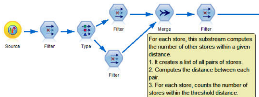
図 53. コメント付きストリームの例
