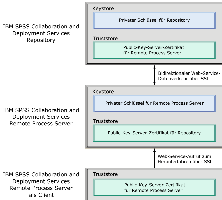
Abbildung 1. SSL-Architektur für IBM SPSS Collaboration and Deployment Services Remote Process Server
