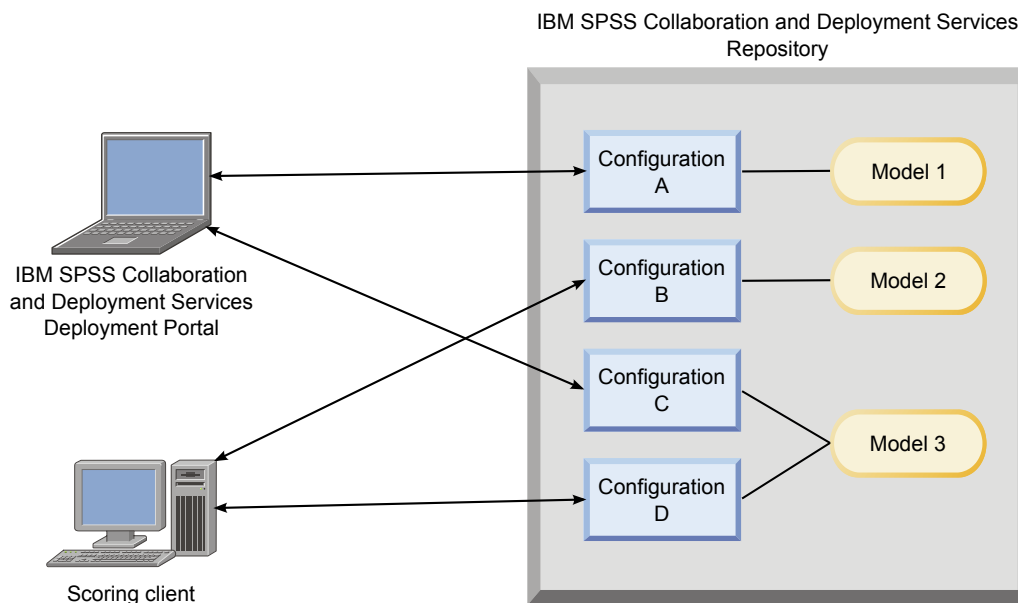
Figura 6. Arquitectura de puntuación general
