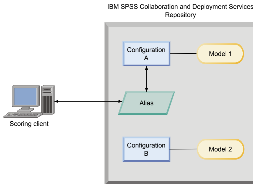
Figura 7. Ejemplo de alias para configuraciones de puntuación
