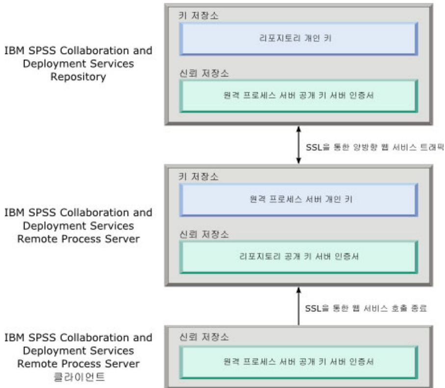
그림 1. IBM SPSS Collaboration and Deployment Services Remote Process Server의 SSL 아키텍처
