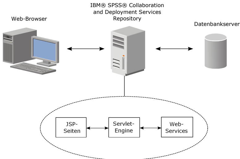
Abbildung 1. JSP-Architektur
