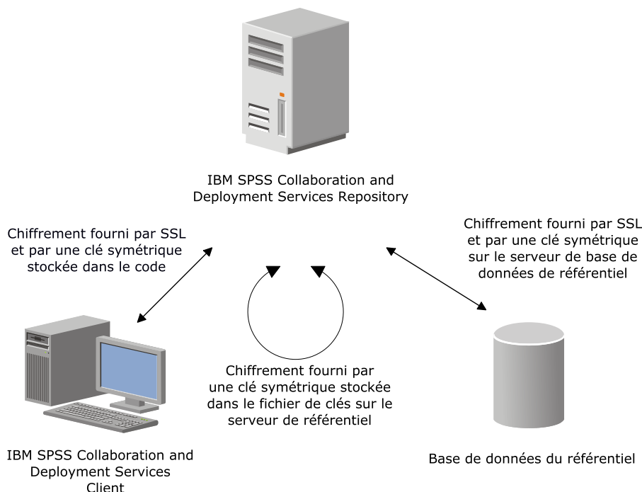
Figure 4. Configuration de la sécurité conforme à la norme FIPS 140-2 de IBM SPSS Collaboration and Deployment Services
