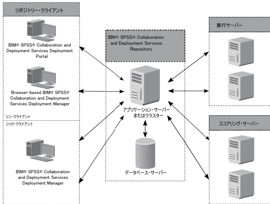
図 1. IBM SPSS Collaboration and Deployment Services のアーキテクチャ
