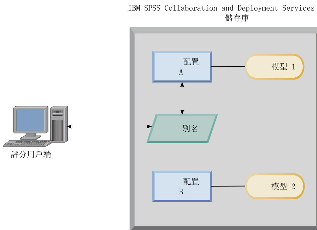
圖 7. 用於評分配置的別名範例
