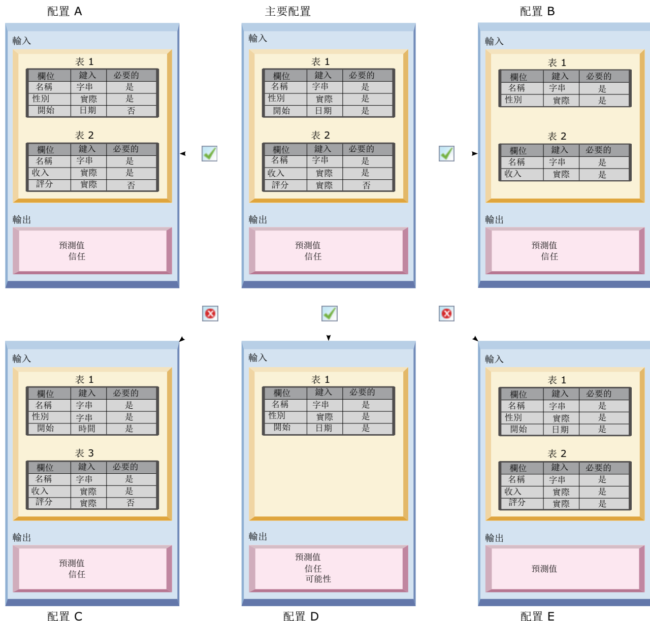
圖 9. 評分配置相容性
