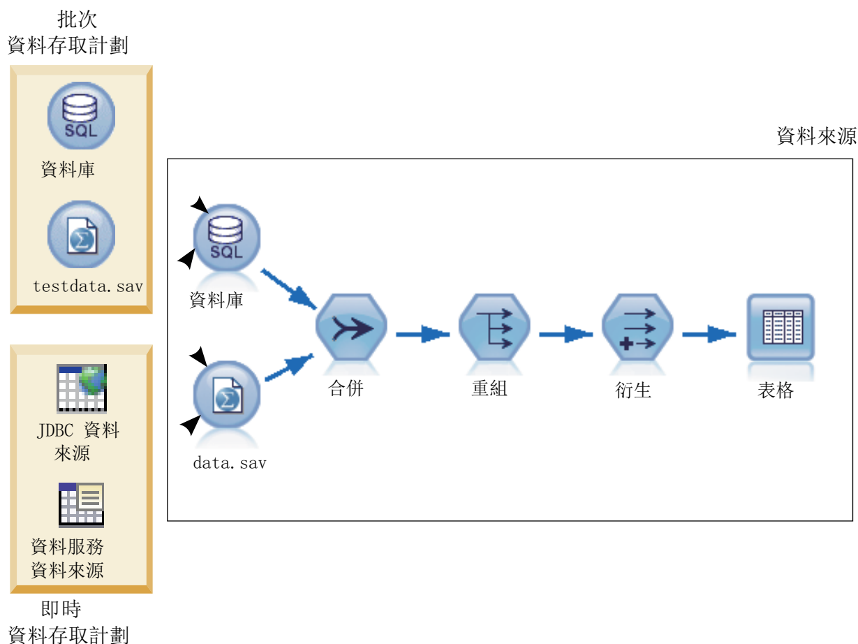
圖 3. 資料來源的資料存取計劃
