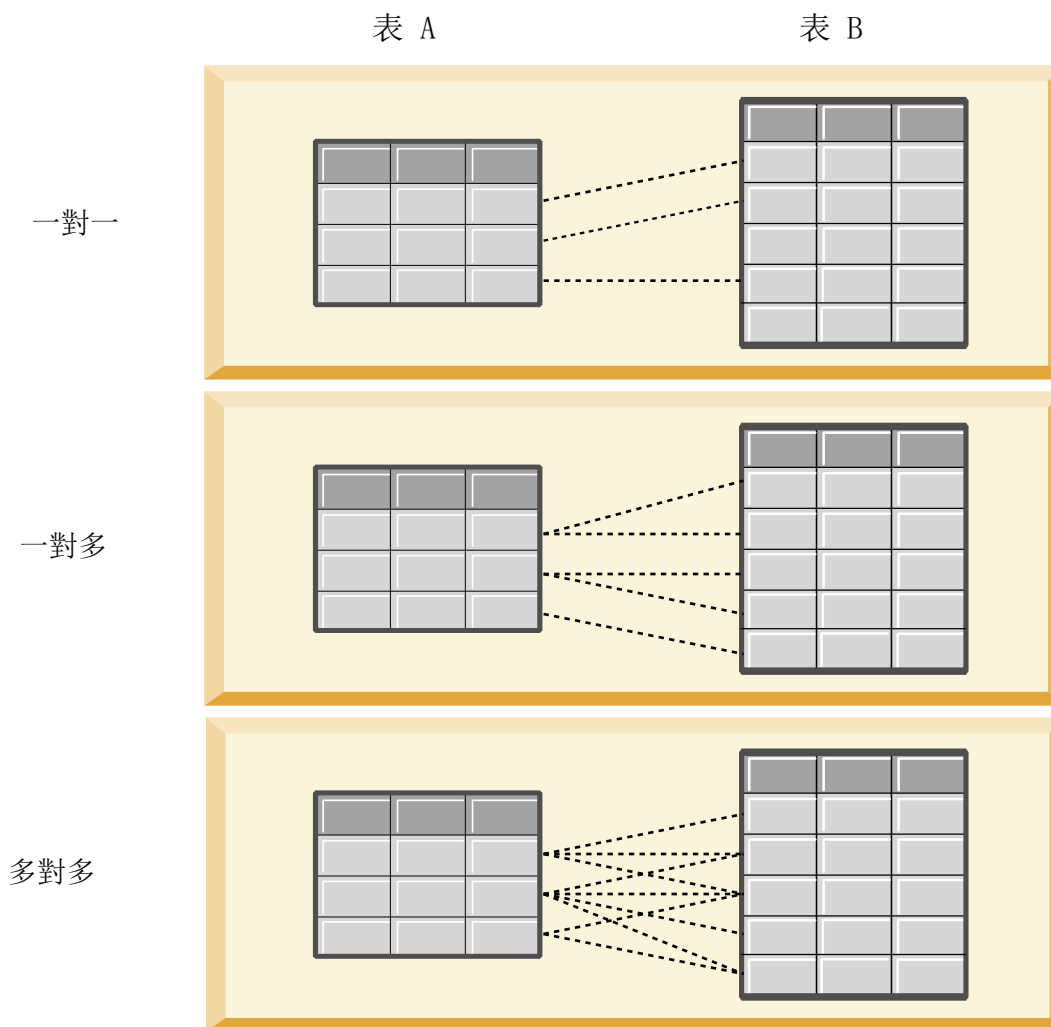
圖 4. 表格關係類型
