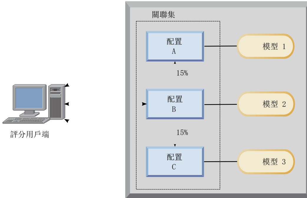
圖 8. 用於評分配置的關聯集範例
