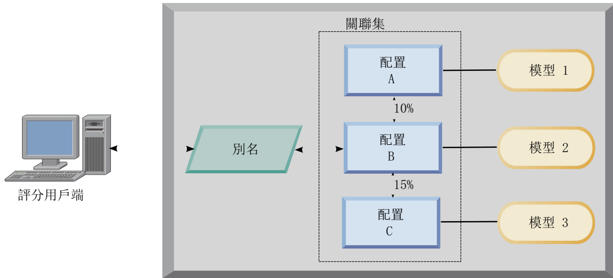
圖 10. A/B 測試範例
