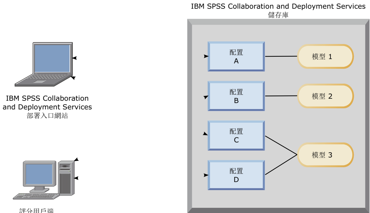
圖 6. 一般評分架構
