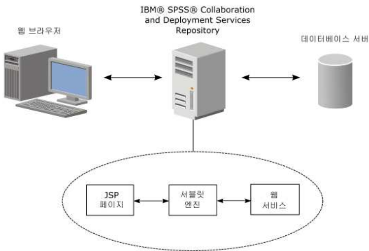
그림 1. JSP 아키텍처
