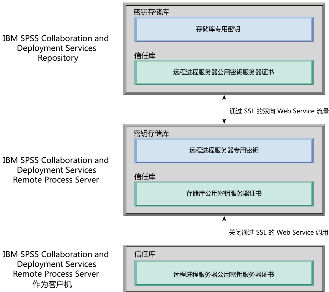
图 1. IBM SPSS Collaboration and Deployment Services Remote Process Server 的 SSL 体系结构
