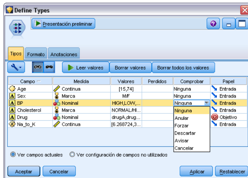
Figura 4-28 Selección de opciones de comprobación para el campo seleccionado
