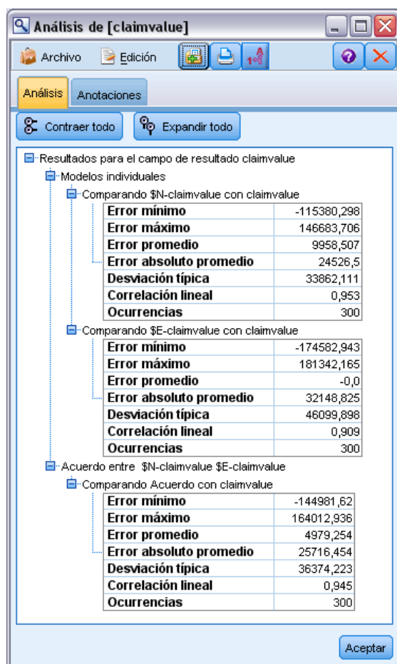
Figura 6-13 Explorador de resultados de análisis
