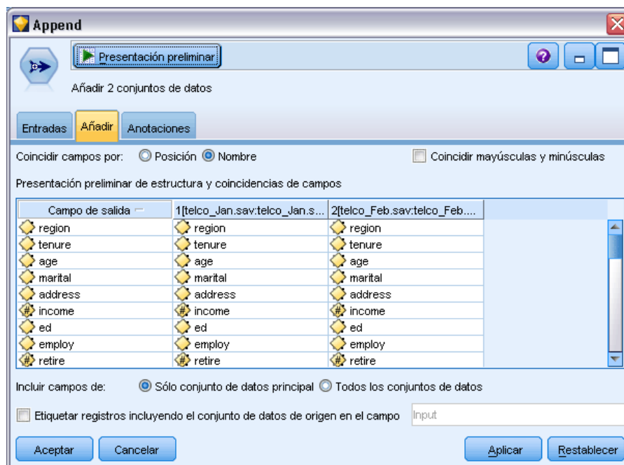
Figura 3-22 Cuadro de diálogo del nodo Añadir con una correspondencia de campos por nombre.
