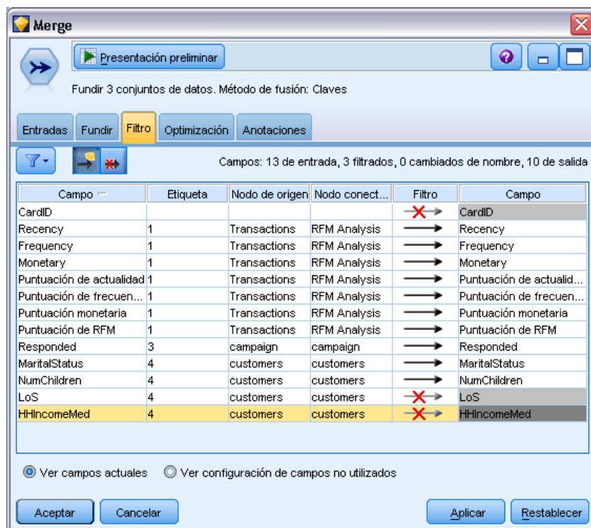
Figura 3-18 Filtrado desde el nodo Fundir
