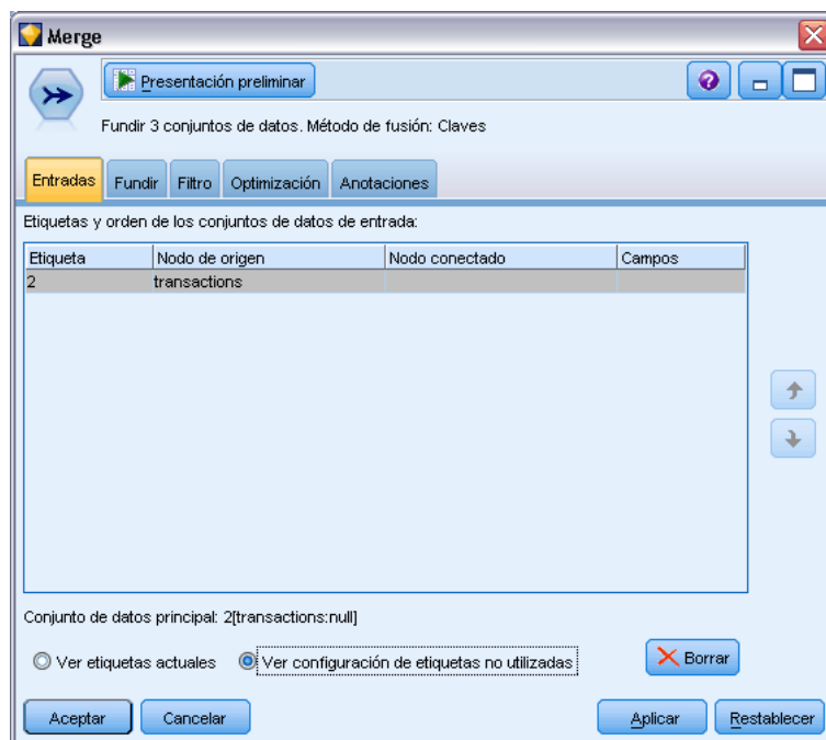
Figura 3-20 Eliminación de etiquetas no utilizadas del nodo Fundir
