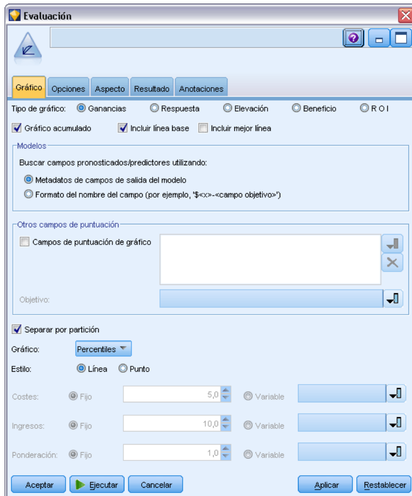
Figura 5-63 Configuración de la pestaña Gráfico de un nodo Evaluación
