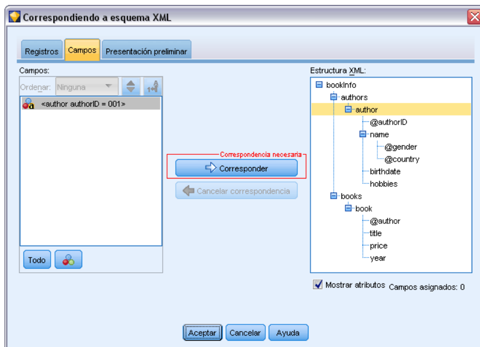
Figura 7-15 Campos de correspondencia XML
