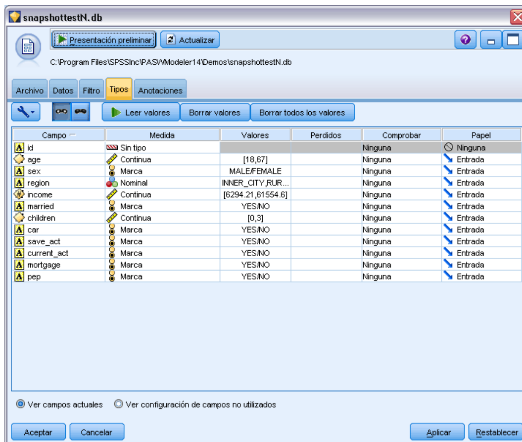
Figura 2-34 Opciones de la pestaña Tipos
