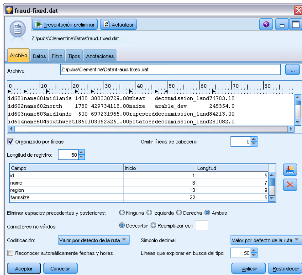
Figura 2-12 Especificación de columnas en los datos de campo fijo
