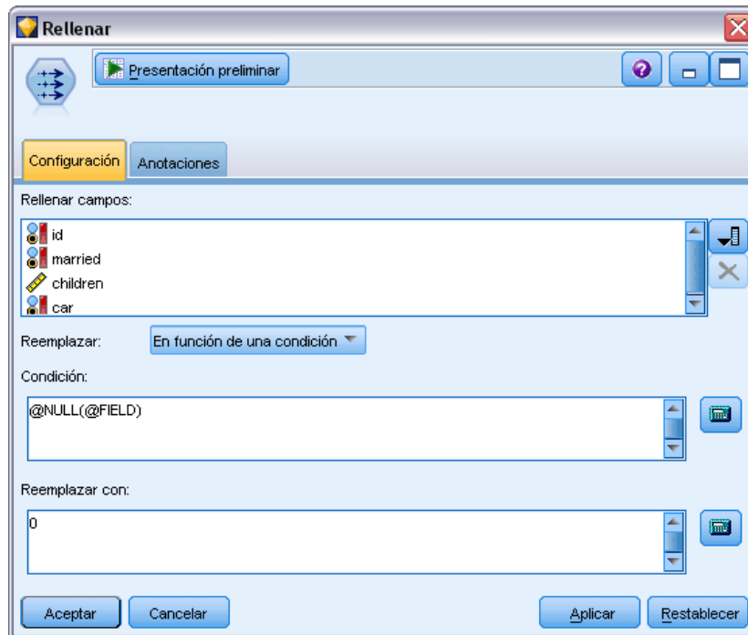
Figura 4-53 Cuadro de diálogo del nodo Rellenar
