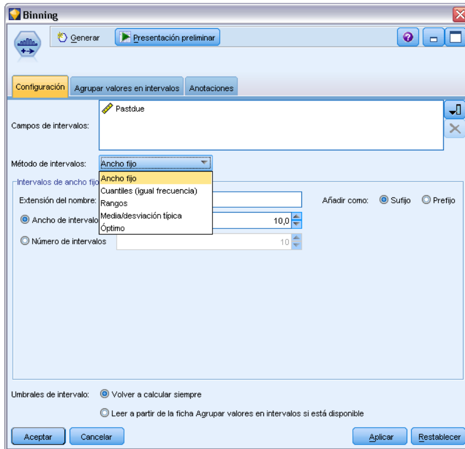
Figura 4-63 Cuadro de diálogo del nodo Intervalos, pestaña Configuración
