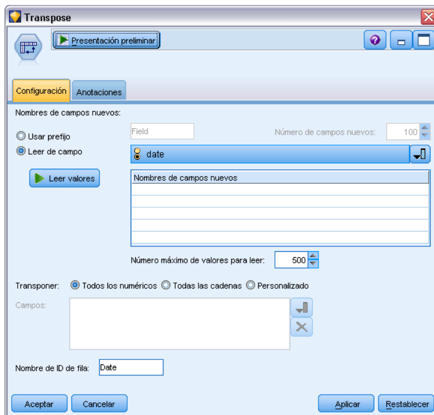
Figura 4-80 Lectura de nombres de campo de un campo existente
