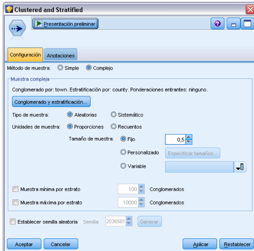
Figura 3-4 Opciones de muestreo complejo
