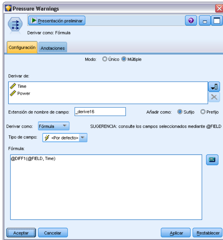
Figura 4-43 Derivación de múltiples campos
