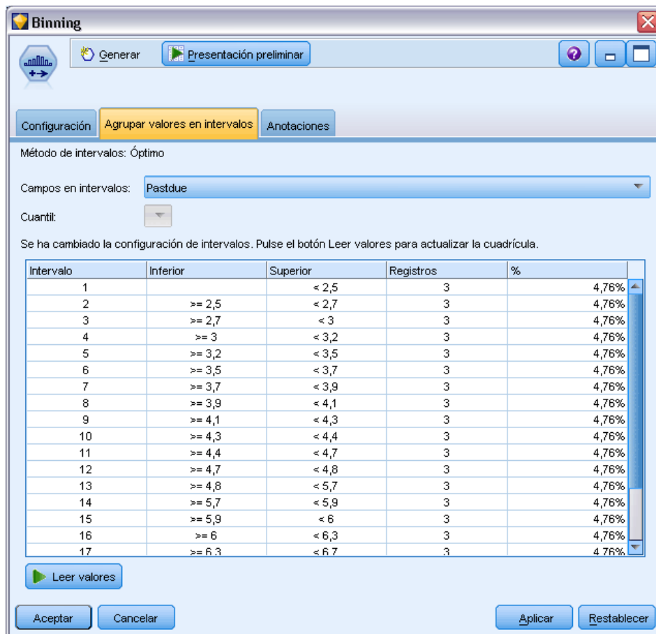
Figura 4-71 Cuadro de diálogo del nodo Intervalos, pestaña Agrupar valores en intervalos
