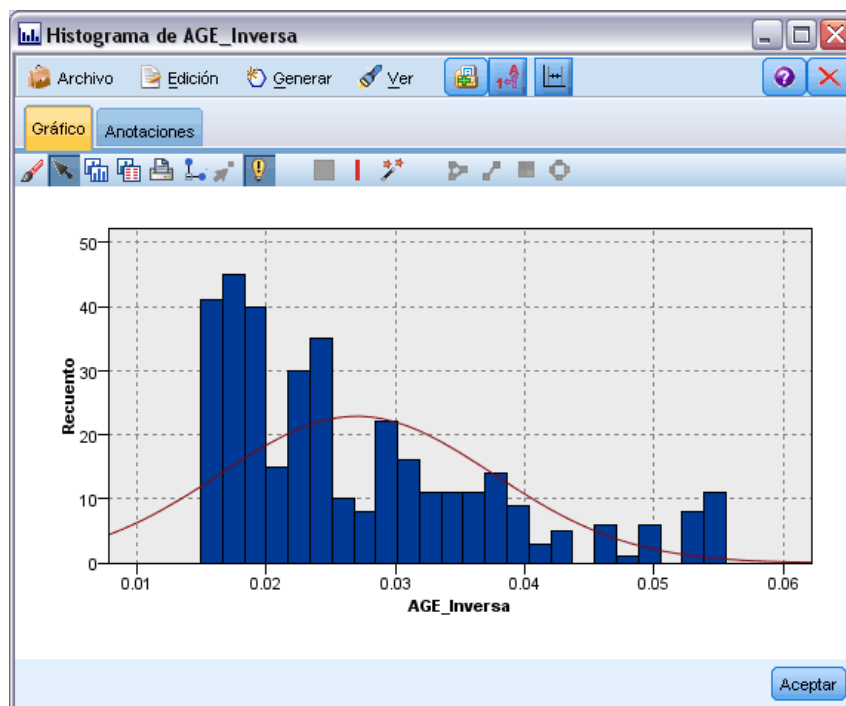
Figura 6-35 Histograma de transformación con curva de distribución normal superpuesta
