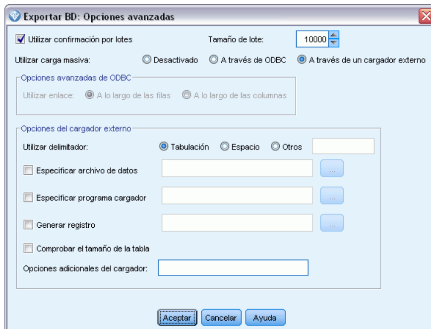
Figura 7-6 Especificación de opciones avanzadas para la exportación de la base de datos
