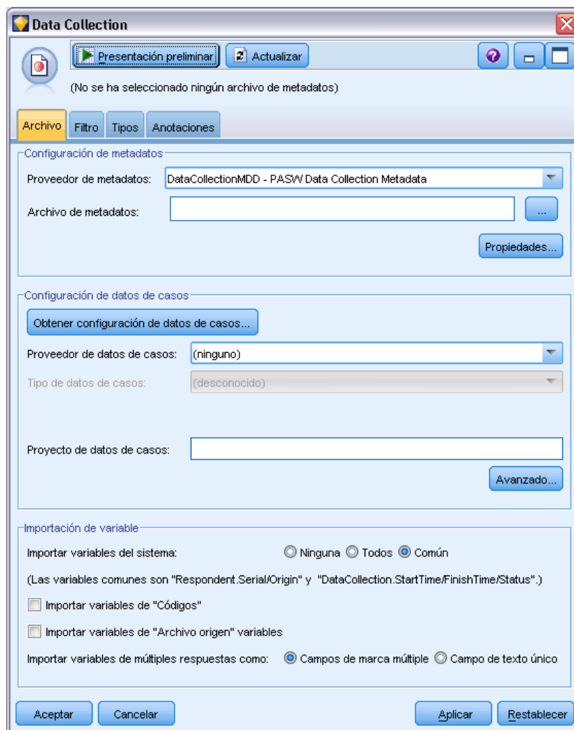
Figura 2-15 Opciones de archivo del nodo de origen Data Collection
