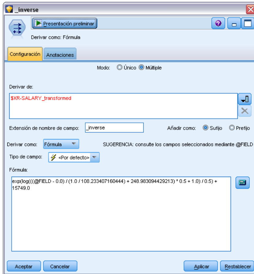
Figura 4-18 Nodo Derivar generado desde el nodo Preparación automática de datos
