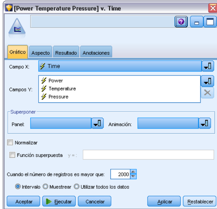
Figura 5-38 Configuración de la pestaña Gráfico de un nodo G. múltiple
