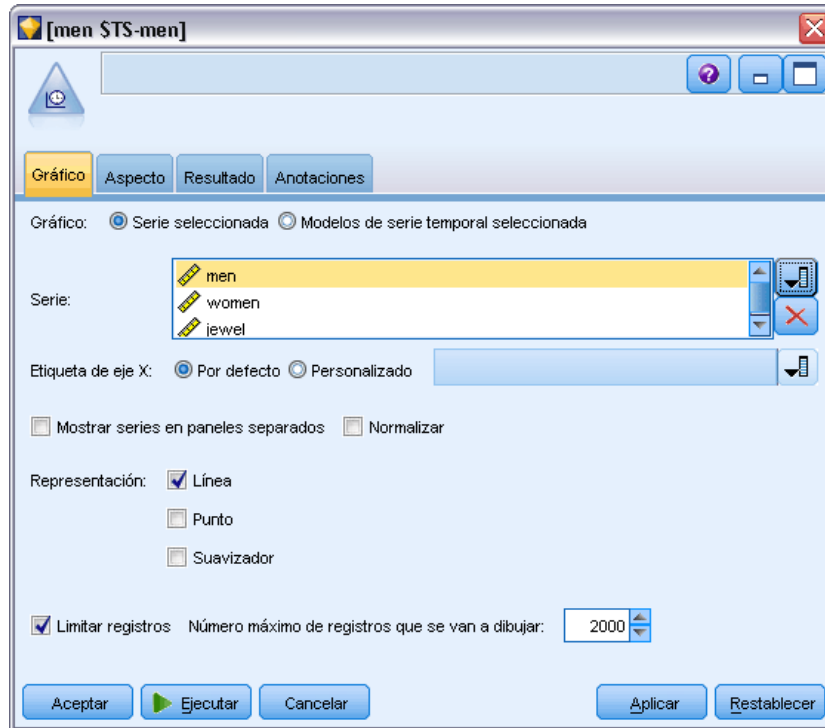
Figura 5-55 Configuración de la pestaña Gráfico de un nodo Gráfico de Tiempo
