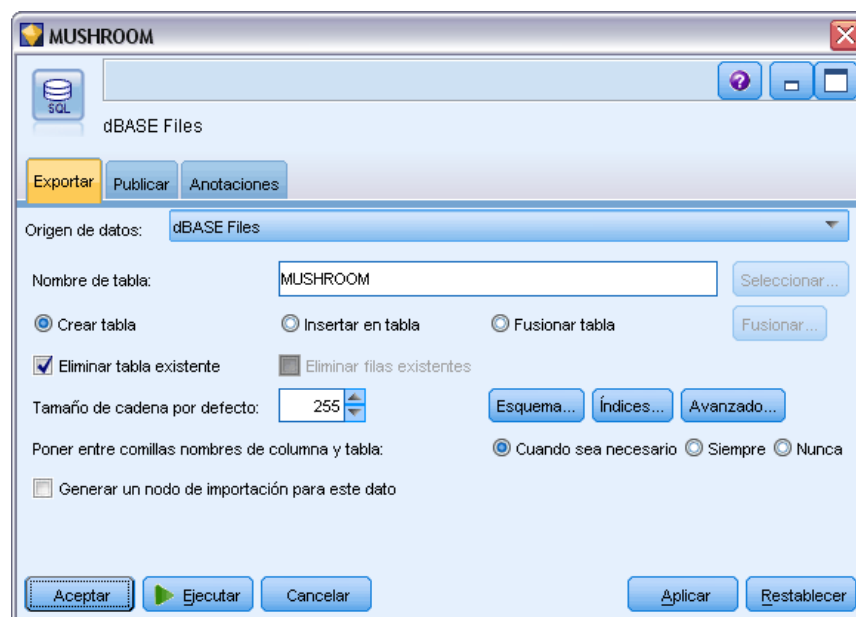
Figura 7-1 Nodo Exportar base de datos, pestaña Exportar
