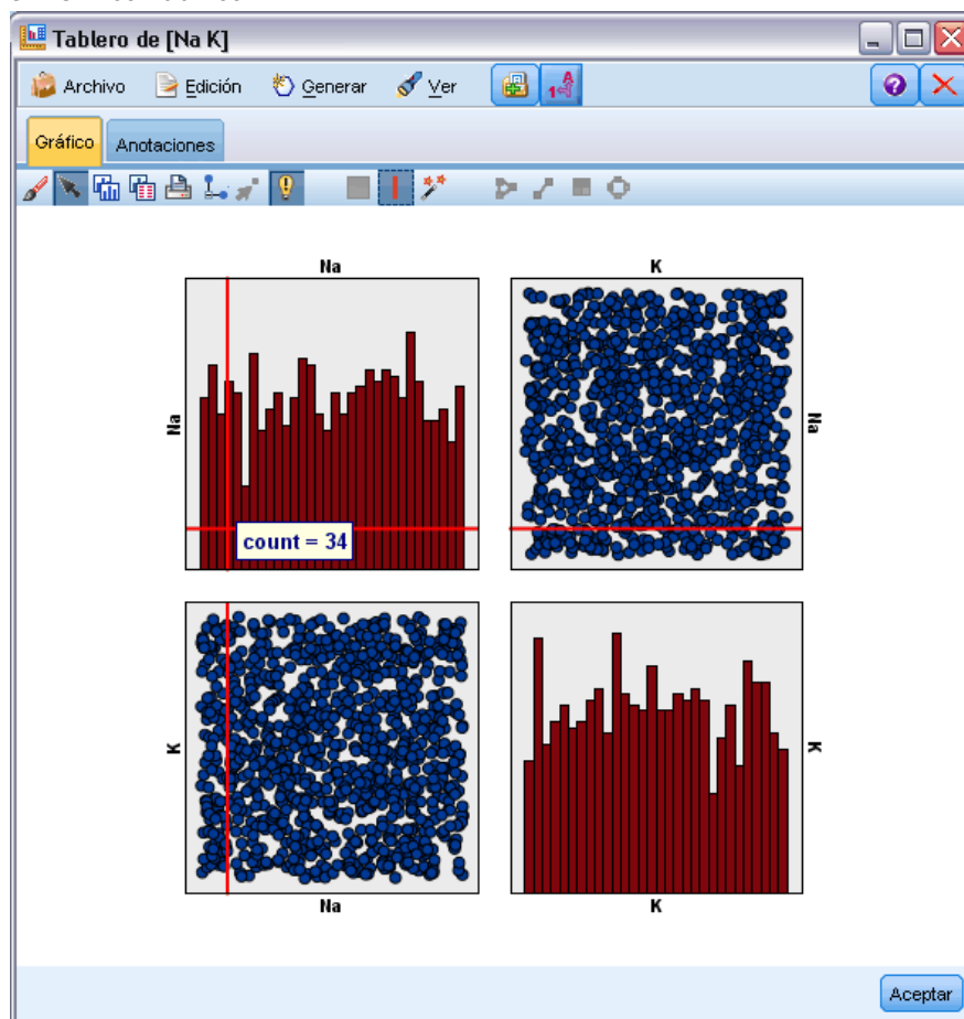
Figura 5-71 SPLOM con tramos
