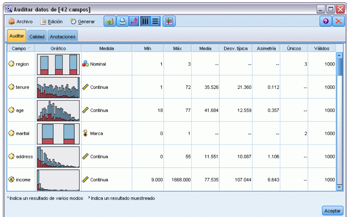
Figura 6-14 explorador de auditoría de datos
