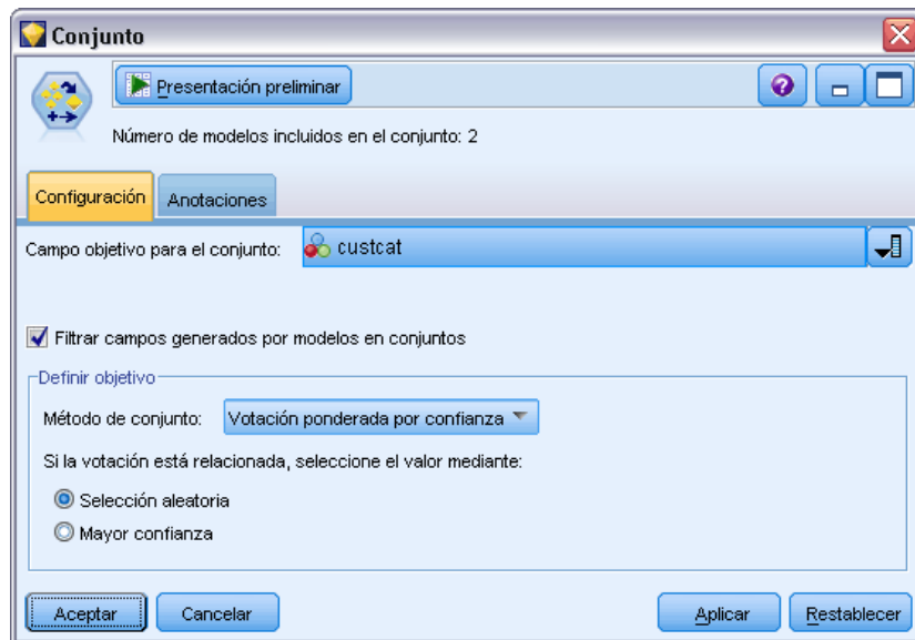
Figura 4-40 Nodo Conjunto con un campo nominal seleccionado como objetivo
