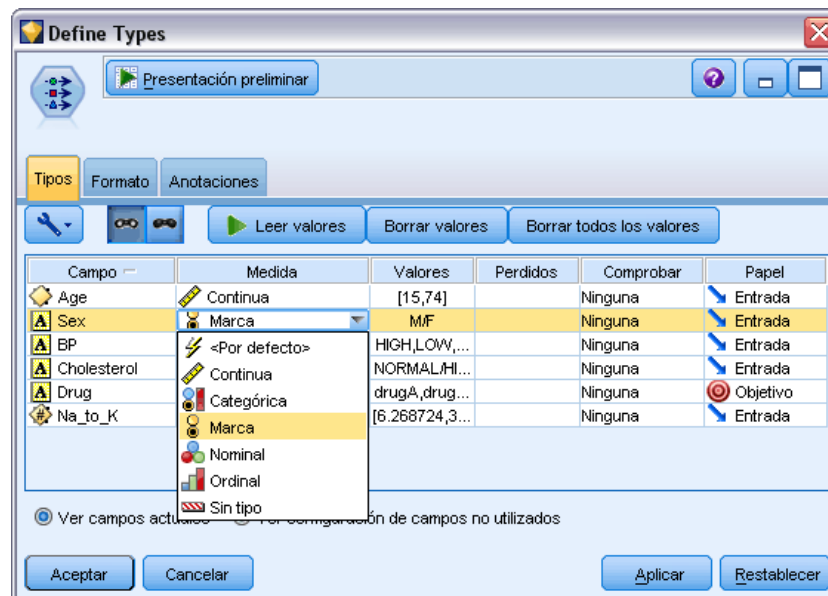
Figura 4-20 Configuración manual de los niveles de medición
