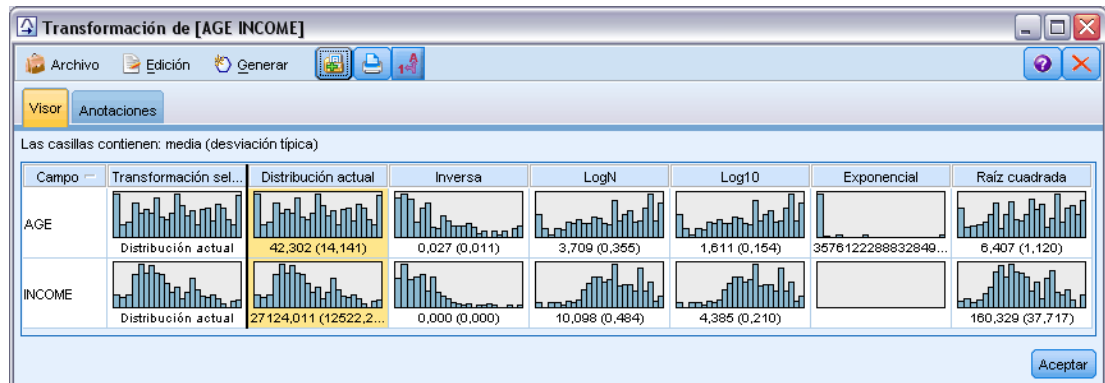
Figura 6-32 Visualización de transformaciones disponibles por campo
