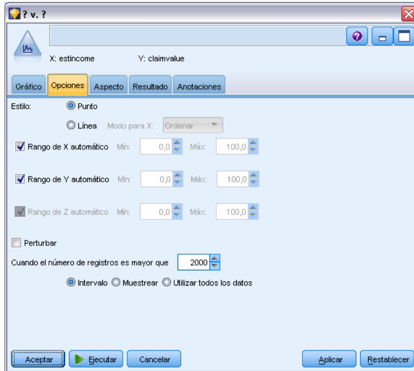
Figura 5-20 Configuración de la pestaña Opciones de un nodo Gráfico
