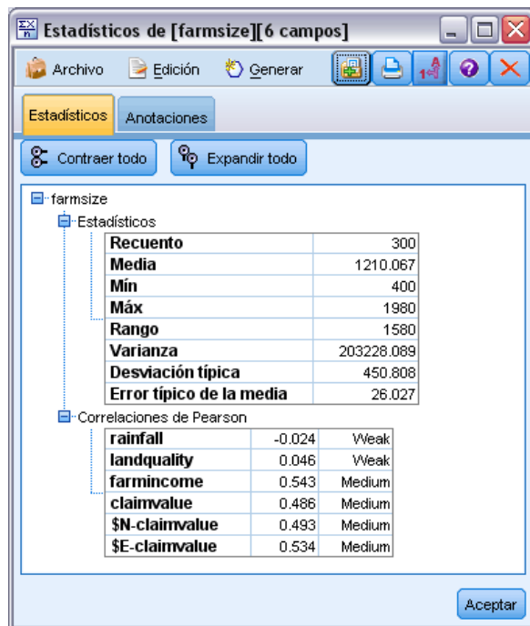
Figura 6-38 Explorador de resultados de estadísticos
