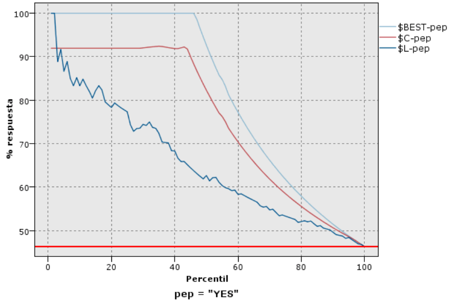
Figura 5-60 Gráfico de respuestas (acumulado) con mejor línea
