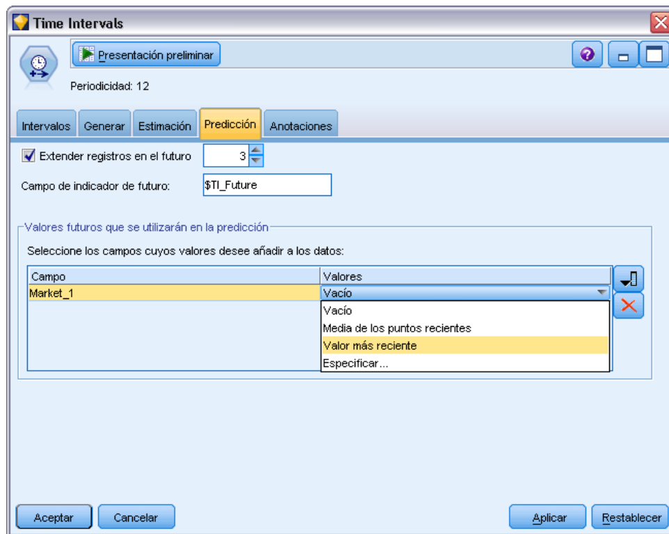
Figura 4-87 Nodo Intervalos de tiempo, pestaña Predicción
