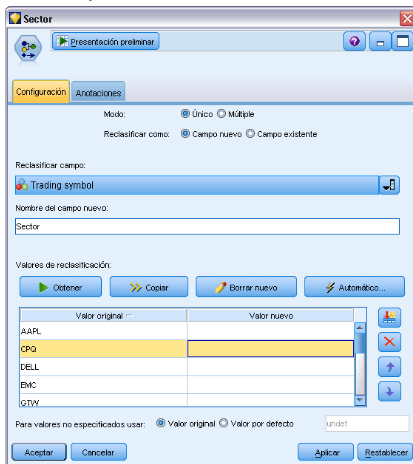
Figura 4-60 Cuadro de diálogo del nodo Reclasificar
