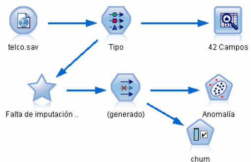
Figura 6-15 Ruta con Supernodo de valores perdidos
