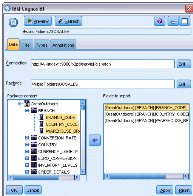
Figura 2-21 Importación de datos de Cognos
