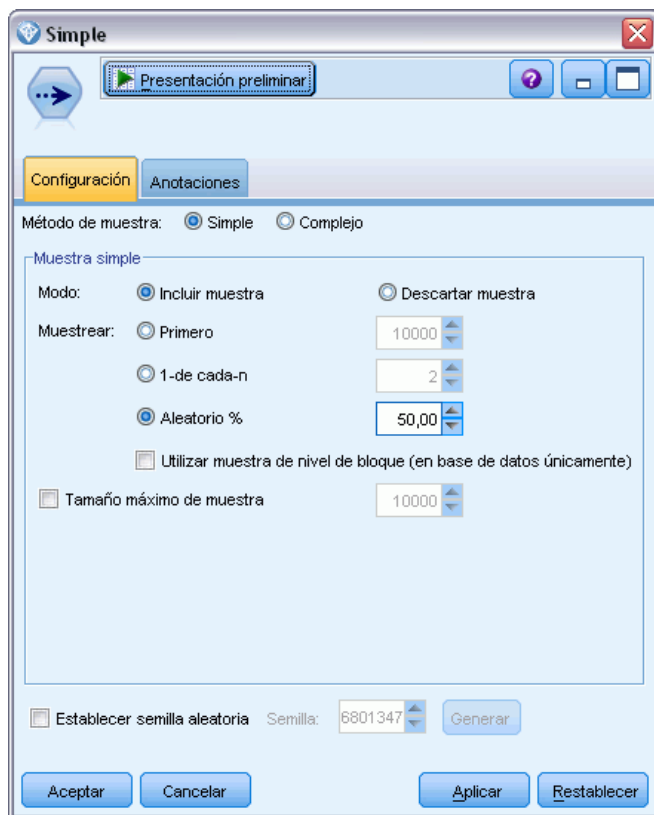
Figura 3-3 Opciones de muestreo simple
