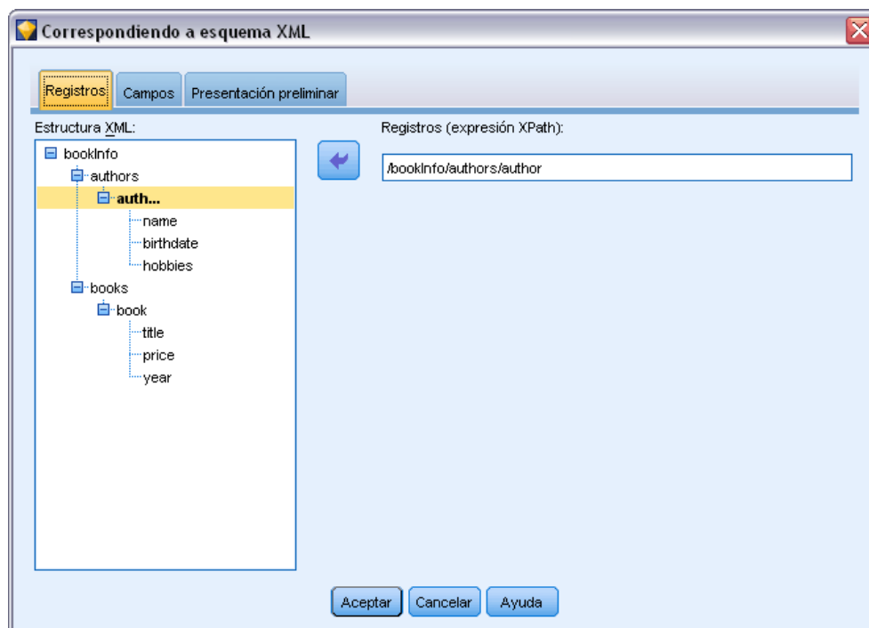
Figura 7-14 Registros de correspondencia XML
