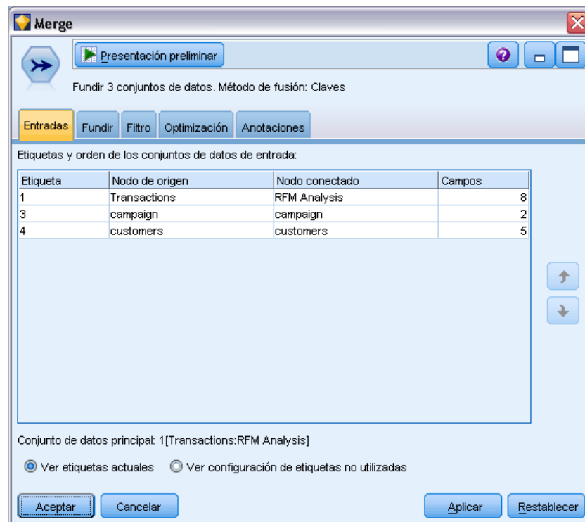
Figura 3-19 Uso de la pestaña Entradas para especificar etiquetas y orden de entrada
