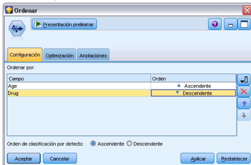
Figura 3-10 Cuadro de diálogo del nodo Ordenar
