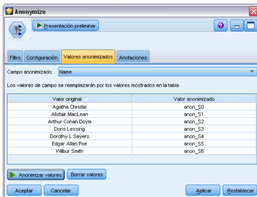
Figura 4-59 Anonimización de valores de campo
