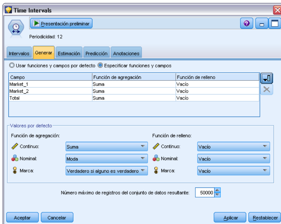
Figura 4-85 nodo Intervalos de tiempo, pestaña Generar
