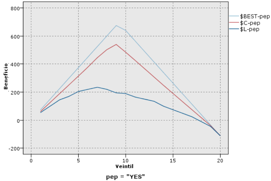
Figura 5-61 Gráfico de beneficios (acumulado) con mejor línea
