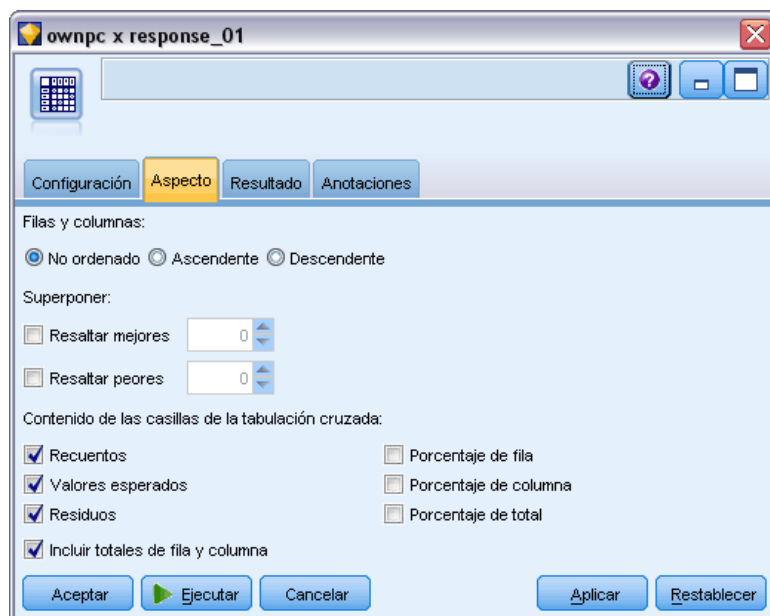
Figura 6-10 Nodo Matriz: Pestaña Aspecto
