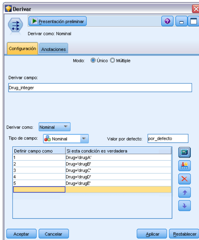
Figura 4-52 Nueva codificación de valores de cadena
