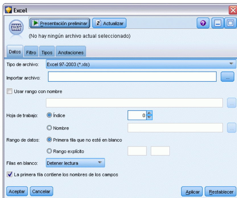
Figura 2-25 Nodo de origen de Excel
