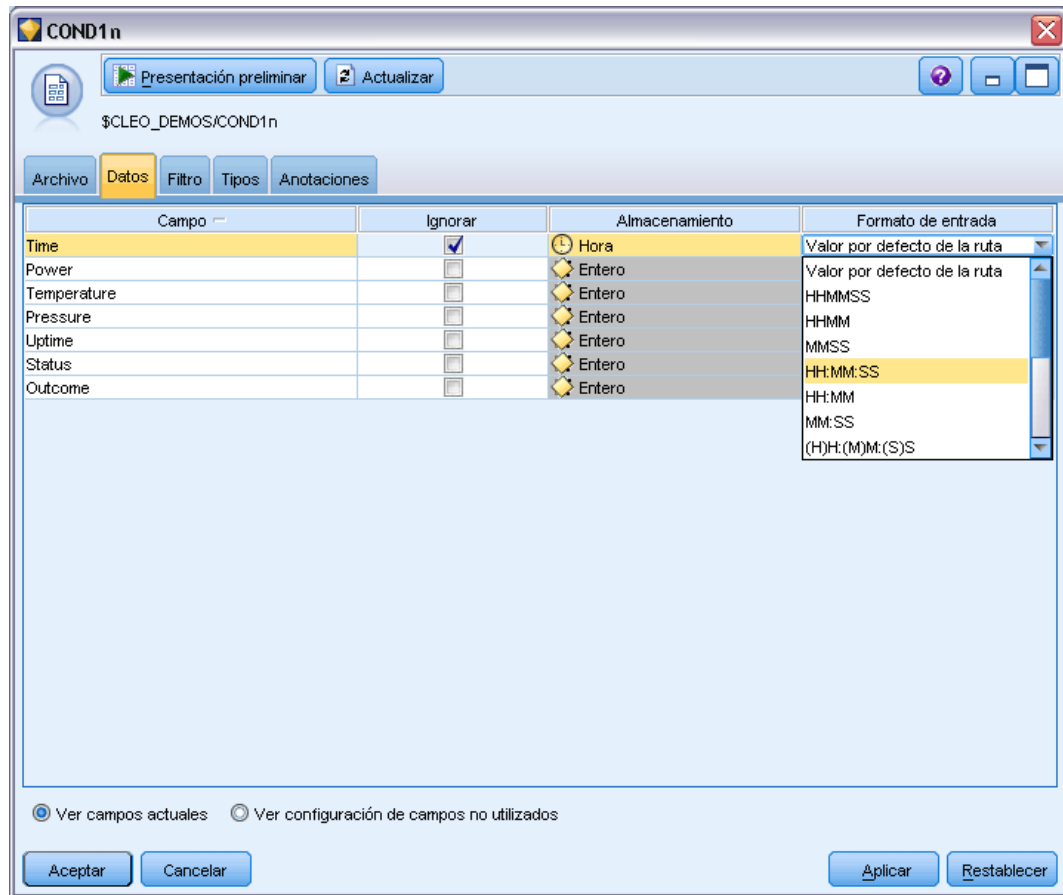
Figura 2-13 Sustitución del tipo de almacenamiento y asignación de formato al campo en la importación
