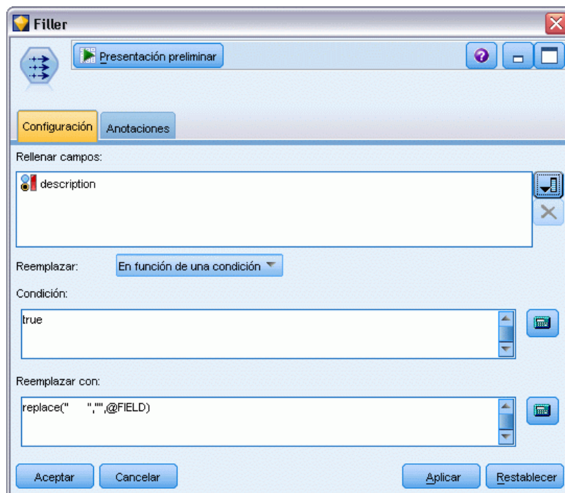
Figura 2-29 Nodo Rellenar con los ajustes para eliminar espacios
