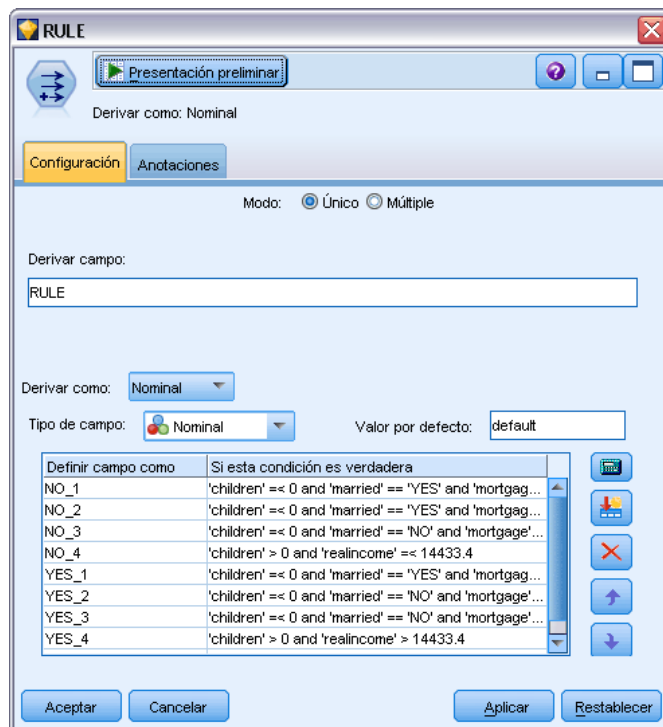
Figura 4-48 Uso de un nodo de derivación como conjunto
