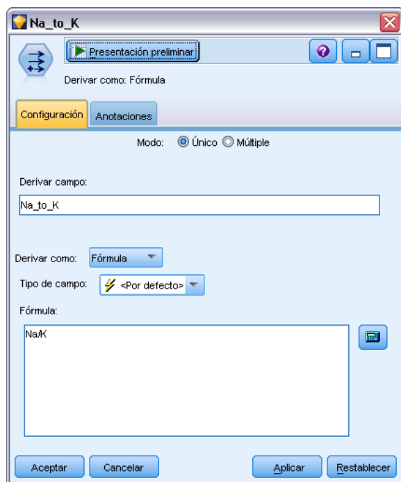
Figura 4-42 Cuadro de diálogo del nodo Derivar
