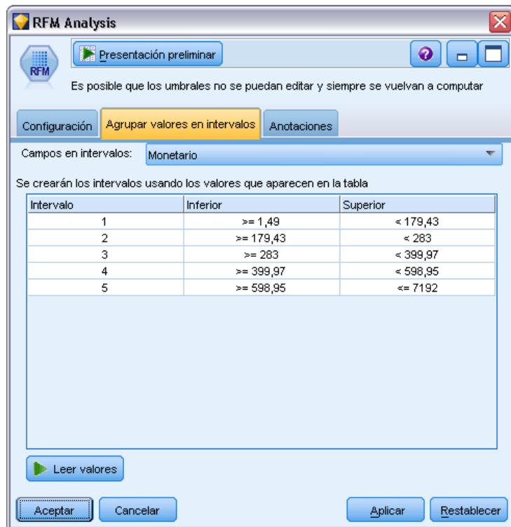
Figura 4-73 Configuración de los valores de intervalo de Análisis de RFM
