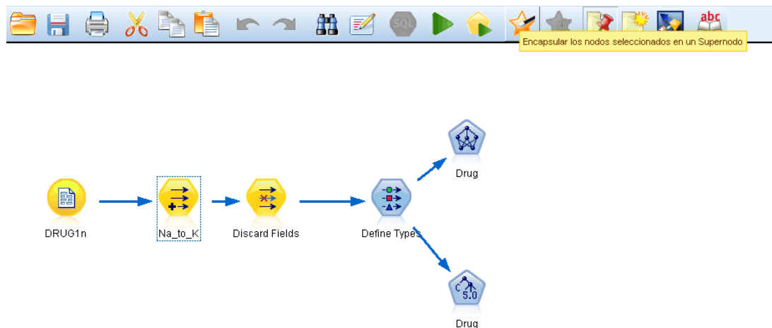
Figura 9-4 Creación de un supernodo mediante la selección múltiple
