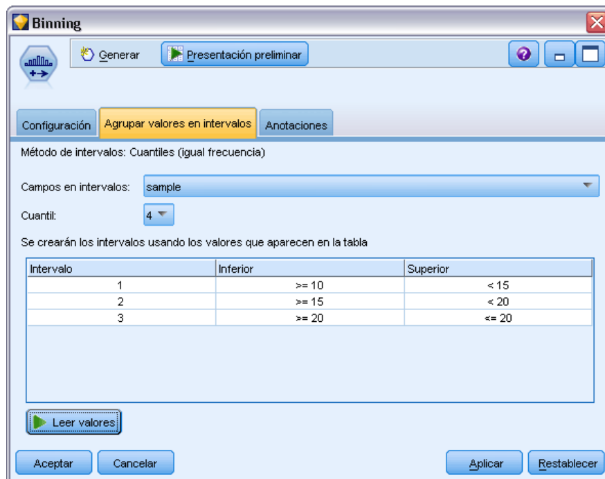
Figura 4-66 Umbrales para intervalos generados
