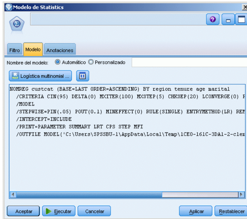
Figura 8-5 Sintaxis mostrada en la pestaña Modelo
