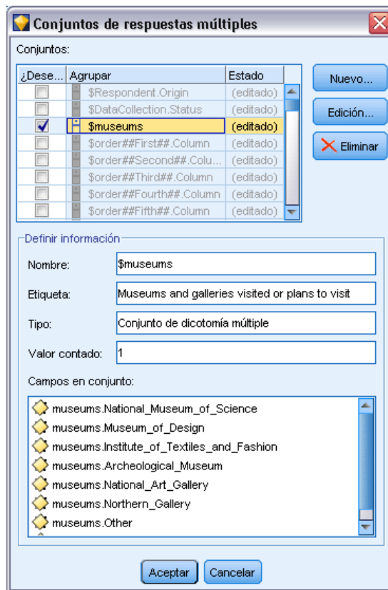
Figura 4-36 Cuadro de diálogo Conjuntos de respuestas múltiples
