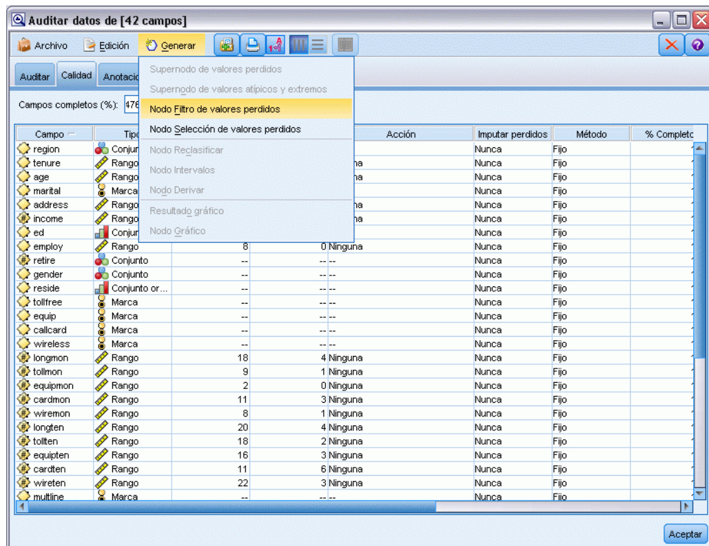
Figura 6-18 Creación de un nodo Filtro de valores perdidos
