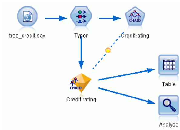
Figure 4-16 Ajout d'un noeud Analyse
