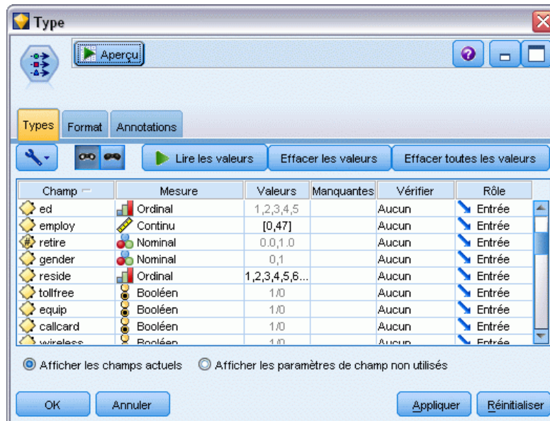
Figure 8-3 Définition des niveaux de mesure
