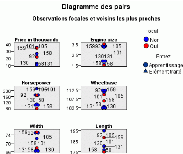
Figure 29-11 Comparaison des caractéristiques dans le diagramme des pairs
