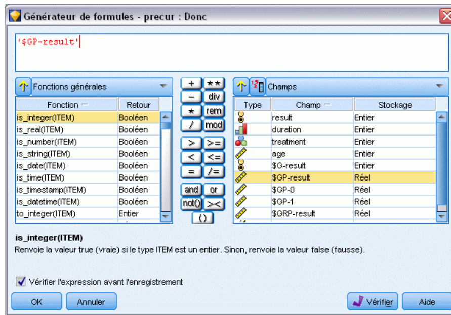
Figure 23-12 Noeud Calculer : Générateur de formules pour la formule Then
