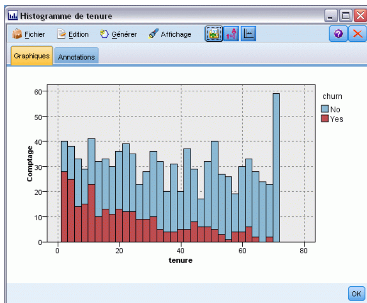
Figure 8-8 Histogramme de durée d'affectation
