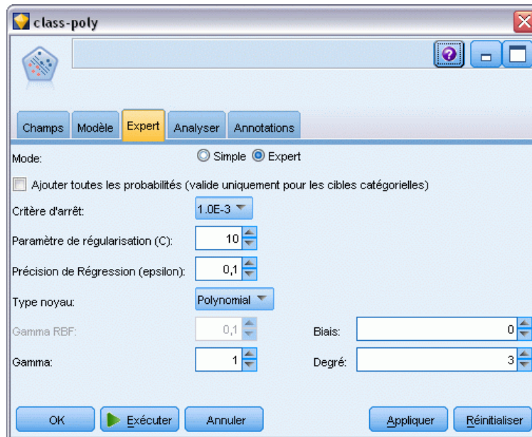
Figure 26-10 Paramètres de l'onglet Expert pour polynomial
