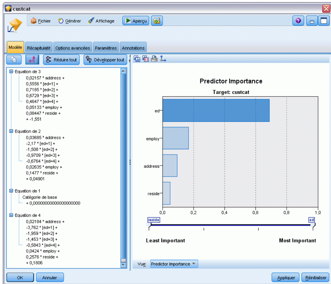
Figure 13-7 Navigation dans les résultats du modèle
