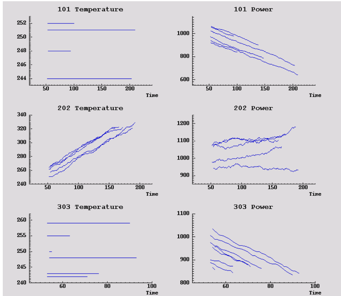
Figure 21-2 Température et puissance dans le temps
