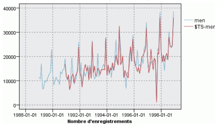
Figure 16-17 Modèle ARIMA avec variables indépendantes spécifiées
