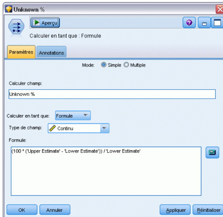
Figure 27-31 Noeud Calculer : onglet Paramètres
