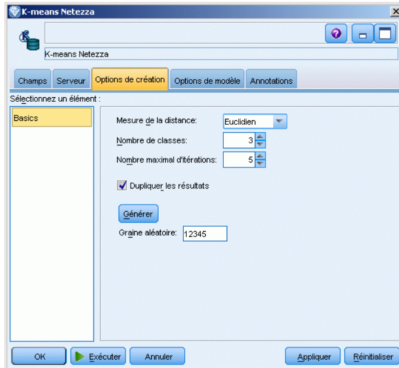
Figure 6-9 Options de création K-Means
