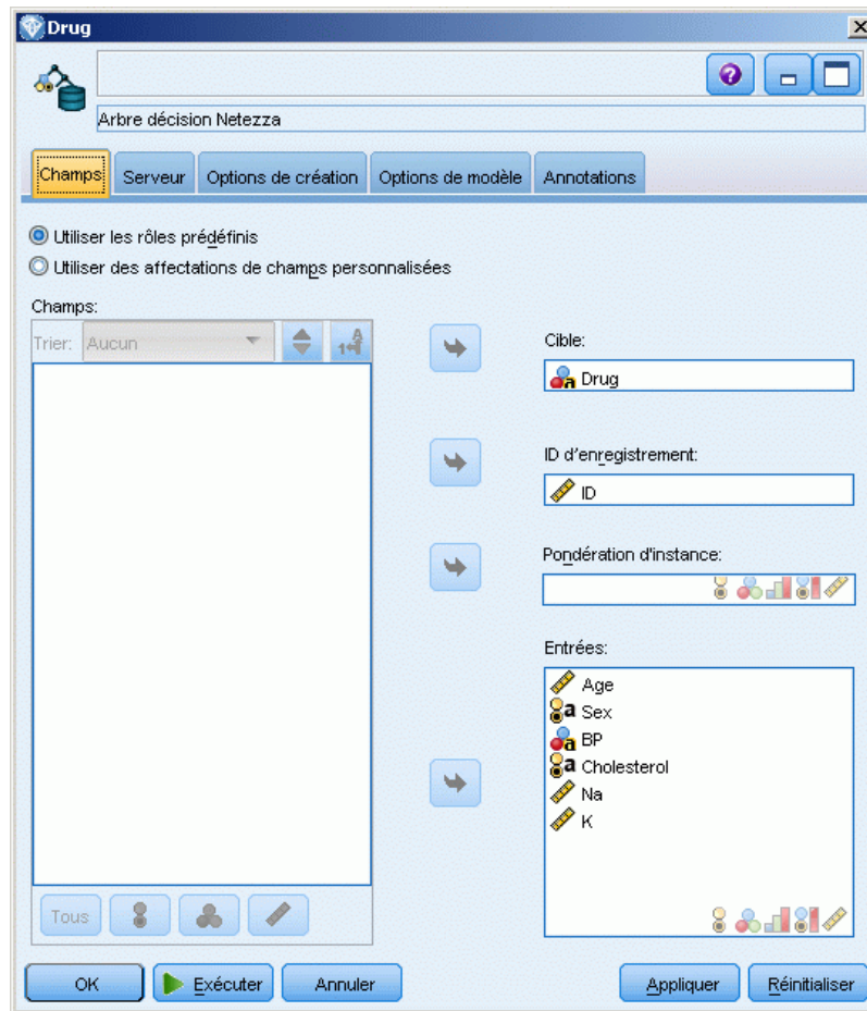
Figure 6-4 Options du champ Arbre décision
