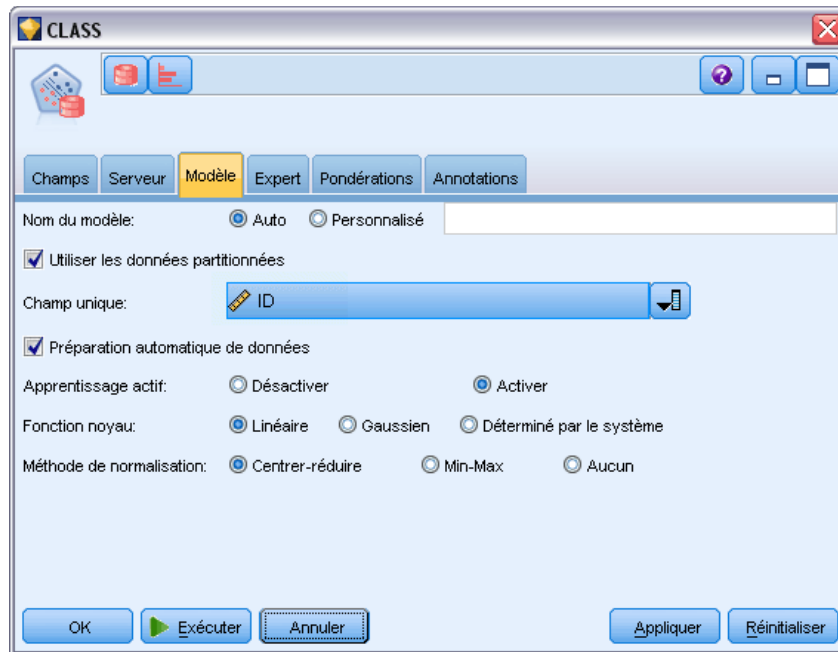
Figure 4-42 Options de modèle Oracle SVM
