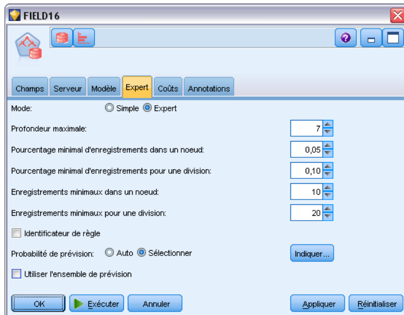
Figure 4-17 Arbre de décision - Options expert
