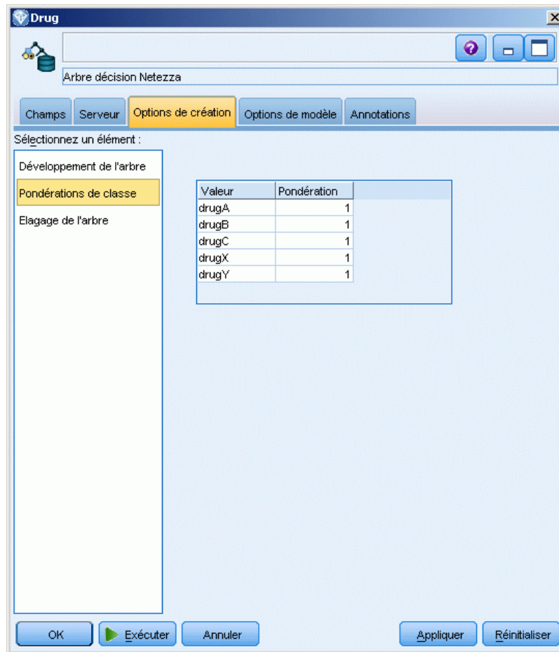
Figure 6-6 Options de pondération de classe de l'arbre décision
