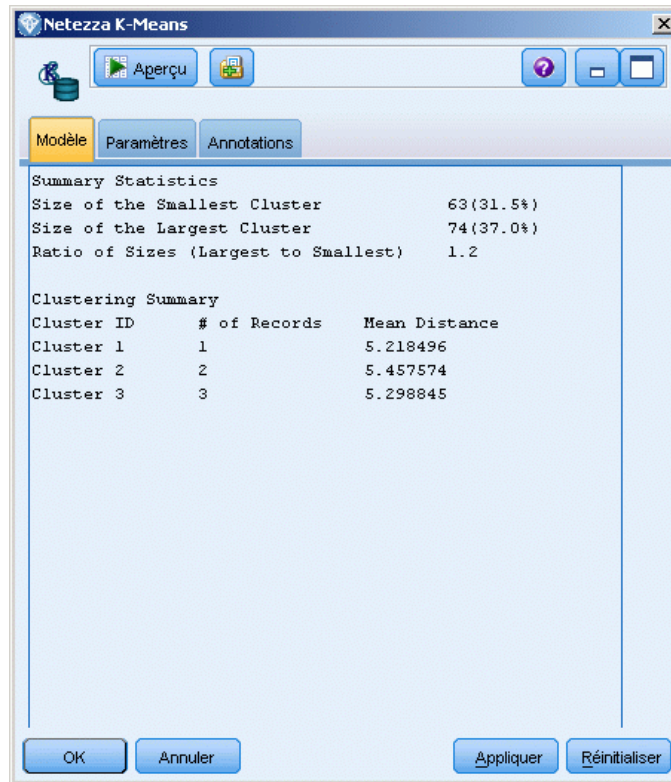
Figure 6-12 Sortie du modèle K-means
