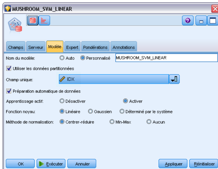
Figure 4-10 Options des modèles SVM
