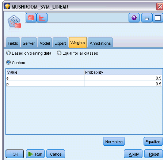
Figure 4-12 Options de pondérations SVM
