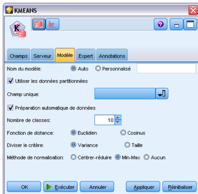
Figure 4-20 Options du modèle k-Means
