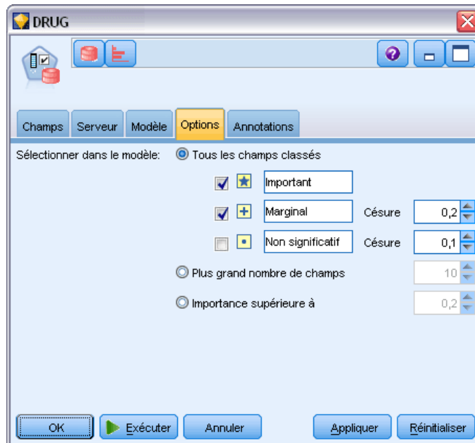
Figure 4-30 IA - Options de sélection
