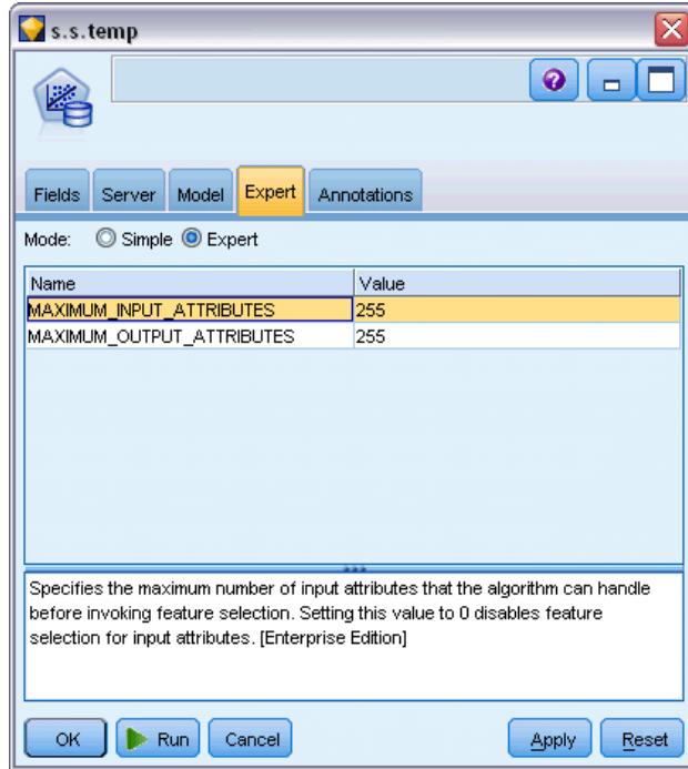
Figure 3-10 Régression linéaire MS - Options expert
