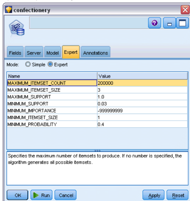
Figure 3-13 Options expert des règles d'association MS
