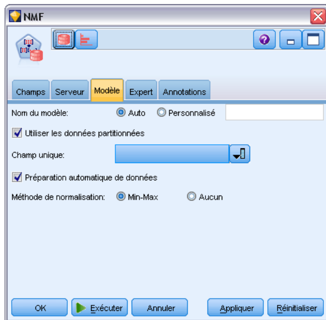
Figure 4-22 Options du modèle NMF
