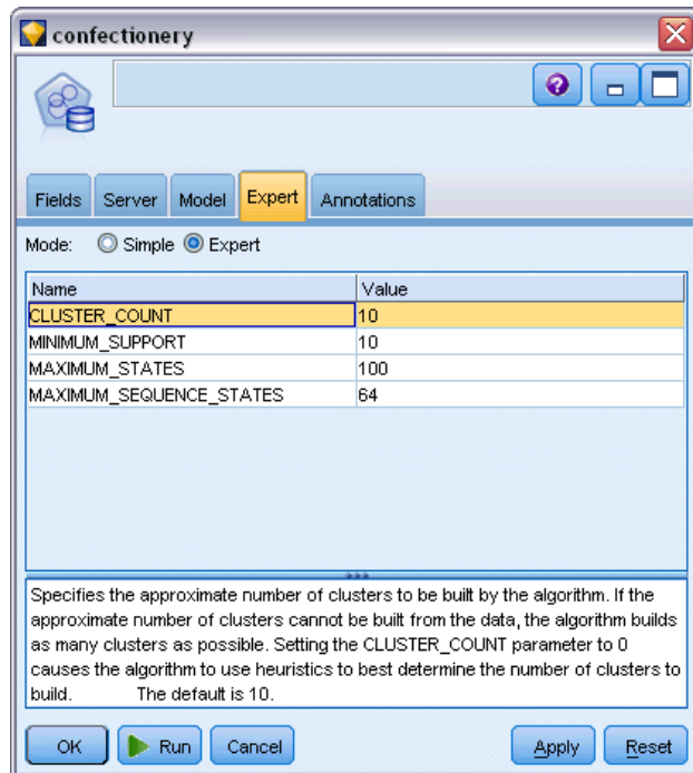
Figure 3-18 Spécification des options expert de la classification de séquences MS
