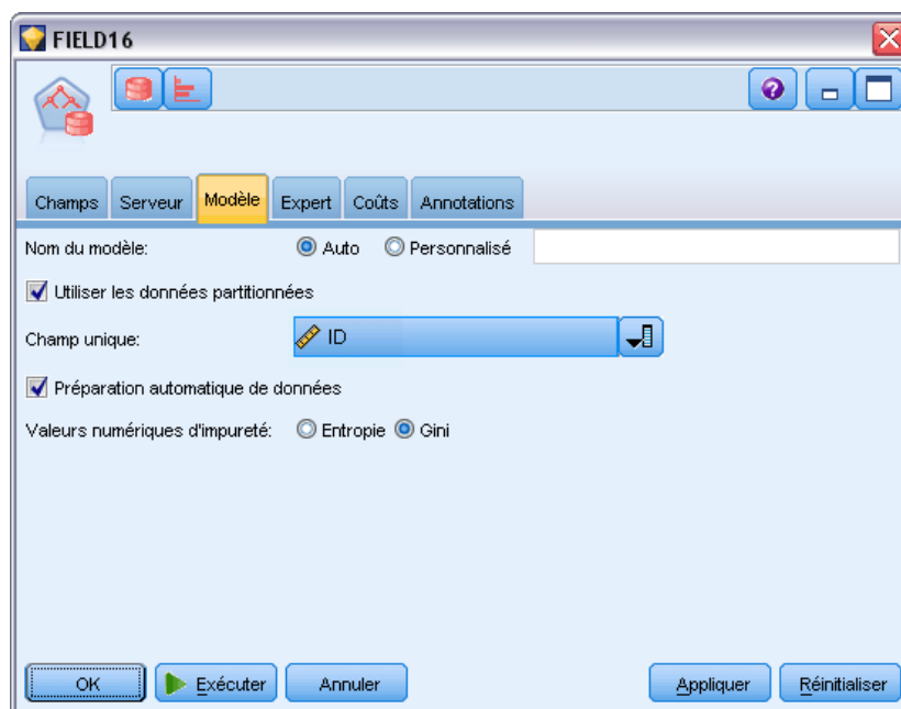
Figure 4-16 Options du modèle Arbre décision
