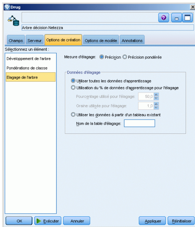
Figure 6-7 Options d'élagage de l'arbre décision
