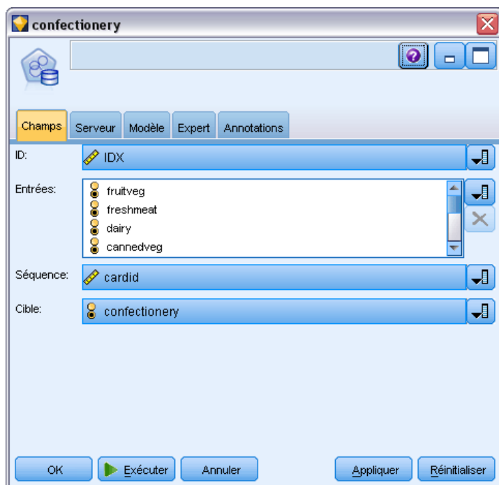
Figure 3-17 Spécification des champs pour la classification de séquences MS
