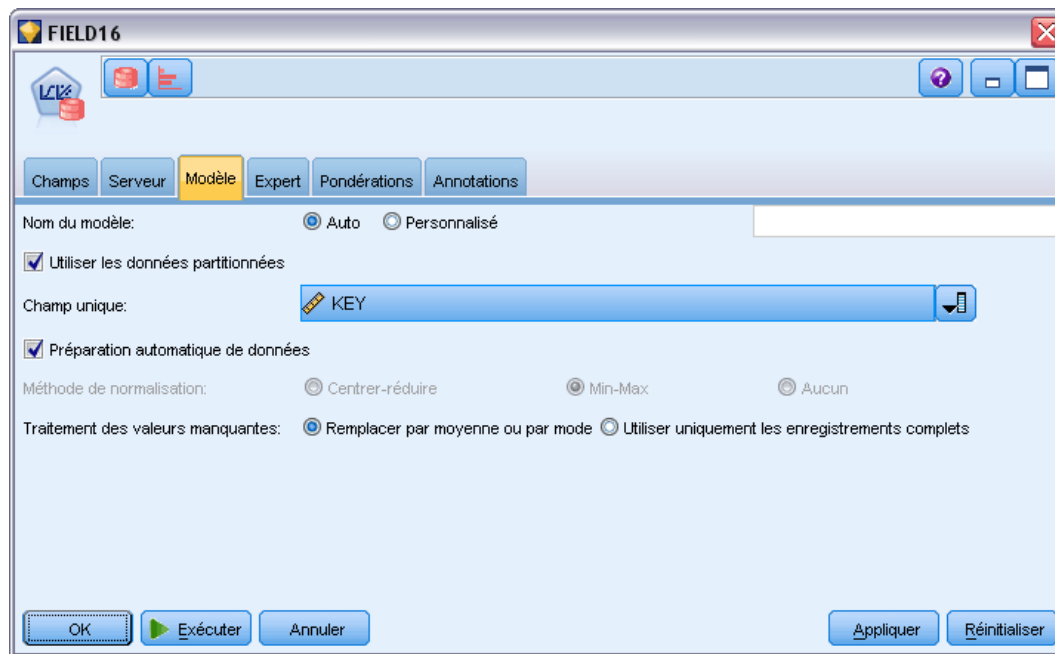
Figure 4-13 options de modèle MLG
