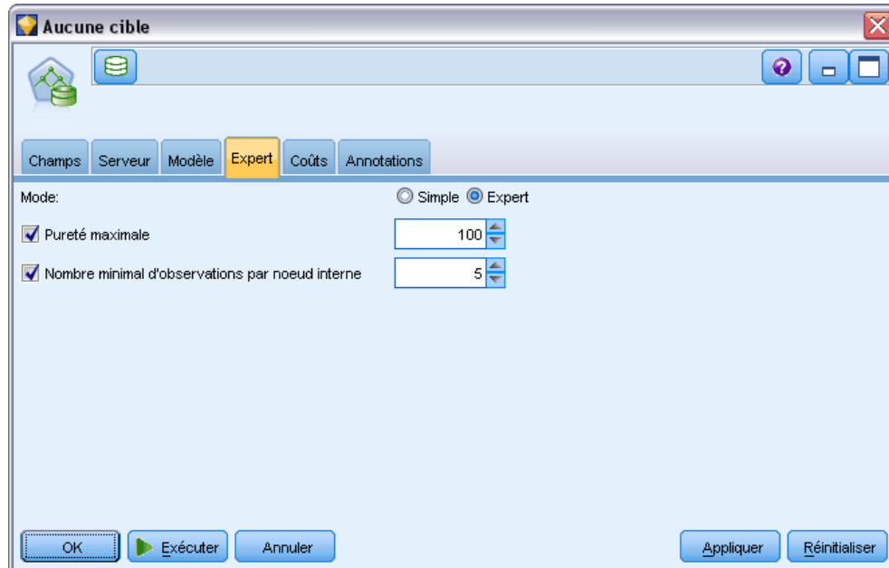
Figure 5-12 Noeud Arbre décision ISW, onglet Expert
