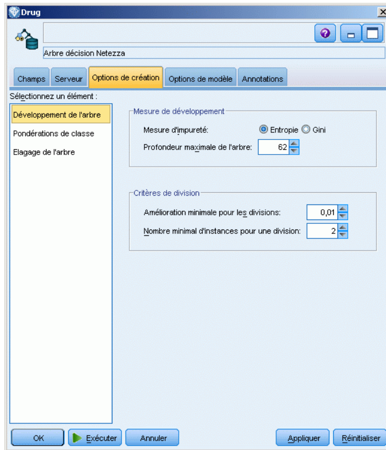
Figure 6-5 Options de création de l'arbre de décision pour le développement de l'arbre
