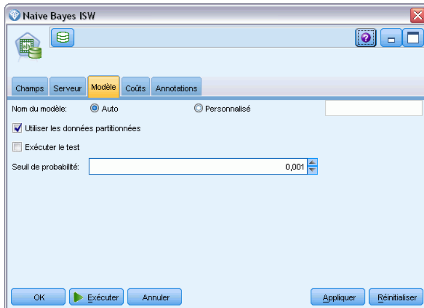
Figure 5-27 Onglet Modèle du noeud Naive Bayes ISW
