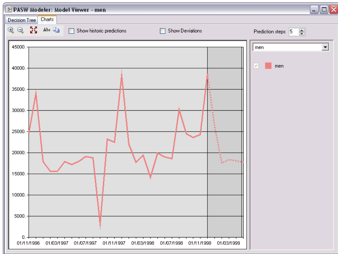
Figure 3-24 Visualiseur de séries temporelles MS avec des valeurs historiques (ligne pleine) et des valeurs prédites futures (ligne en pointillés)
