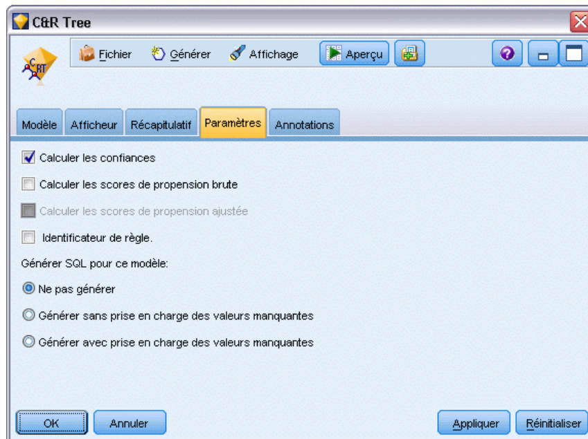
Figure 6-40 Paramètres de nugget du modèle d'arbre décision
