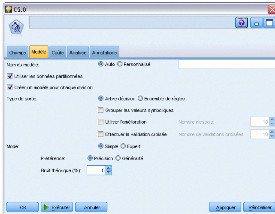
Figure 6-35 Noeud C5.0 - Options du modèle
