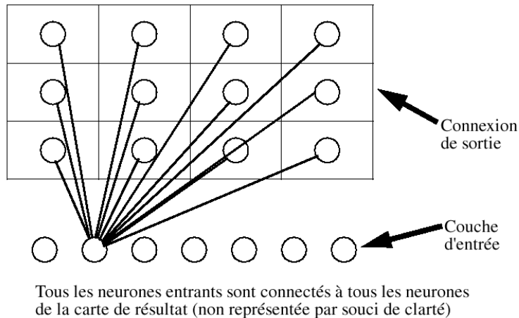
Figure 11-2 Structure d'un réseau Kohonen
