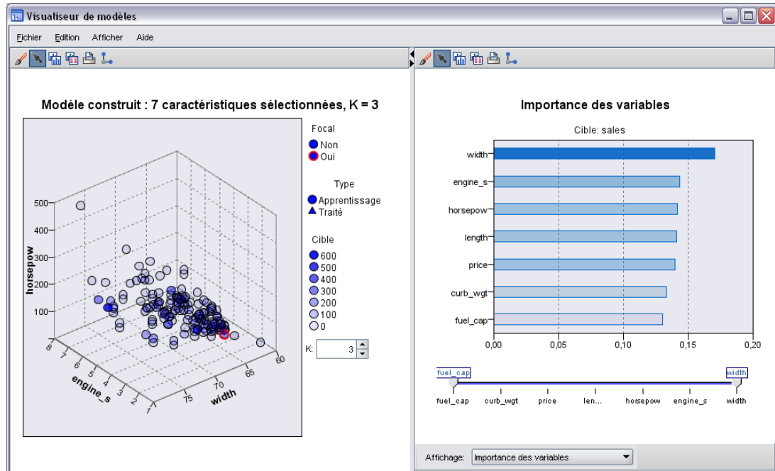
Figure 16-8 Vue du modèle de l'analyse du voisin le plus proche
