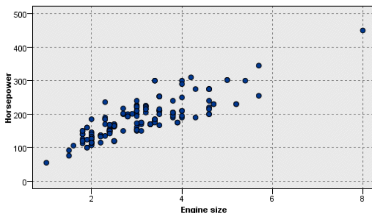
Figure 10-1 Diagramme de régression linéaire simple
