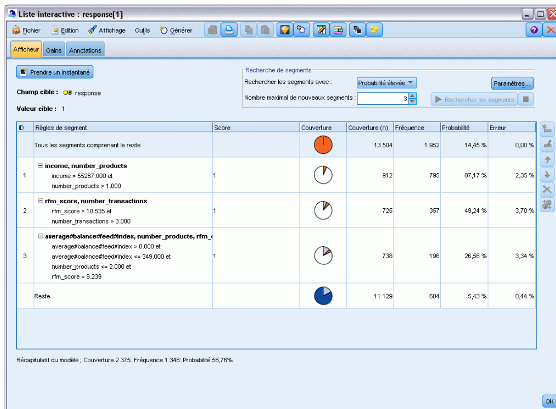
Figure 9-10 Afficheur interactif Liste de décision
