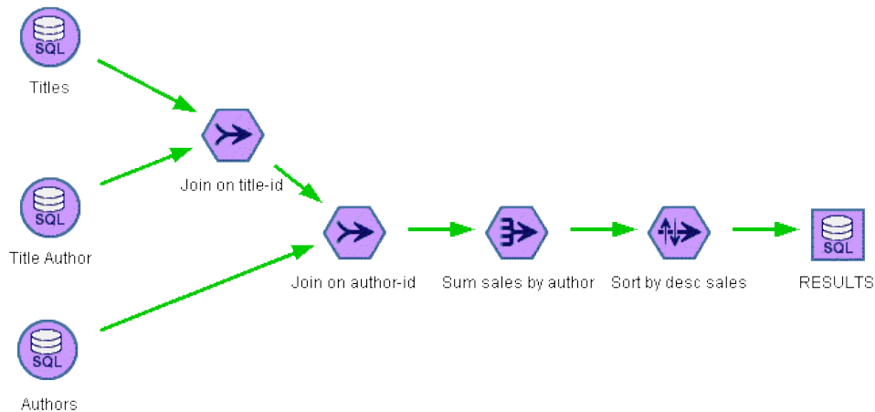
Figura 6-2 Stream intero eseguito nel database
