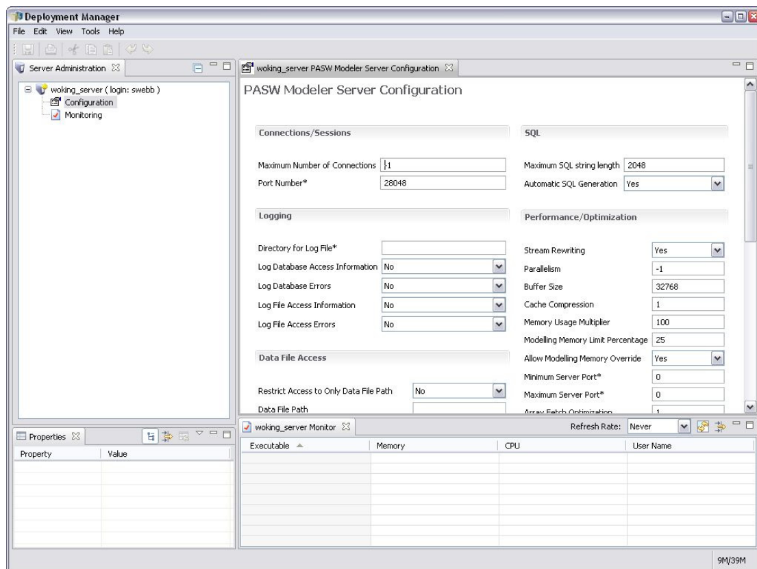
Figura 4-1 Interfaccia di Modeler Administration Console
