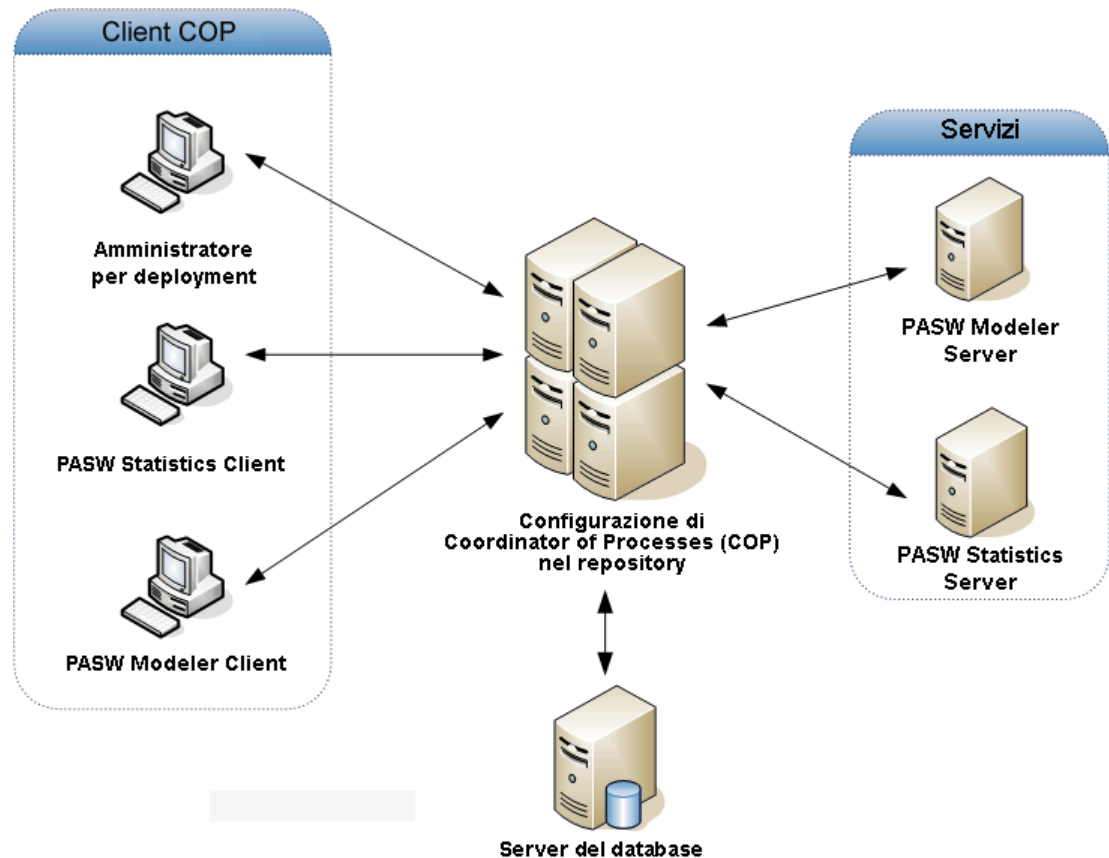
Figura D-1 Architettura di Coordinator of Processes
