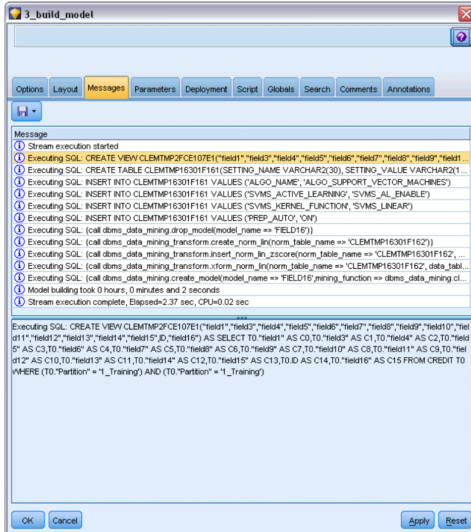
Figura 6-4 SQL generato visualizzato nel registro dei messaggi
