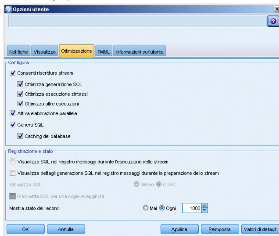
Figura 5-1 Finestra di dialogo Opzioni utente, scheda Ottimizzazione
