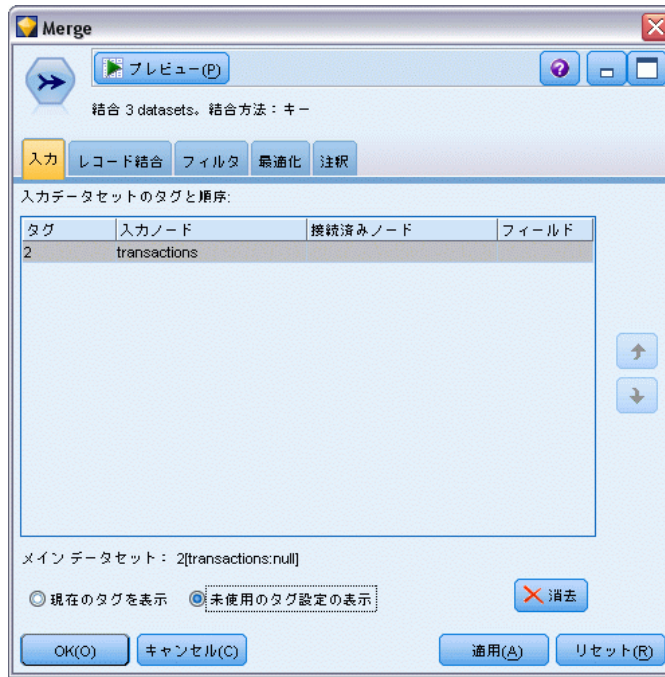
図 3-20 レコード結合ノードからの未使用のタグの削除
