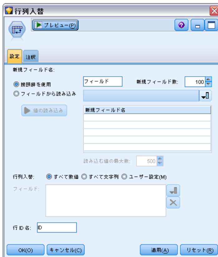
図 4-77 行列入替ノードの [設定] タブ
