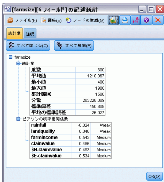
図 6-38 記述統計量出力ブラウザ
