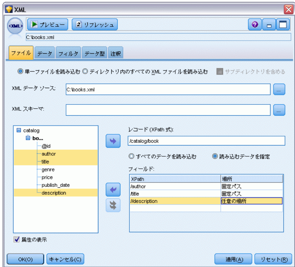
図 2-26 XML データのインポート
