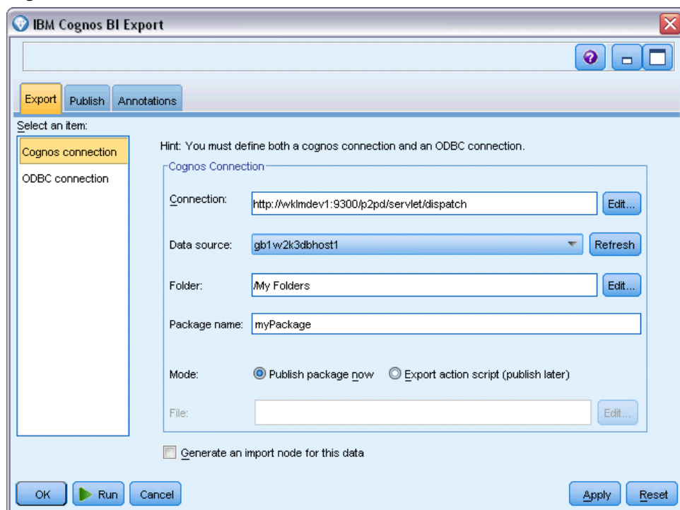
図 7-9 Cognos データのエクスポート
