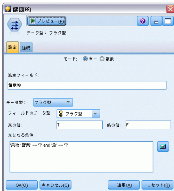
図 4-46 フラグ型フィールドの作成
