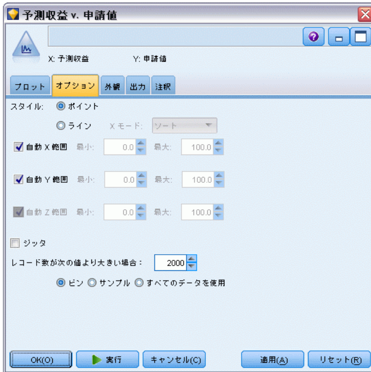
図 5-20 散布図ノードの [オプション] タブの設定
