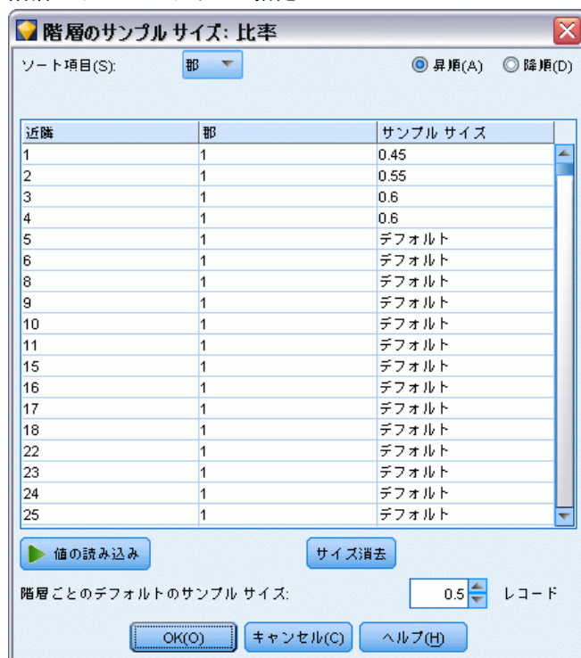
図 3-6 階層のサンプル サイズの指定
