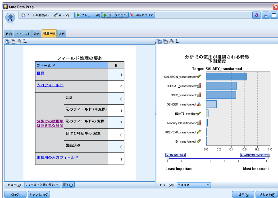
図 4-10 自動データ準備の [分析] タブ
