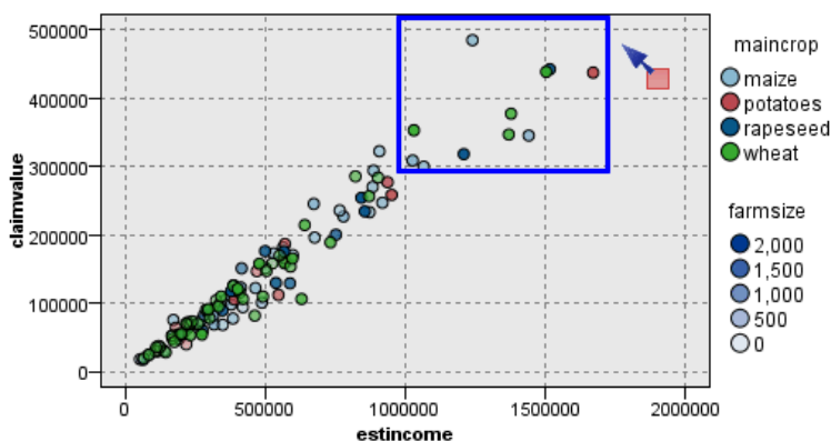
図 5-76 申請値の高い領域の定義
