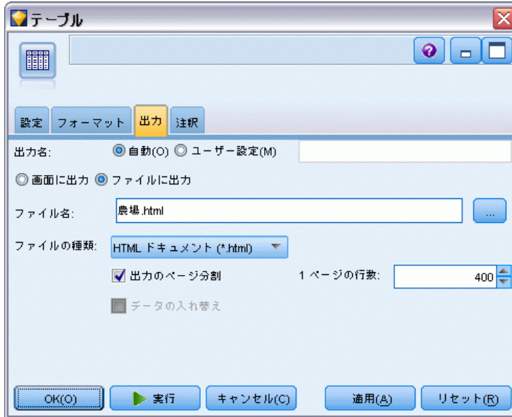
図 6-6 出力ノードの [出力] タブ
