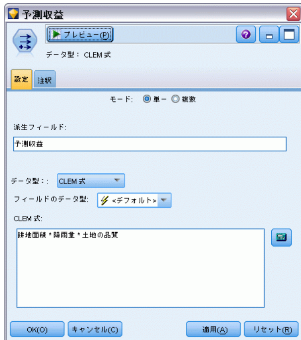
図 4-45 フィールド作成ノード（CLEM 式型）のオプションの設定
