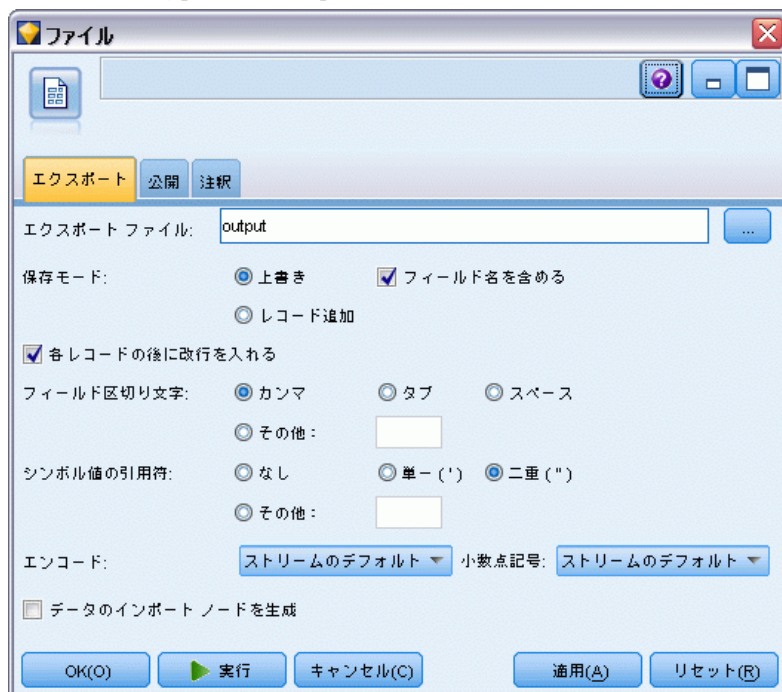
図 7-7 ファイルノード、[エクスポート] タブ
