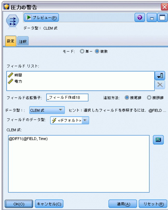
図 4-43 複数フィールドの作成
