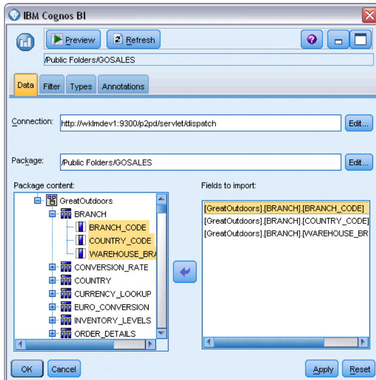
図 2-21 Cognos データのインポート
