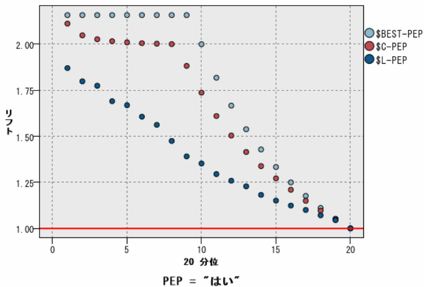
図 5-59 ポイントおよびベストラインを使用するリフト グラフ (累積)
