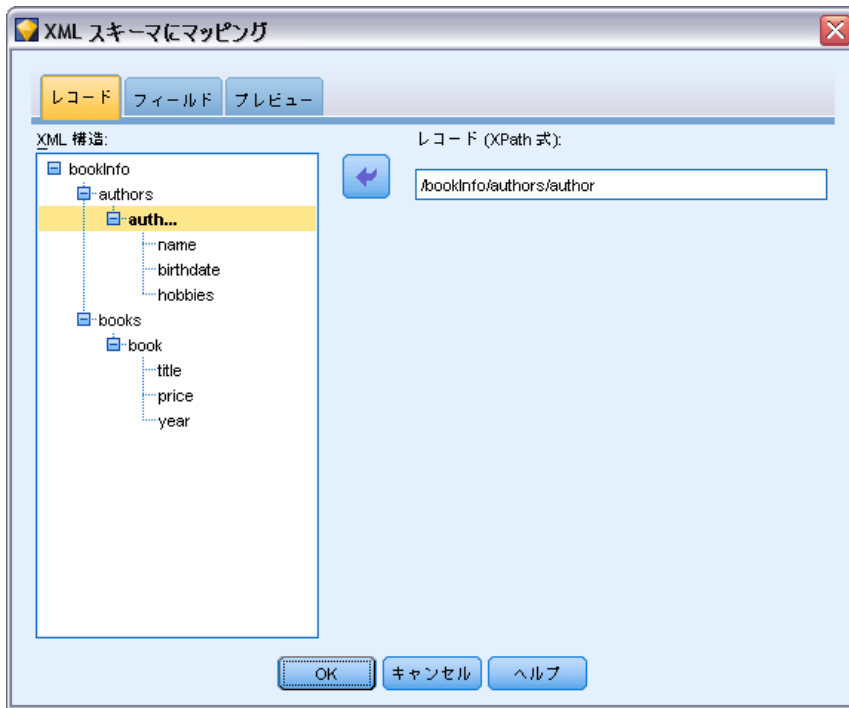
図 7-14 XML マッピング レコード
