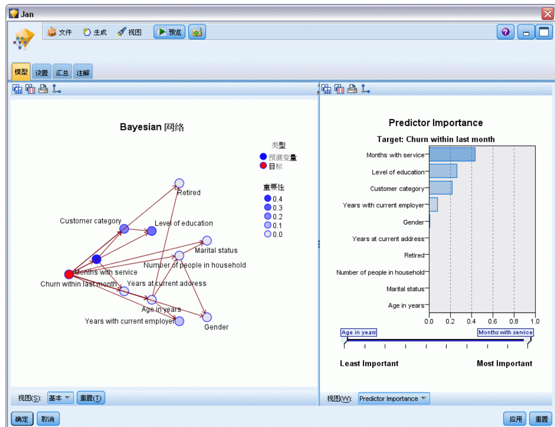
图片 19-10 贝叶斯网络模型显示了预测变量重要性
