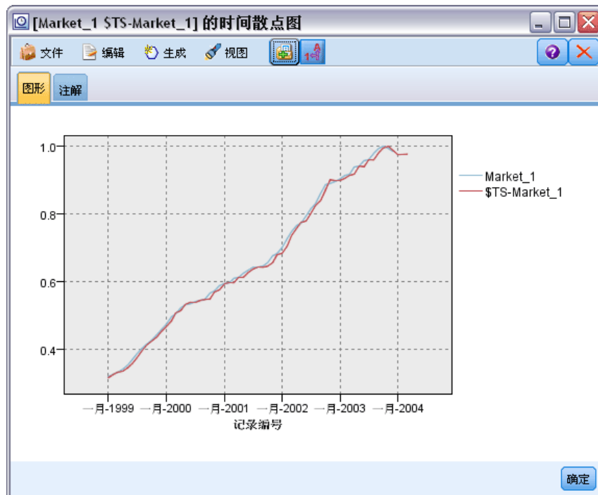
图片 15-19 Market_1 的实际数据和预测数据的时间散点图
