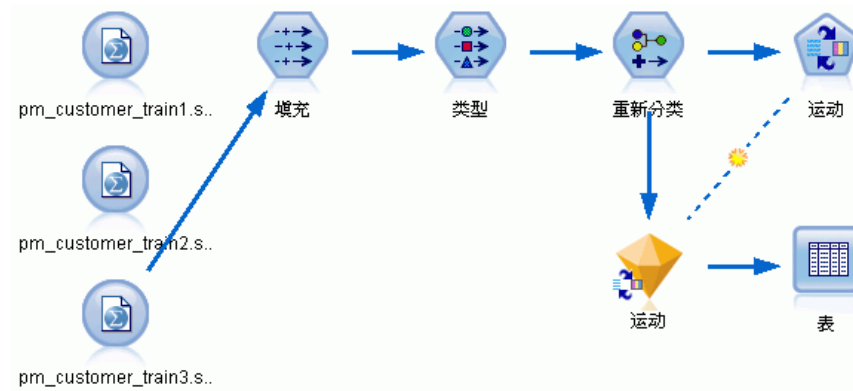
图片 17-11 将第三个数据源附加到 SLRM 流
