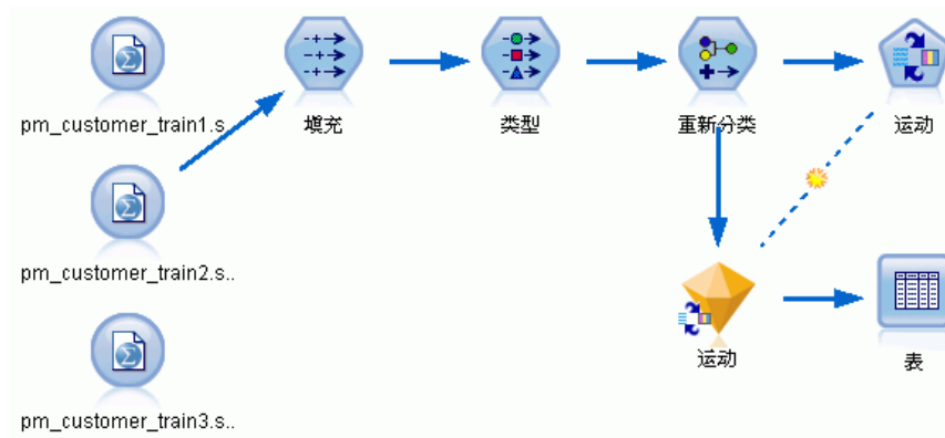
图片 17-9 将第二个数据源附加到 SLRM 流
