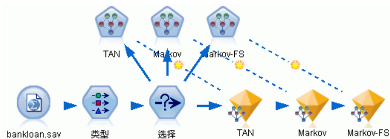
图片 18-8 对齐流中的模型块
