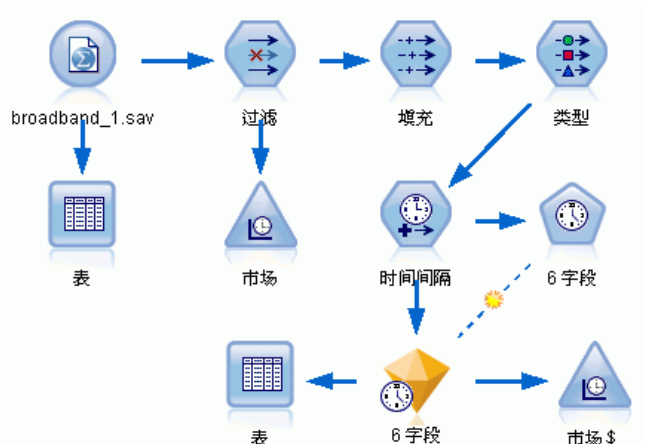
图片 15-1 显示时间序列建模的样本流
