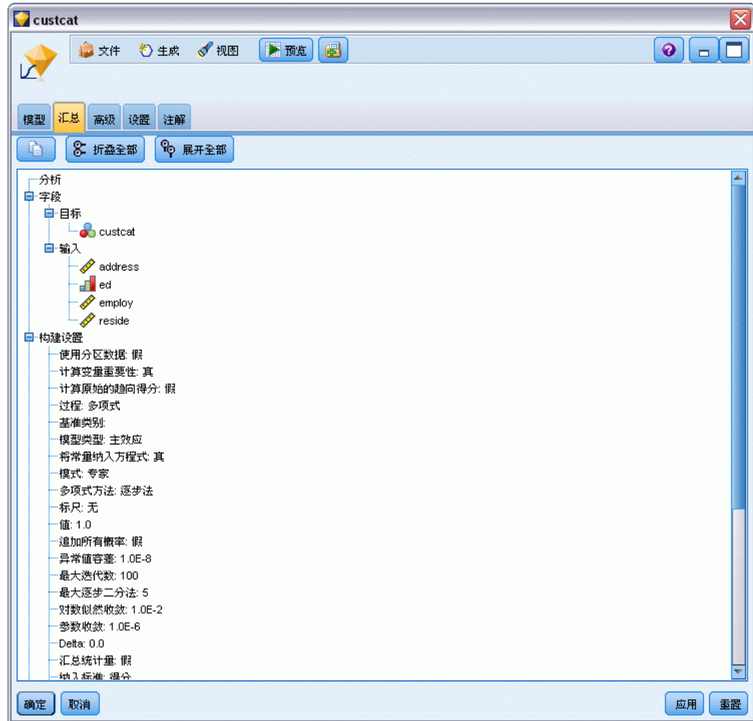
图片 13-8 显示目标和输入字段的模型汇总
