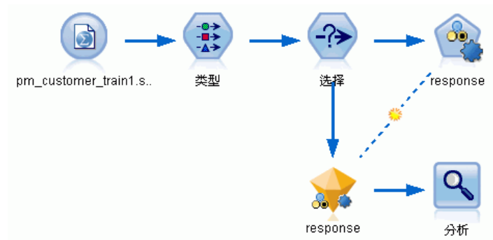
图片 5-1 自动分类器样本流
