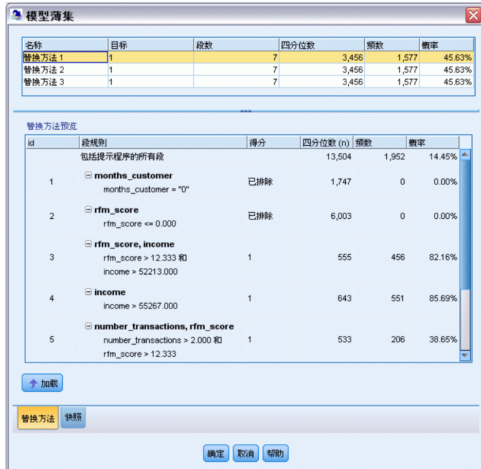
图片 12-19 组合模型的替代模型
