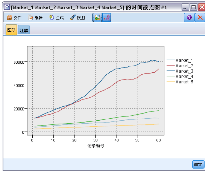
图片 15-7 多个字段的时间散点图
