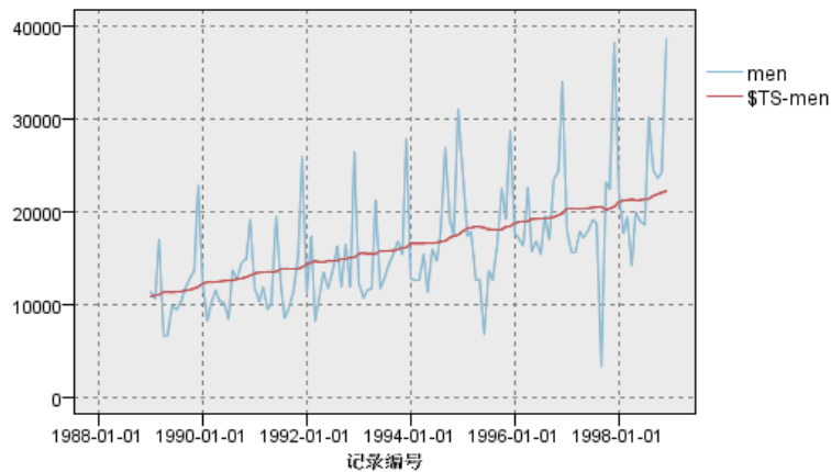
图片 16-10 Holt 线性趋势模型
