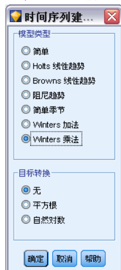
图片 16-11 选择 Winters 模型
