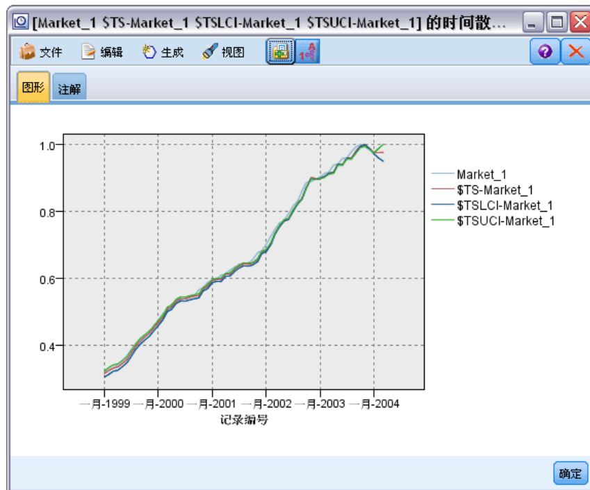
图片 15-21 添加了置信区间的时间散点图
