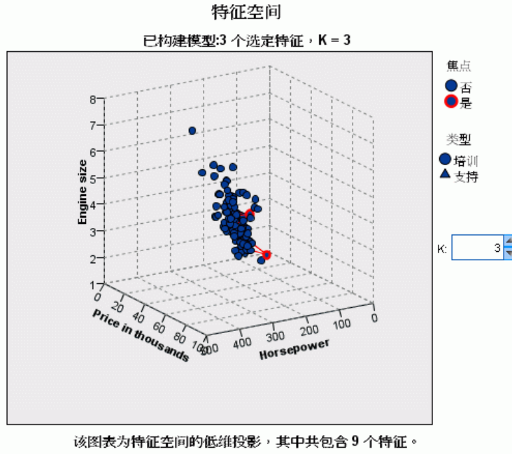
图片 29-8 预测变量空间图表
