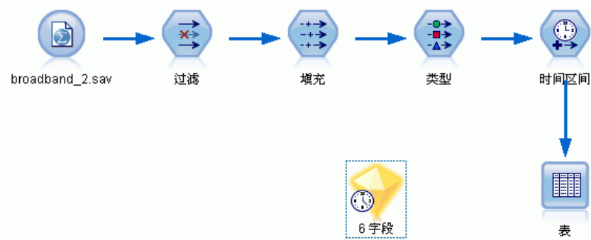
图片 15-25 添加模型块
