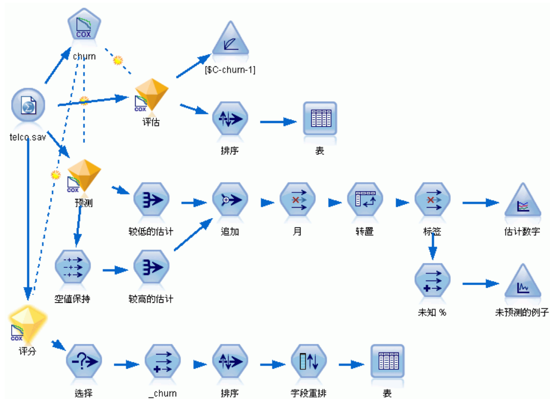
图片 27-1 分析流失时间的样本流
