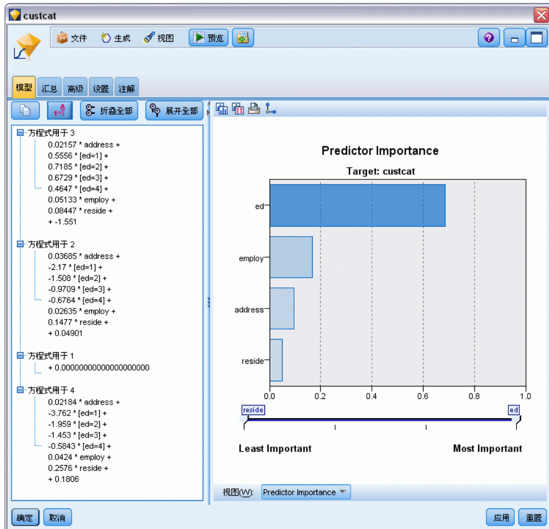
图片 13-7 浏览模型结果
