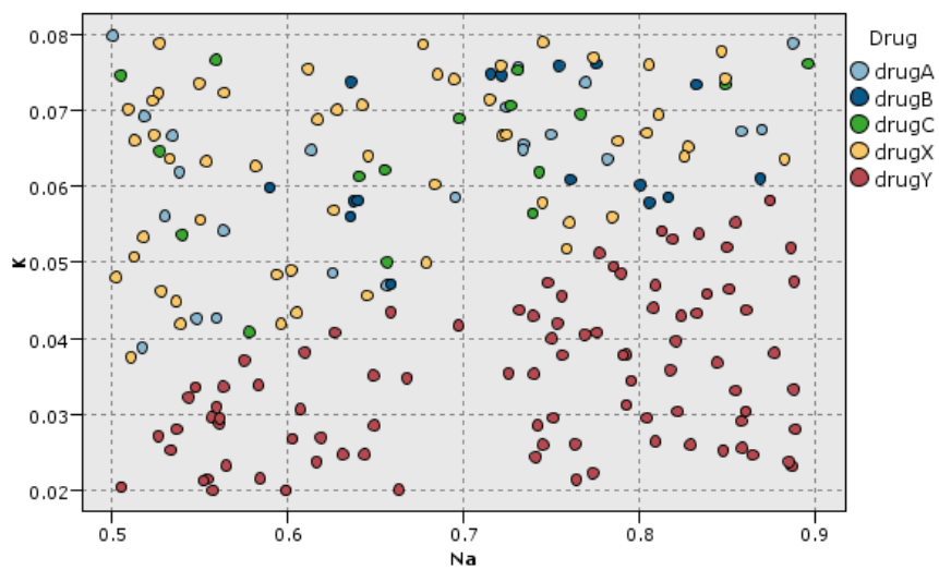
图片 9-11 药品分布散点图
