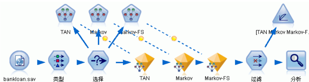
图片 18-1 贝叶斯网络样本流
