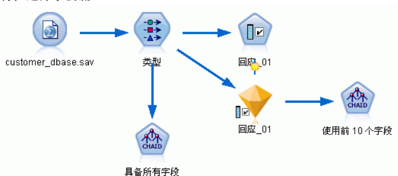
图片 10-1 特征选择示例流
