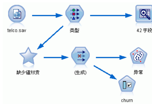
图片 8-13 具有缺失值超节点的流
