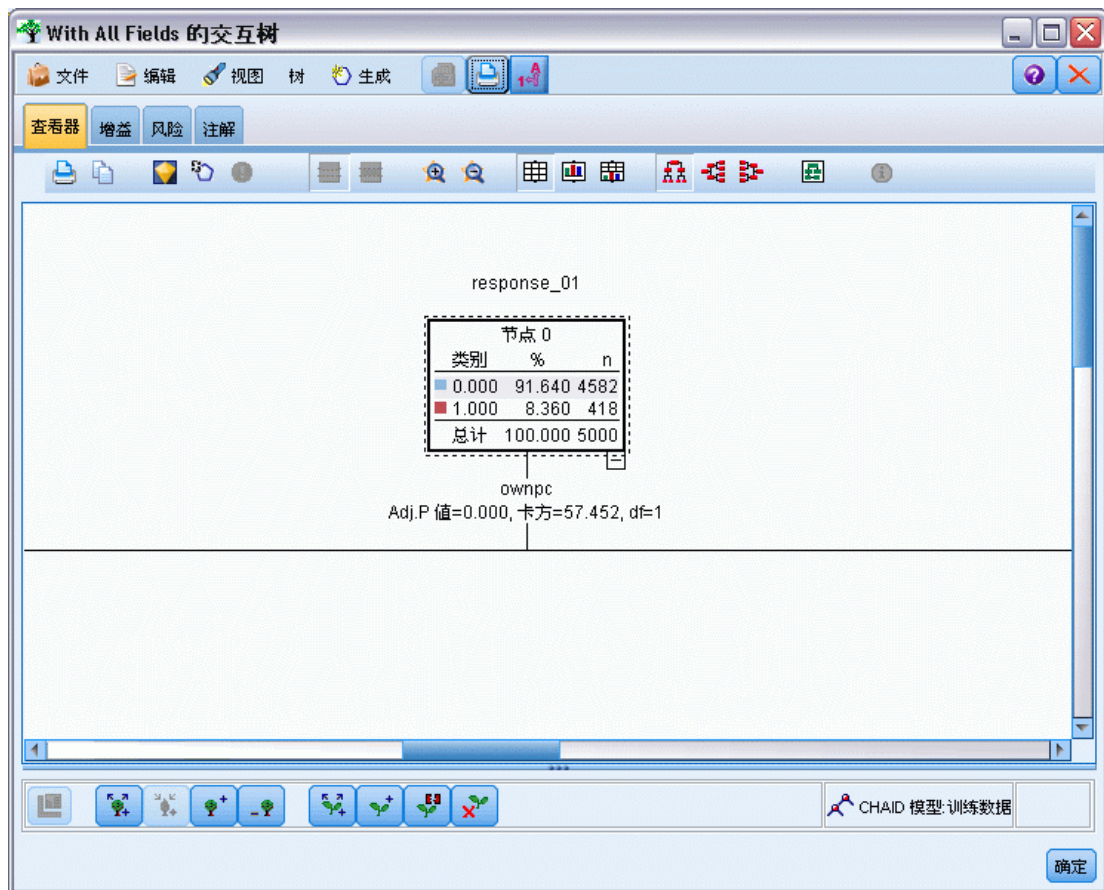
图片 10-4 在树构建器中生成树
