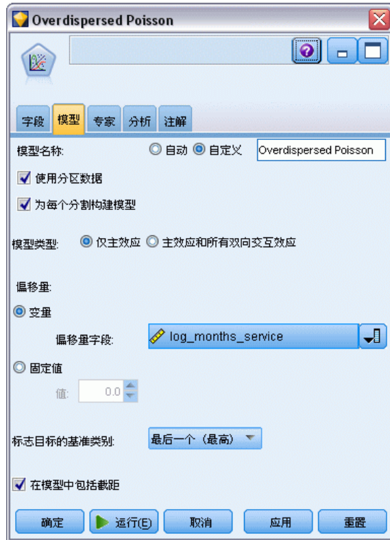
图片 24-4 选择模型选项
