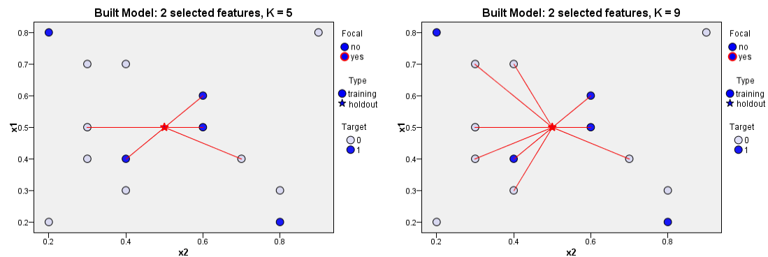
图片 29-1 更改 k 对分类的影响
