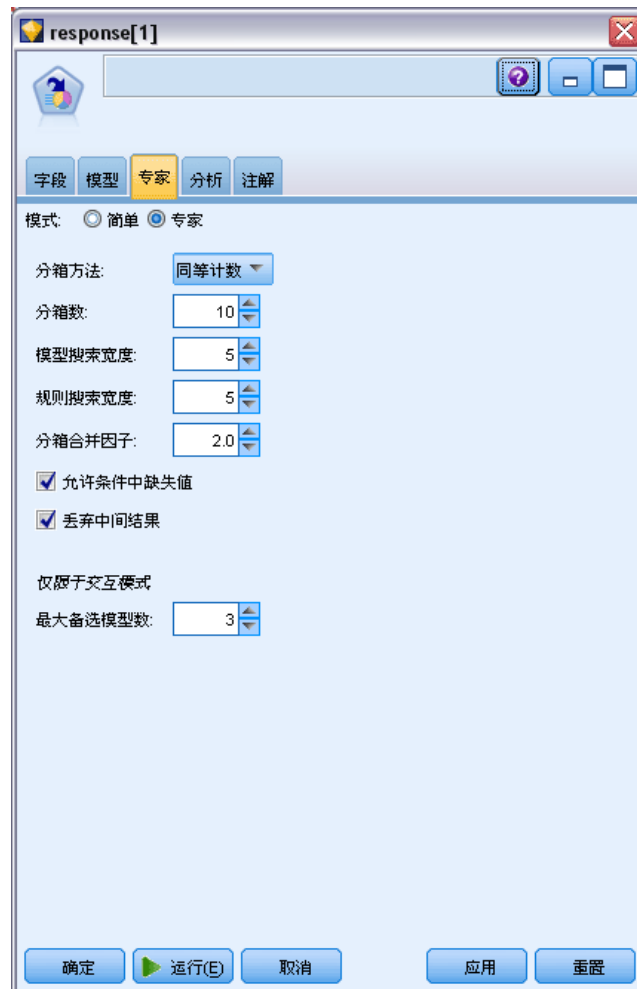
图片 12-7 决策列表节点，“专家”选项卡
