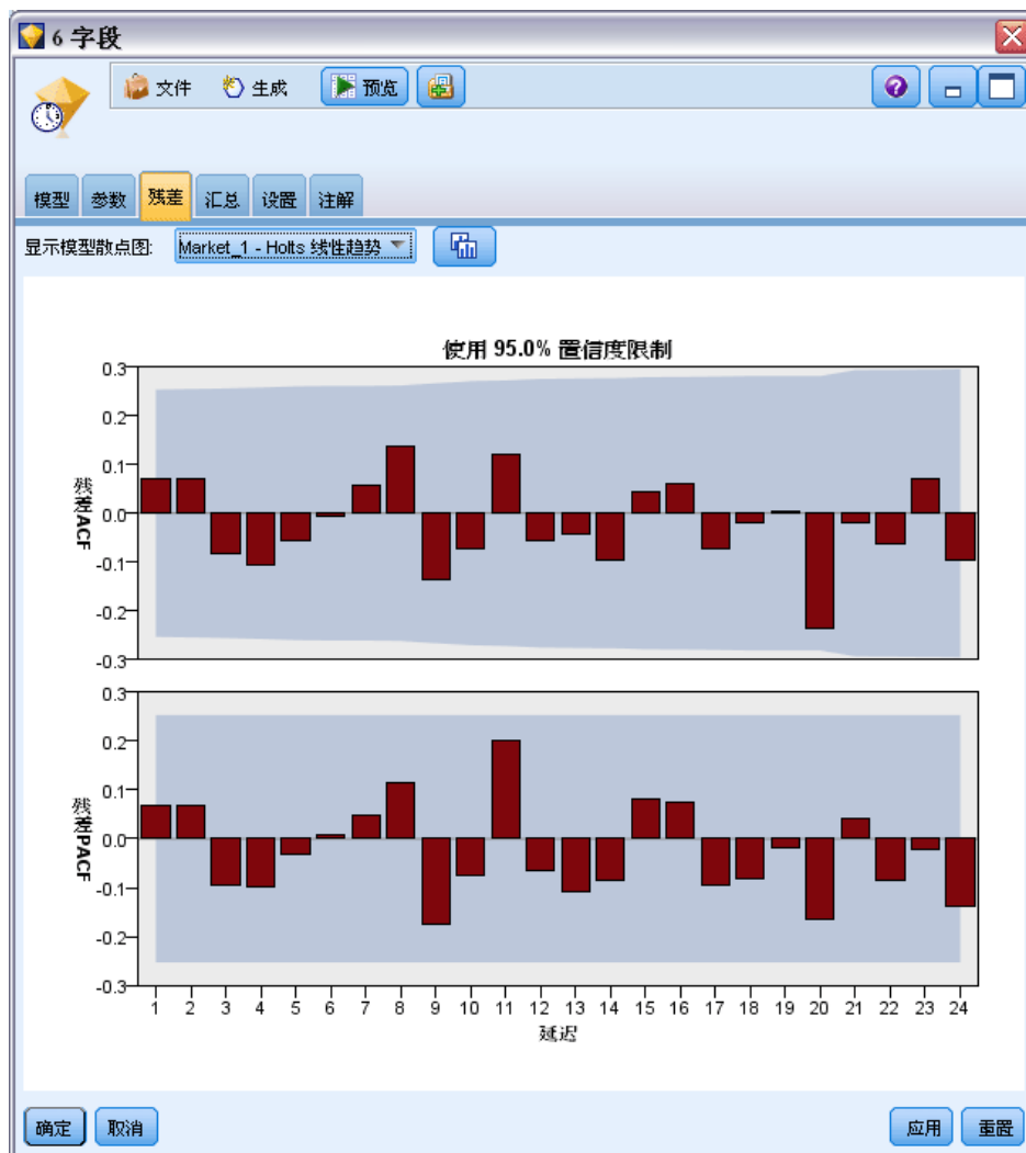
图片 15-17 市场的 ACF 值和 PACF 值
