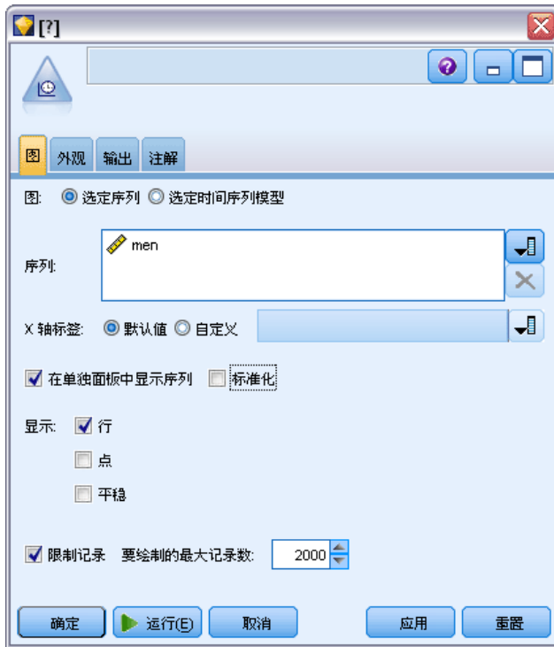
图片 16-4 绘制时间序列
