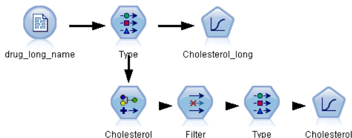
图片 11-1 显示了对二项 logistic 回归的字符串重新分类的样本流
