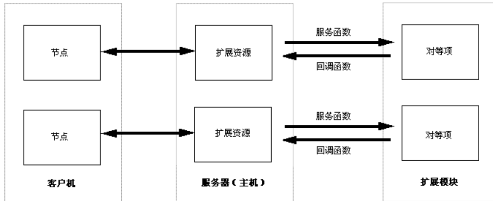
图片 9-1 CLEF API 体系结构
