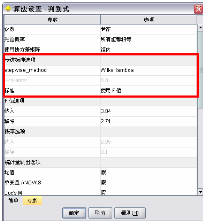
图片 5-9 专家设置被禁用
