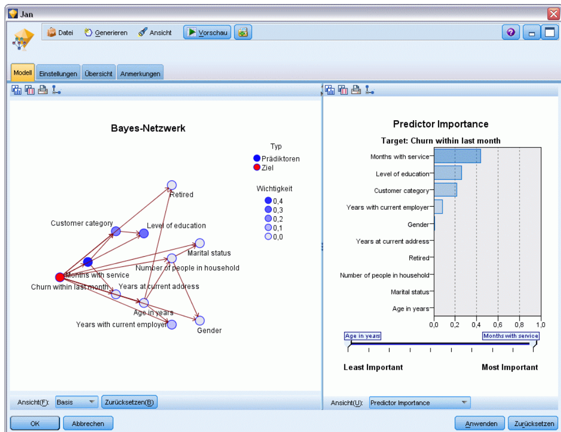
Abbildung 18-10 Bayes-Netzwerk-Modell mit Bedeutsamkeit der Prädiktoren
