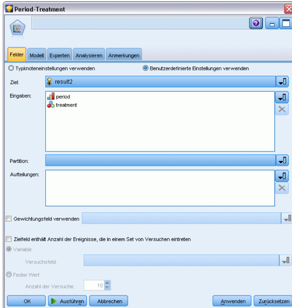
Abbildung 22-23 Auswählen von Felddoptionen
