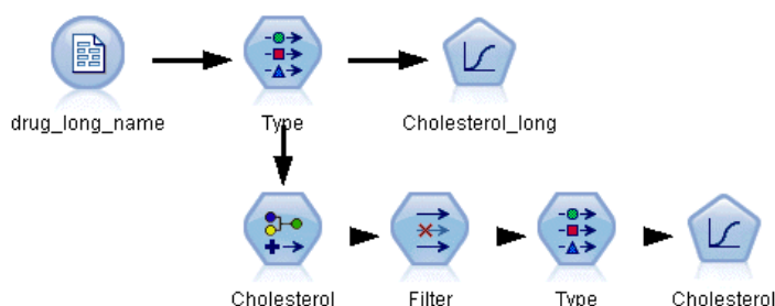
Abbildung 10-1 Beispiel-Stream zur Umkodierung von Zeichenketten für die binomiale logistische Regression
