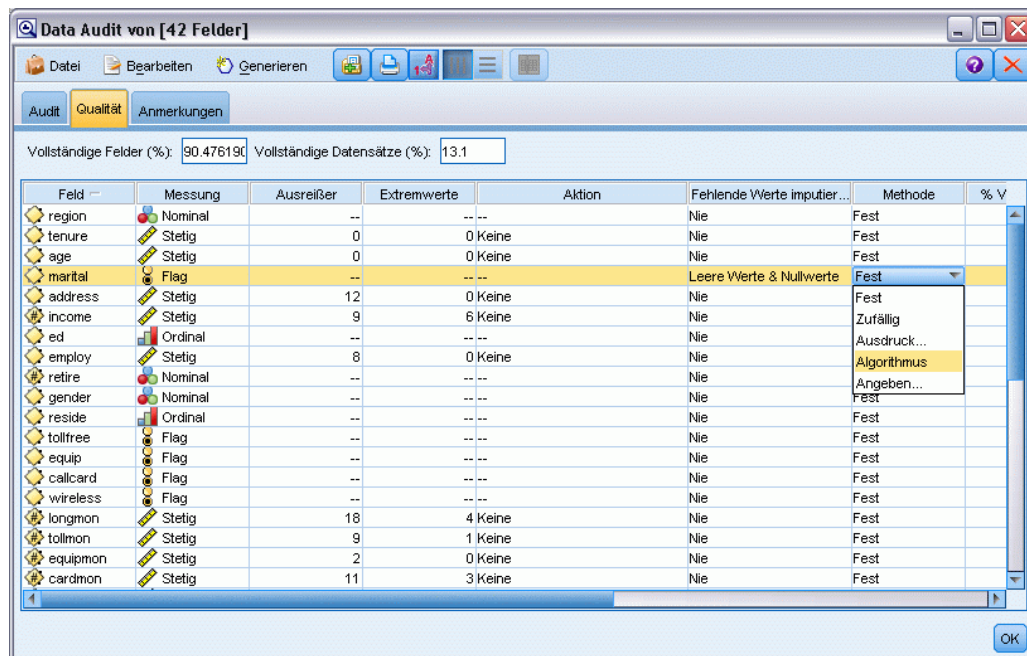
Abbildung 7-11 Auswahl einer Imputationsmethode
