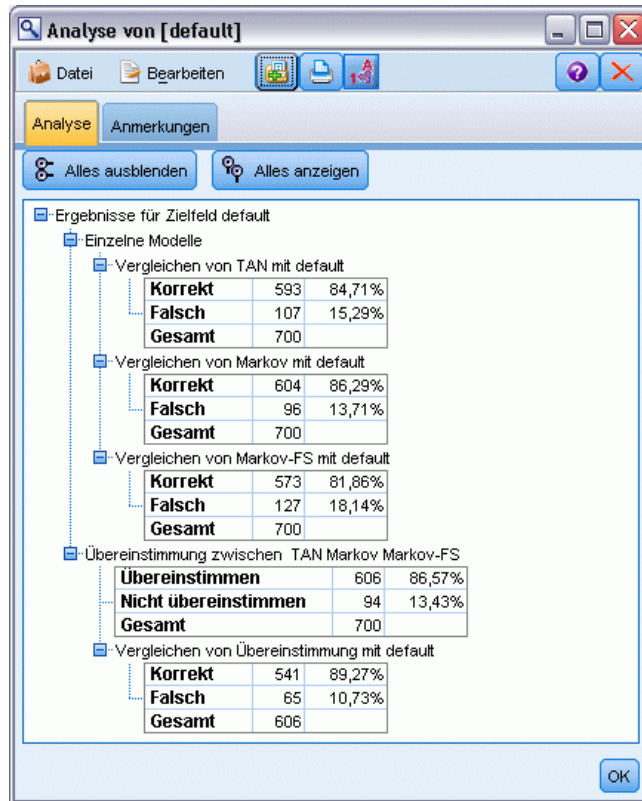
Abbildung 17-11 Analysieren der Modellgenauigkeit
