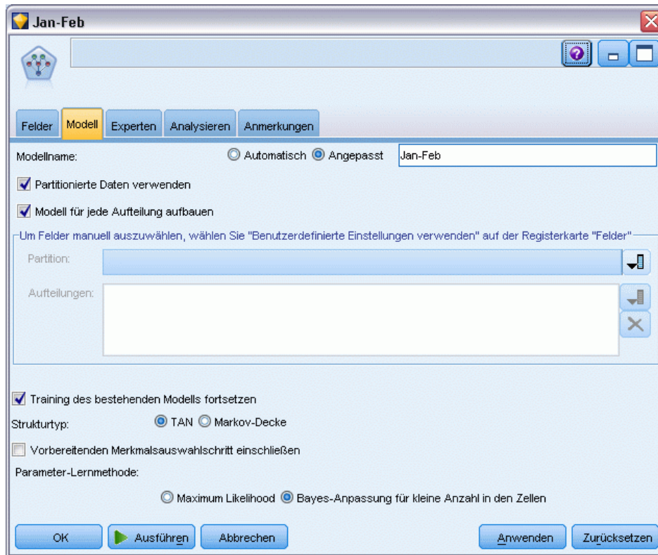
Abbildung 18-6 Erneutes Trainieren des Modells
