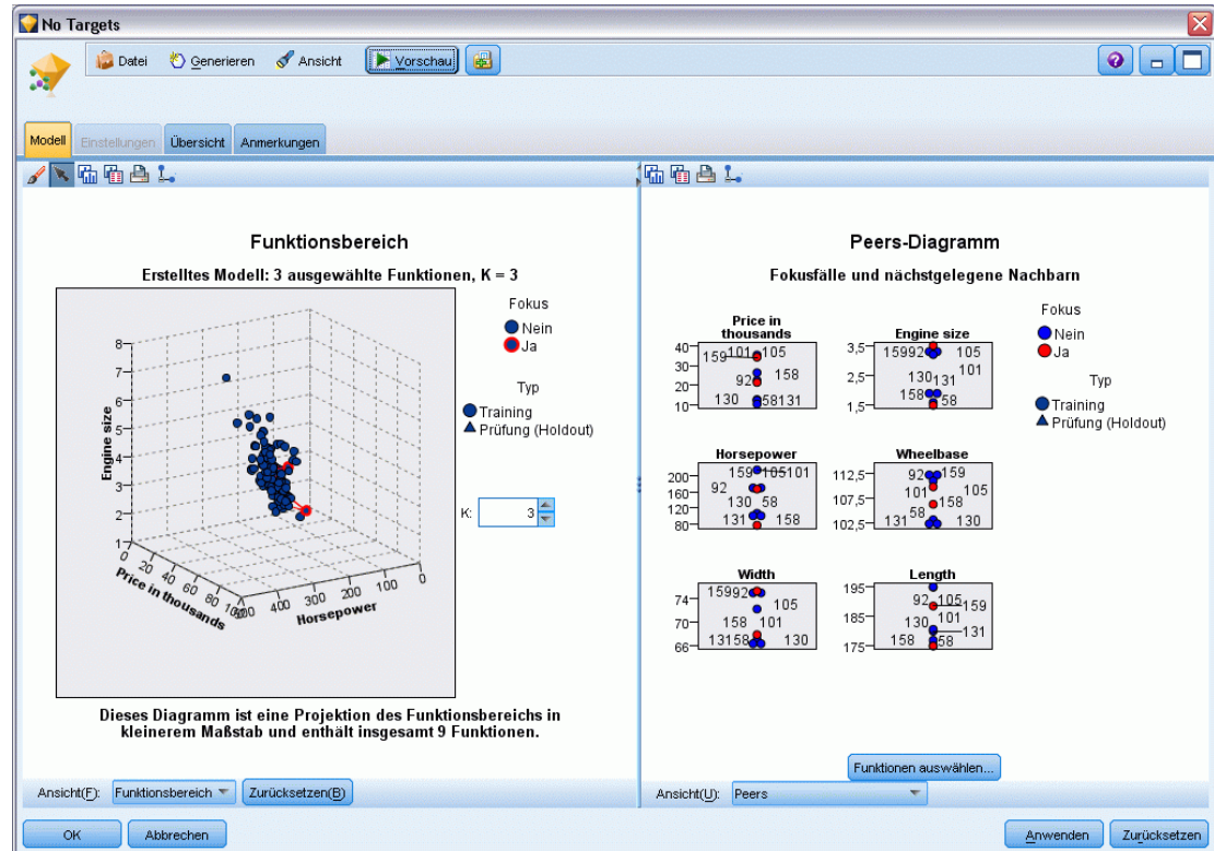
Abbildung 28-7 Das Fenster "Modell-Viewer"
