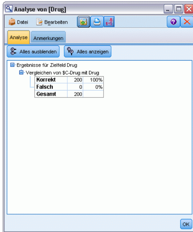
Abbildung 8-25 Analyseknott – Ausgabe
