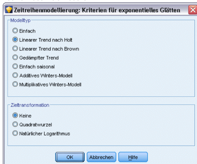
Abbildung 15-9 Auswahl des Holt-Modells
