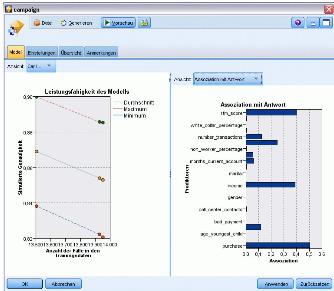
Abbildung 16-12 Aktualisiertes SLRM-Modell-Nugget
