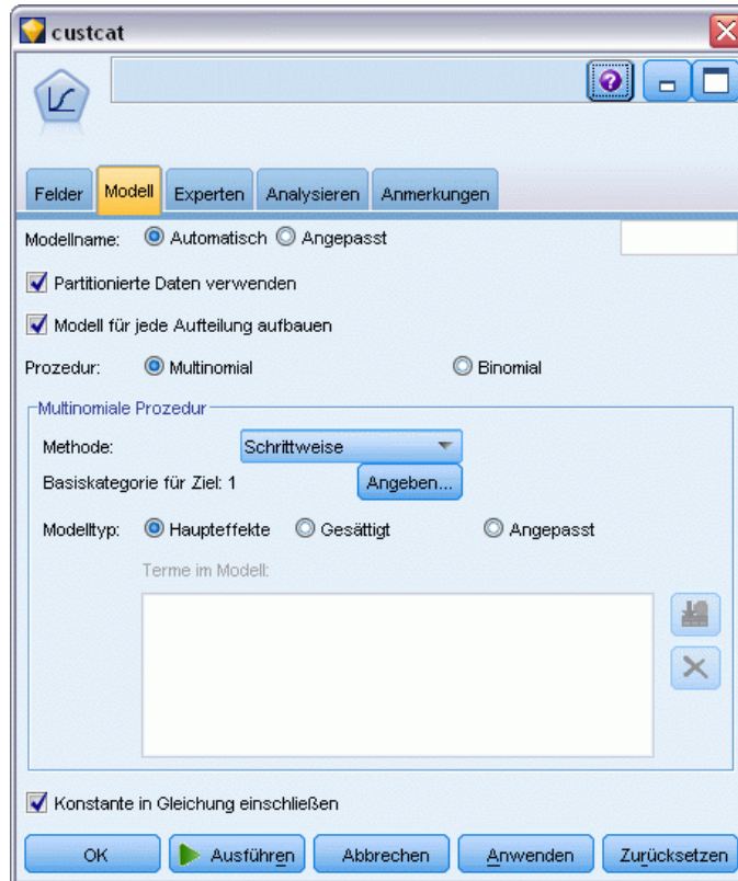
Abbildung 12-5 Auswählen Modelloptionen
