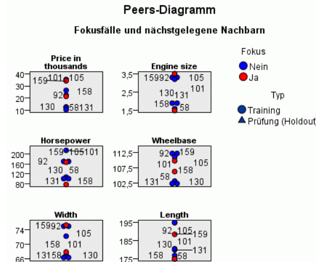
Abbildung 28-9 Peers-Diagramm
