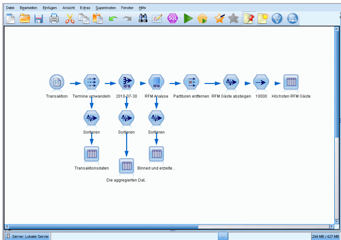
Abbildung 2-12 Maximierter Stream-Zeichenbereich
