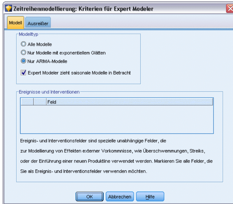
Abbildung 15-15 Ausschließliche Auswahl von ARIMA-Modellen
