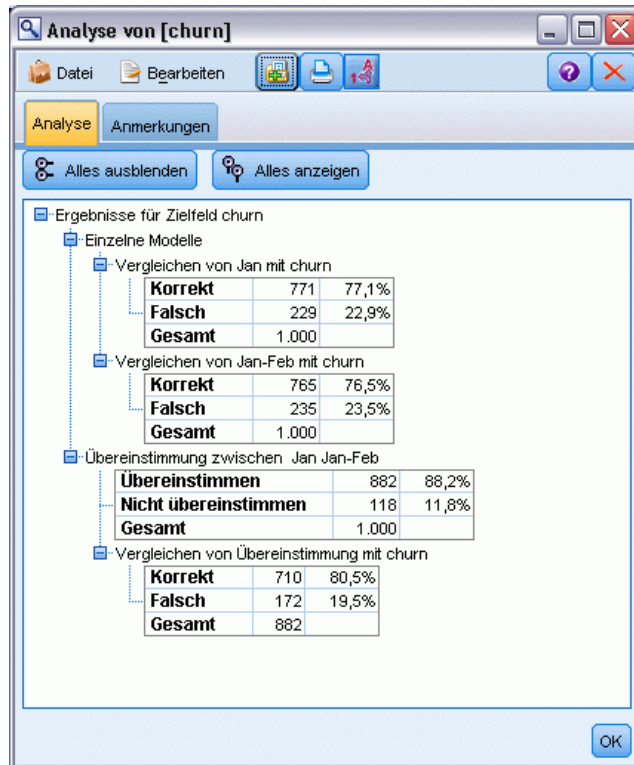
Abbildung 18-13 Analysieren der Modellgenauigkeit
