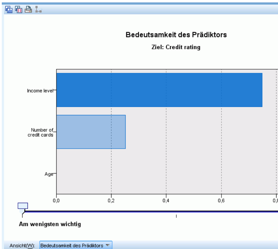
Abbildung 3-10 Bedeutsamkeit der Prädiktoren – Diagramm
