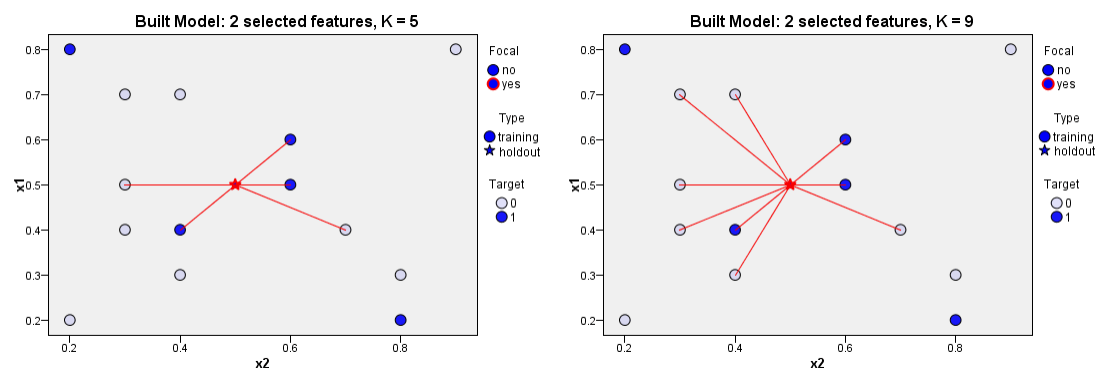
Abbildung 28-1 Auswirkungen der Änderung von "k" bei der Klassifizierung
