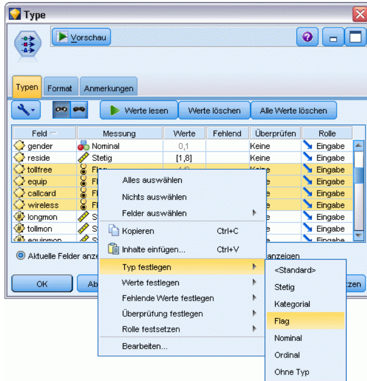
Abbildung 21-3 Festlegen des Messniveaus für mehrere Felder
