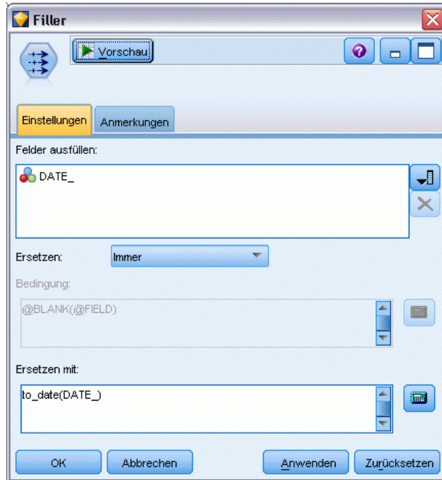
Abbildung 14-8 Einrichten des Datenspeichertyps
