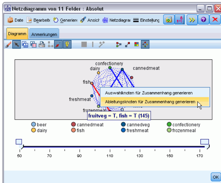
Abbildung 27-6 Ableiten eines Flags für eine Kundengruppe
