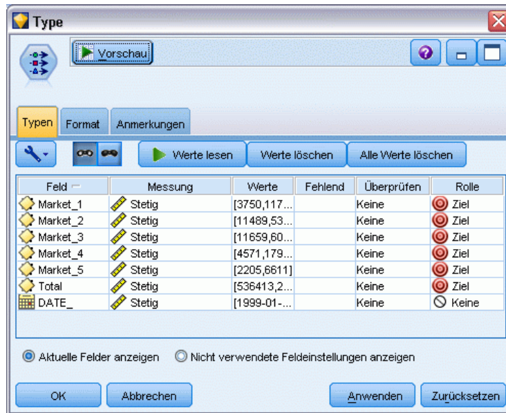
Abbildung 14-10 Festlegen der Rolle für mehrere Felder
