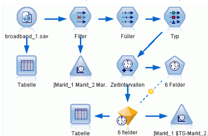
Abbildung 14-14 Beispiel-Stream zur Anzeige der Zeitreihenmodellierung
