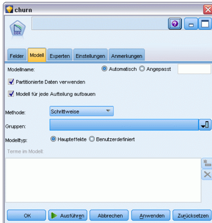
Abbildung 26-5 Auswählen Modelloptionen
