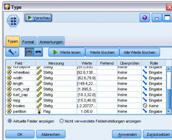
Abbildung 28-4 Typknoteneinstellungen
