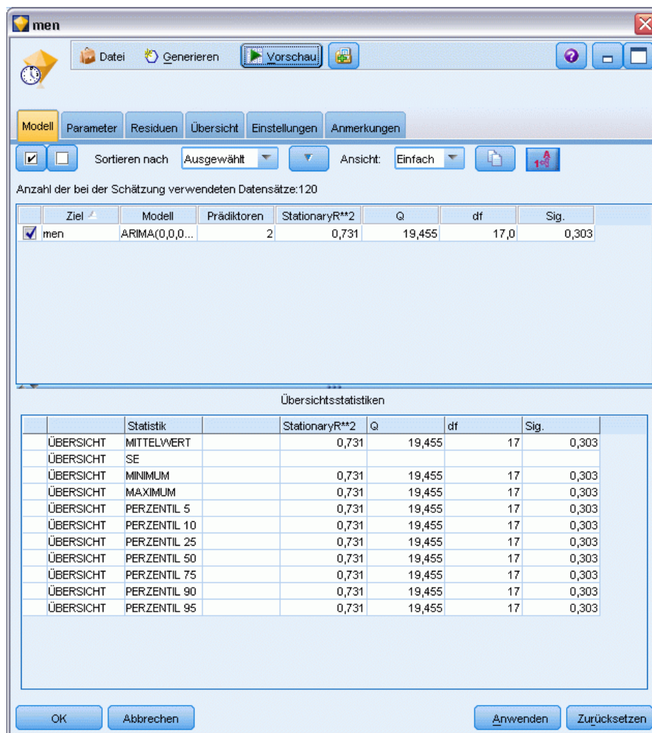
Abbildung 15-16 Der Expert Modeler wählt zwei Prädiktoren aus.
