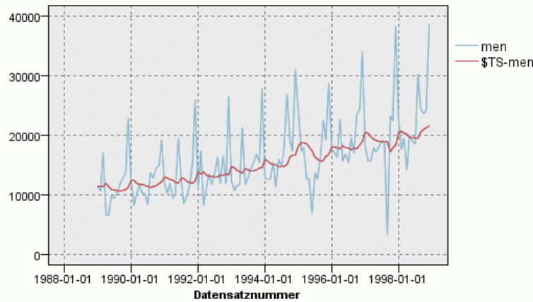
Abbildung 15-8 Einfaches Modell mit exponentiellem Glätten
