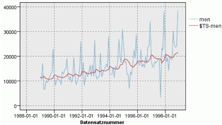
Abbildung 15-17 ARIMA-Modell mit angegebenen Prädiktoren
