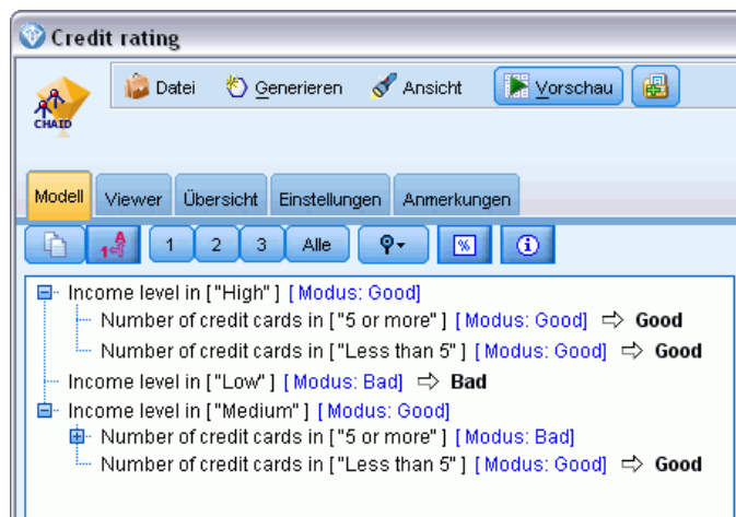
Abbildung 3-9 CHAID-Modell-Nugget, Regelmenge
