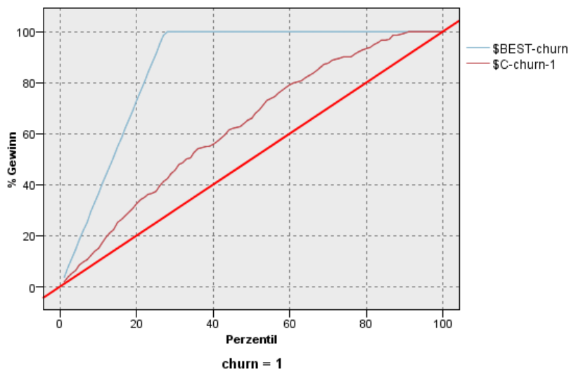
Abbildung 26-18 Gewinndiagramm
