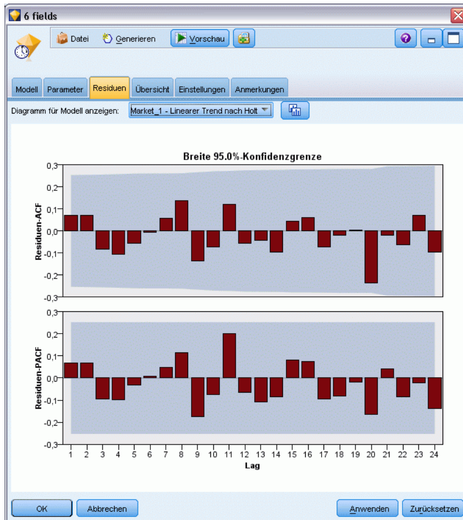
Abbildung 14-17 ACF- und PACF-Werte für die Märkte
