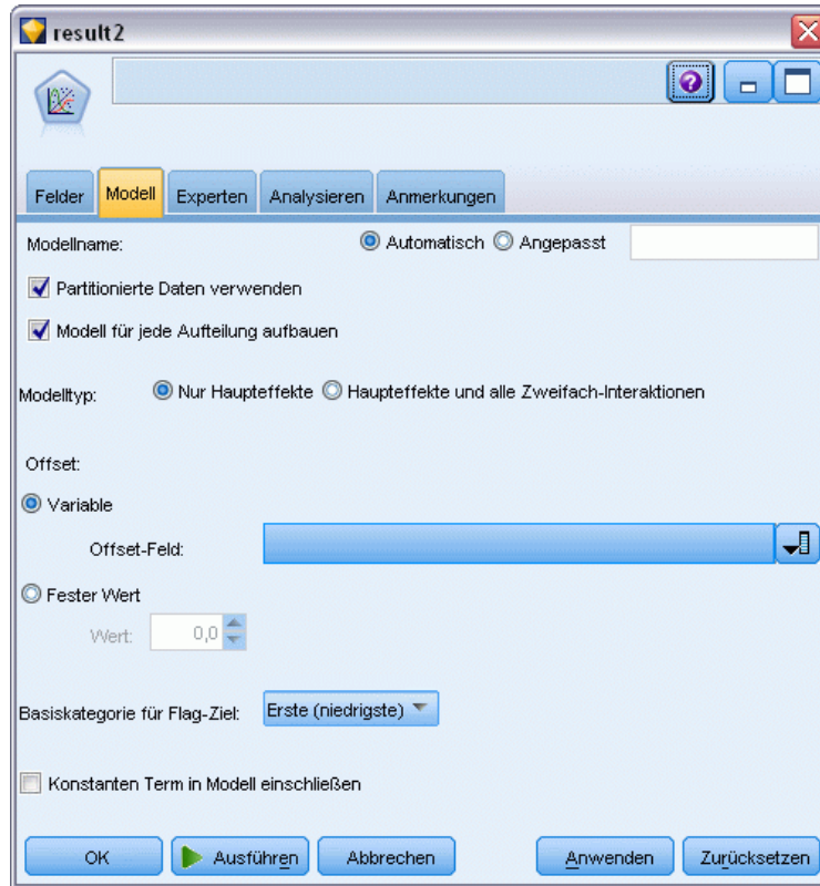
Abbildung 22-20 Auswählen Modelloptionen
