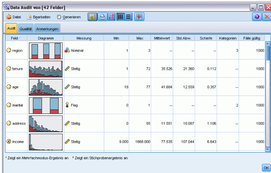
Abbildung 7-6 Data Audit-Browser
