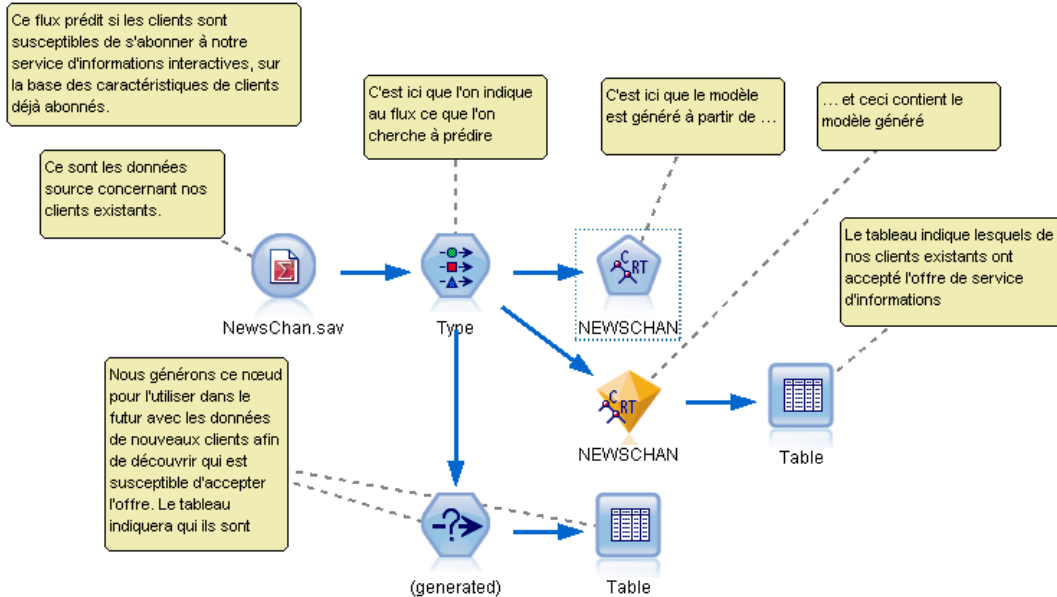
Figure 5-34 Flux avec commentaires ajoutés
