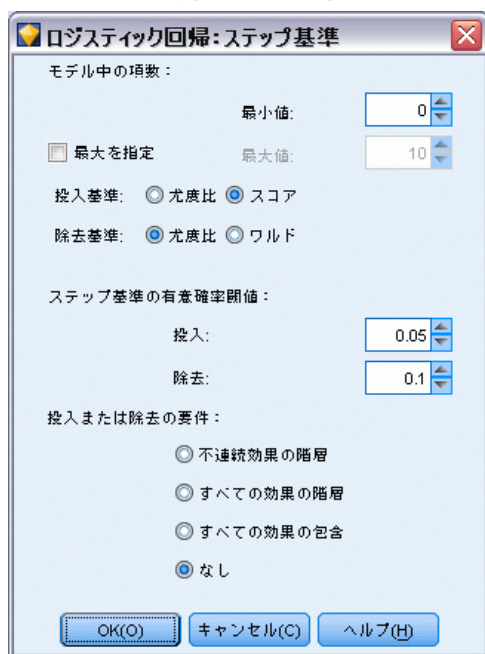
図 10-28 ロジスティック回帰ステップ基準
