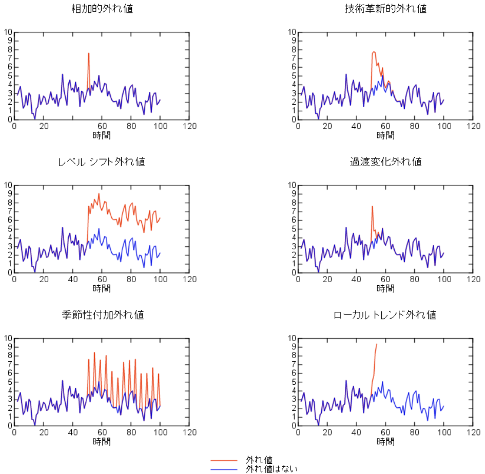
図 13-5 外れ値の種類
