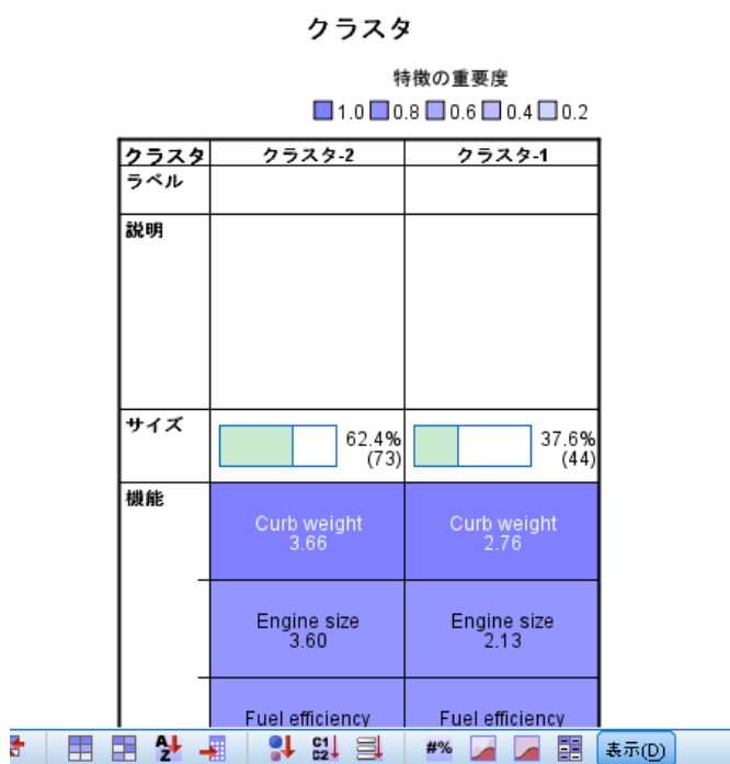
図 11-14 メイン パネルの [クラスタ中心] ビュー
