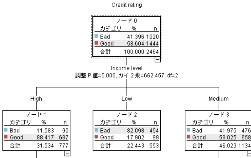
図 2-1 簡単なディビジョン ツリー モデル
