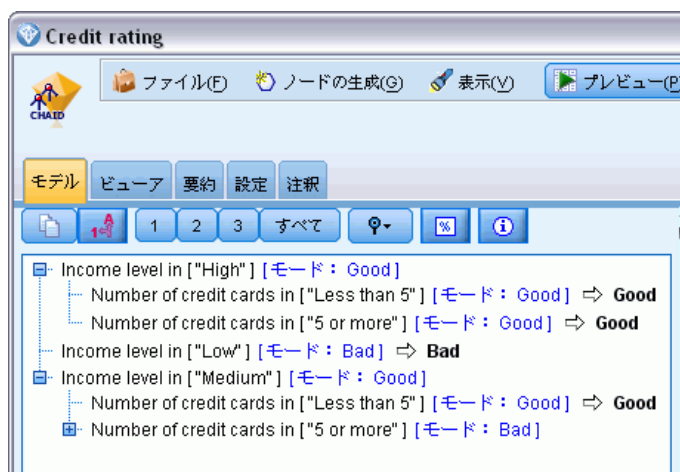
図 2-9 CHAID モデル ナゲット、ルール セット
