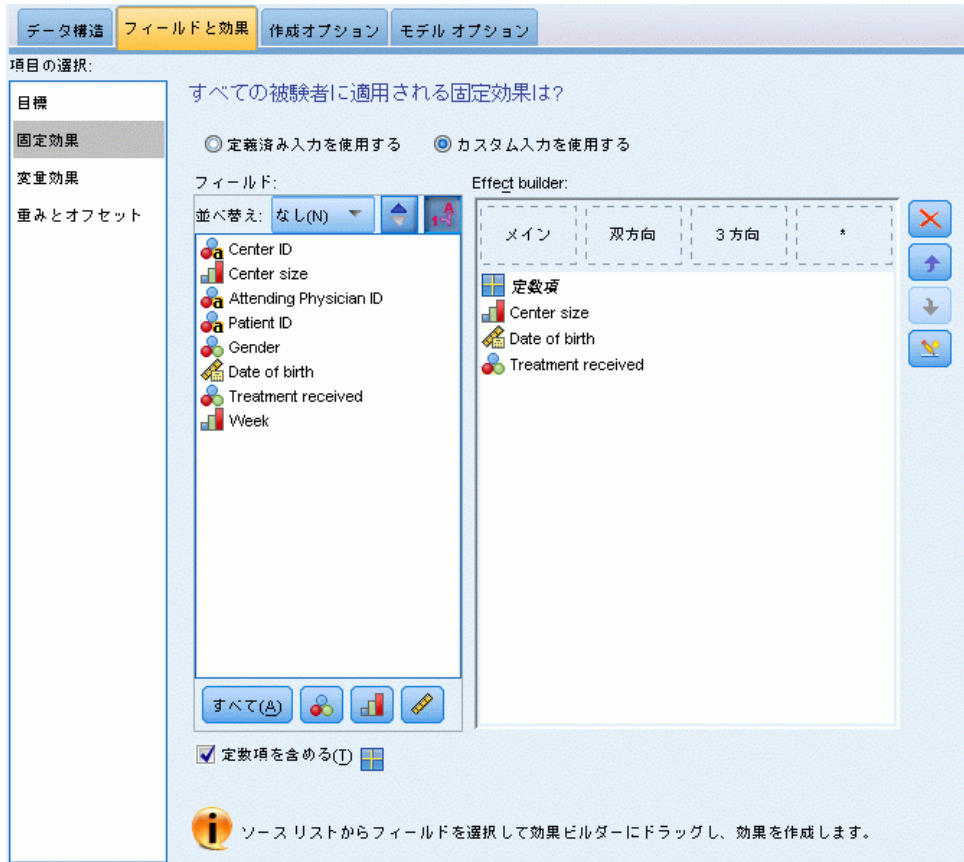
図 10-56 固定効果設定
