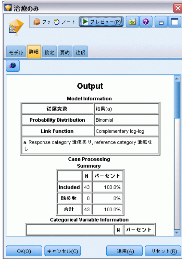
図 10-50 GenLin モデル ナゲット、[詳細] タブ
