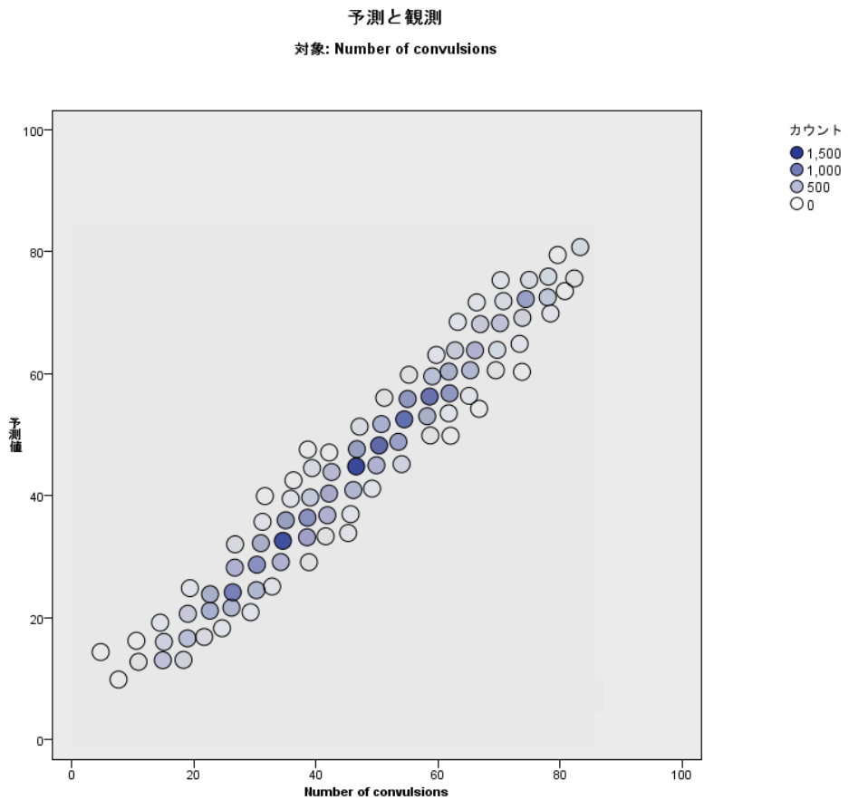
図 10-66 [予測対観測] ビュー
