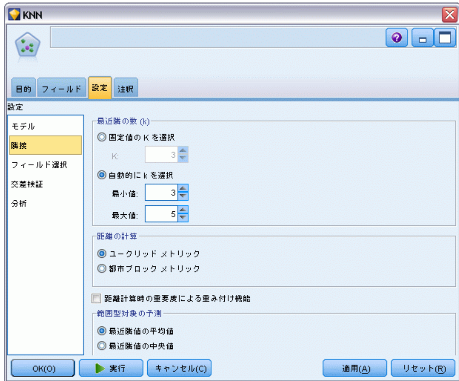
図 16-4 KNN ノードの近隣オプション
