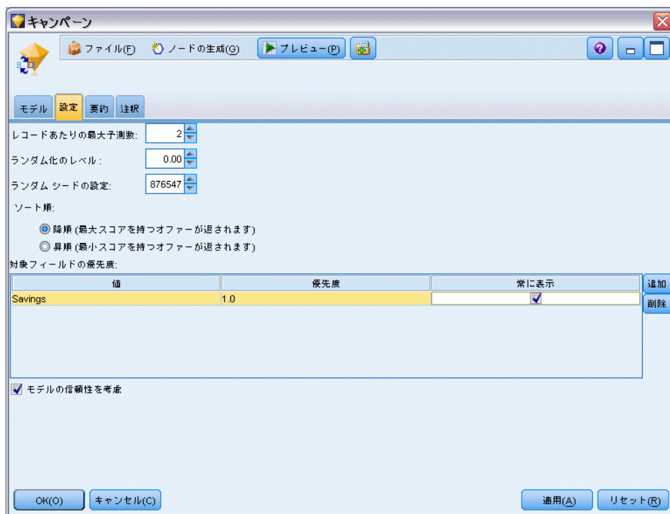
図 14-5 SLRM モデル ナゲットのダイアログ ボックス、[設定] タブ
