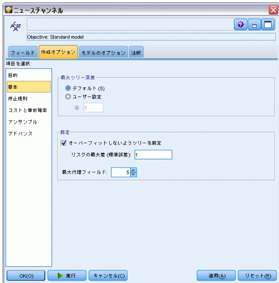
図 6-26 ディシジョン ツリーの基本オプション
