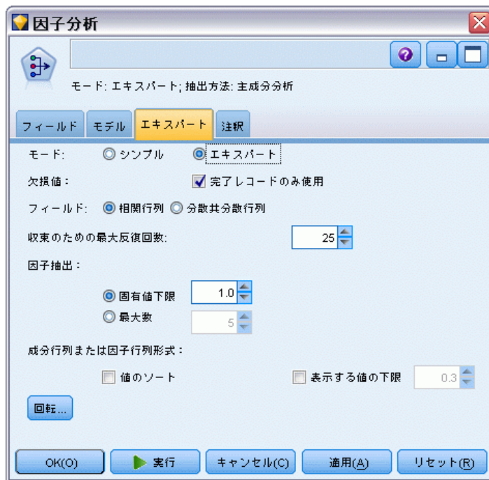
図 10-33 因子分析の [エキスパート] タブ
