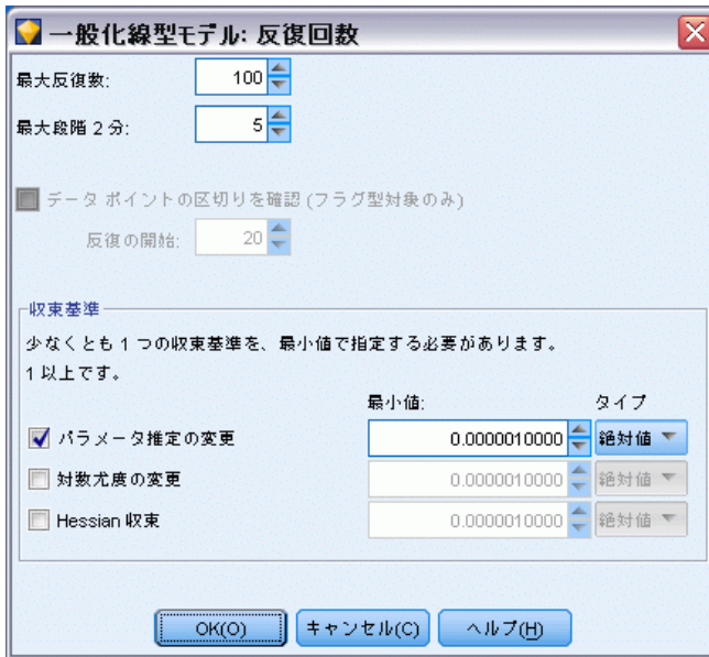
図 10-48 一般化線型モデル作成の反復関連のオプション
