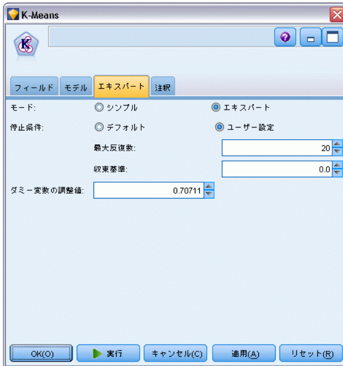
図 11-8 K-Means のエキスパート オプション
