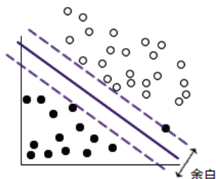
図 15-5 改良されたモデルを含むデータ
