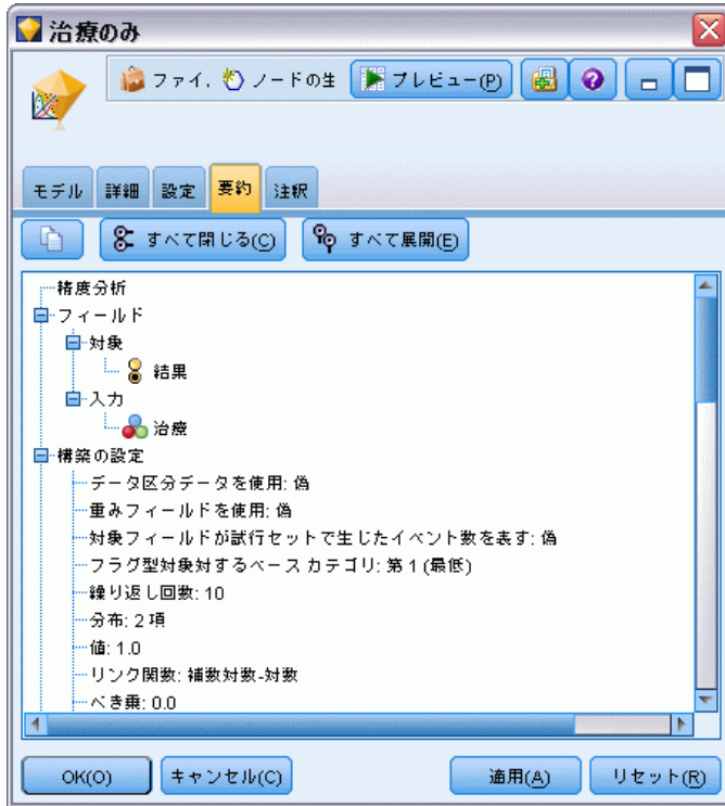
図 10-52 GenLin モデル ナゲット、[要約] タブ
