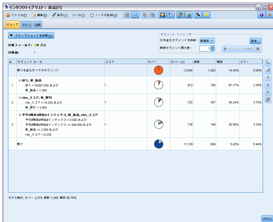
図 9-9 ディシジョン リスト インタラクティブ ビューア
