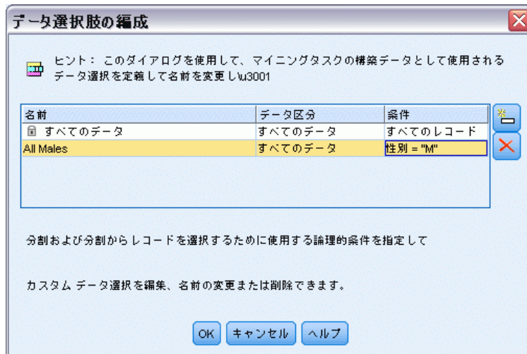
図 9-16 データ条件抽出の編成
