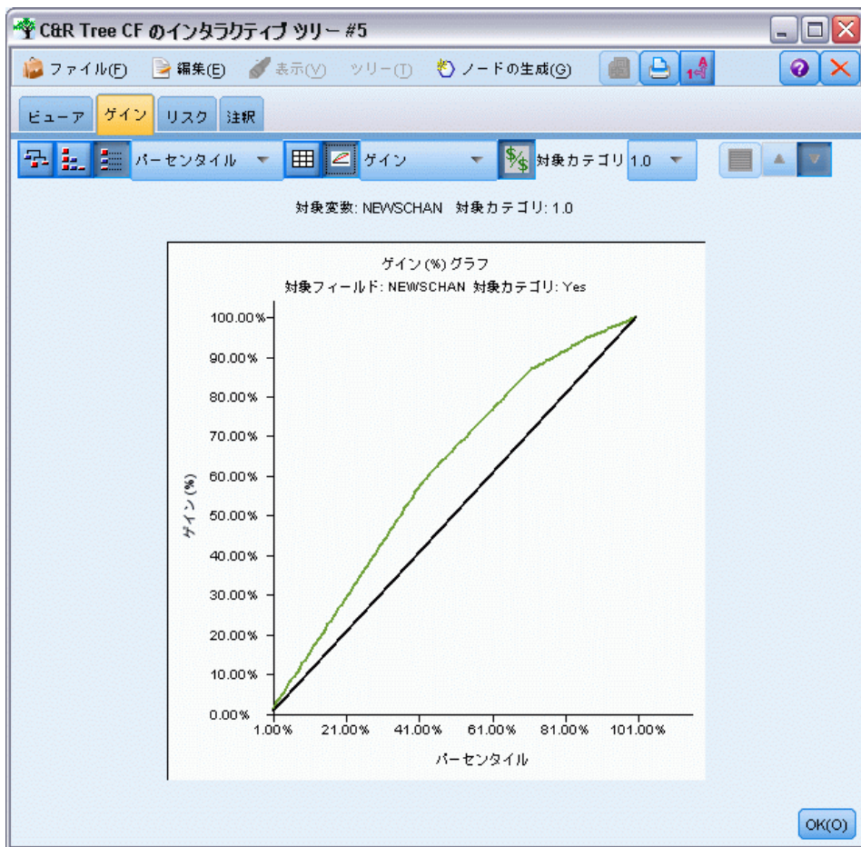
図 6-15 ゲイン グラフ
