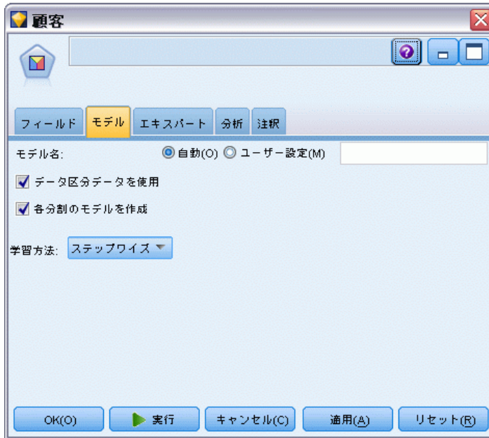
図 10-38 判別分析ノードのダイアログ ボックス、[モデル] タブ
