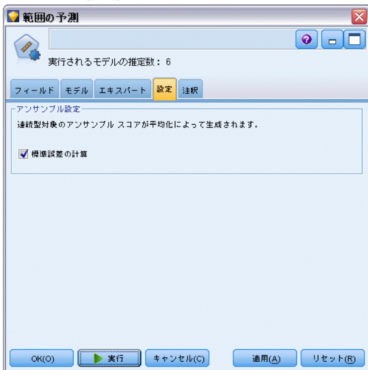
図 5-11 自動数値ノード:[設定] タブ
